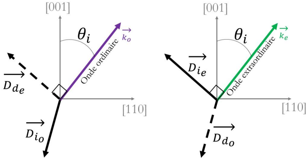
Figure 2.22 : Représentation des vecteurs de polarisation
