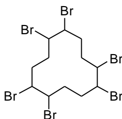
Figure I.5 : Structure chimique du HBCDD
