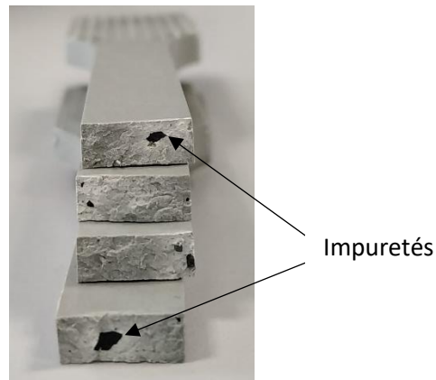
Figure II.21 : Profil de rupture des éprouvettes de traction
