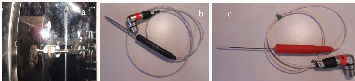
Figure 34 : Images des sondes de températures utilisées pendant les cuissons : a) sonde installée dans la cavité du four mesurant la température de l'environnement de cuisson ; thermosondes utilisées pour mesurer les températures à cœur de la plupart des viandes (à l'exception du blanc de poulet) (b) et des poissons (c).
