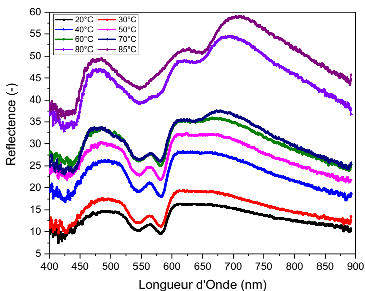
Figure 119 : Spectres collectés dans le visible en mode réflexion sur une tranche de rond parisien cuite au four. La cuisson et la collecte des données ont été réalisées online, en positionnant la fibre à l'intérieur du four. La température de l'échantillon a été suivie par un thermocouple positionné à l'intérieur de la cellule échantillon dans la tranche.
