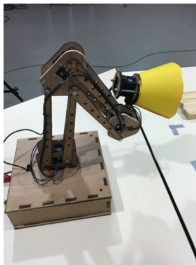
Figure 4 : La lampe robotisée Psyphine
