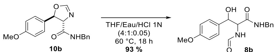
Schéma 110 : Essai de synthèse du diamide- \beta -hydroxylé par ouverture du noyau oxazoline par traitement aqueux
