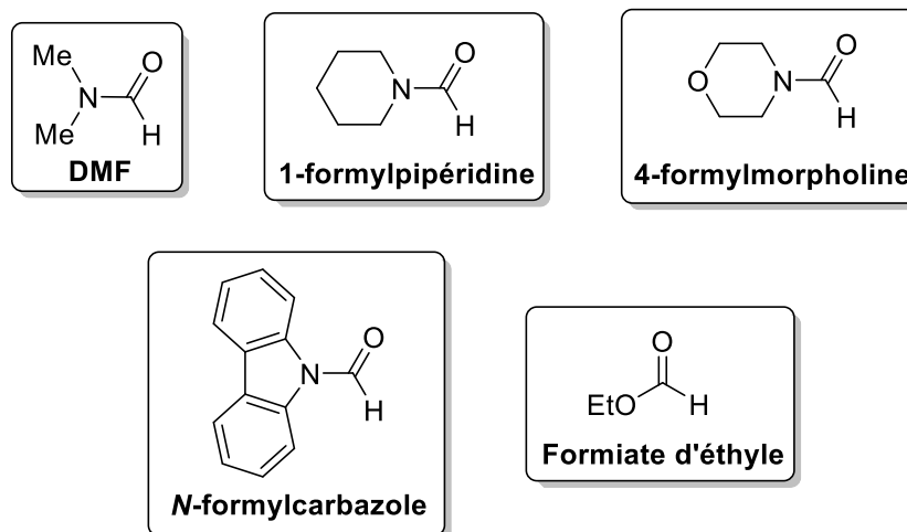
Schéma 74 : Essais de formylation par addition du carbanion sur un agent de formylation
