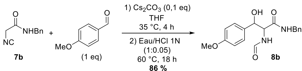
Schéma 111 : Essai de réaction « One-Pot » pour la synthèse du diamide- \beta -hydroxylé à partir d'isocynoacétamide
