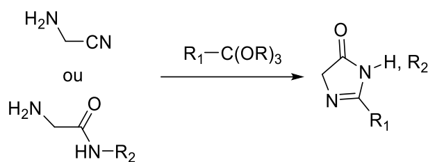
Schéma 11 : Condensation d'ortho-esters sur des dérivés de glycines
