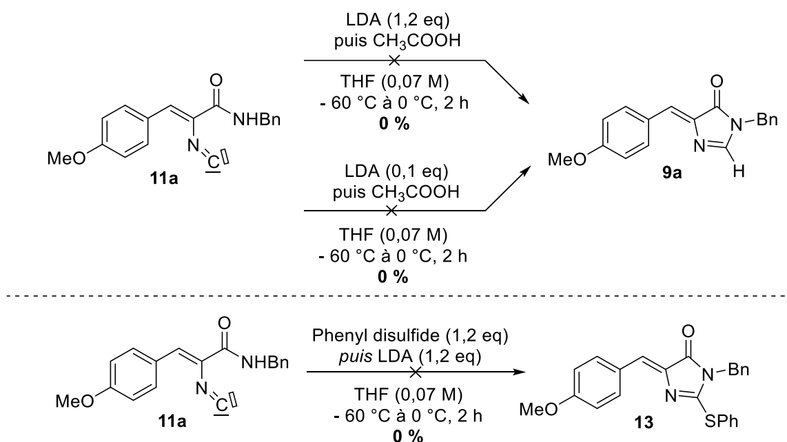
Schéma 117 : Différentes tentatives d'application de la méthodologie de cyclisation-fonctionnalisation sur le motif arylidène-isocynoacétamide
