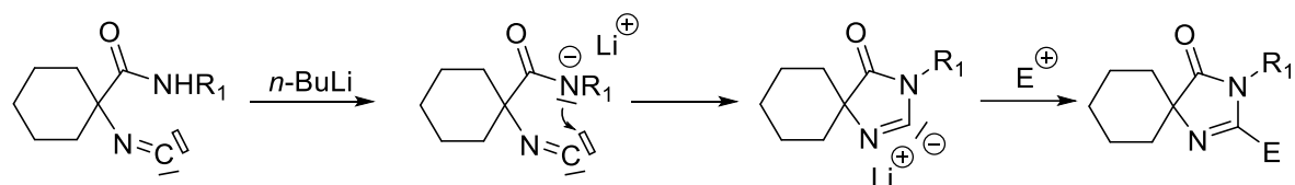
Schéma 58 : Synthèse de spiro-imidazolones proposée par Marcaccini
