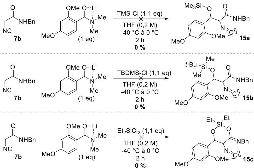
Schéma 145 : Essais de piégeage de l'intermédiaire commun via divers agents de silylation
