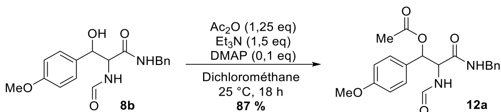
Schéma 112 : Réaction d'acétylation de l'alcool du diamide-β-hydroxylé à partir d'anhydride acétique
