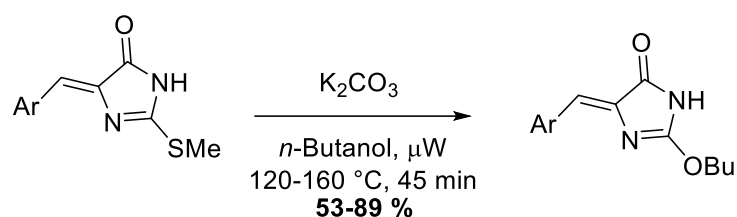
Schéma 22 : Amination et étherification à partir d'imidazolones activées par un groupe partant SME en position C2
