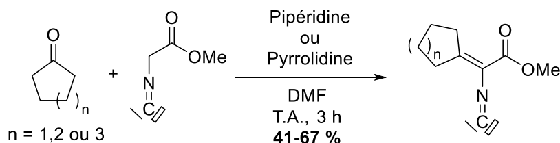
Schéma 86 : Synthèses d'alkylidènes-isocianoacétates proposées par Nunami via élimination de type Knoevenagel
