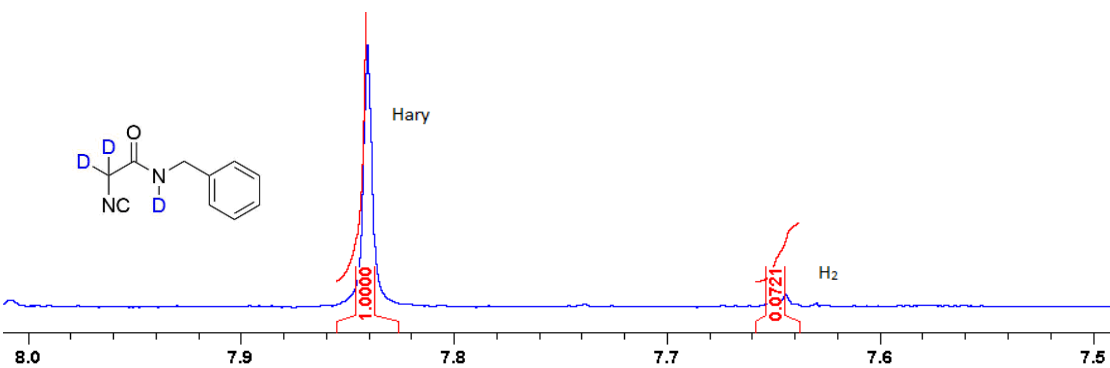
Figure 26 : Essais de deutériation avec comparaison RMN ^1\text{H} des hydrogènes positionnés en C2(H 2 ) et C Arylidène (H ary ) de l'imidazolone à partir d'isonitriles-amides diversement marqués
