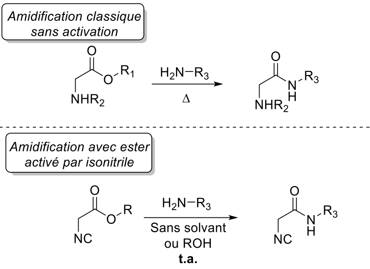
Schéma 88 : Réaction de substitution par une amine primaire pour aboutir aux isocynoacétamides non disubstitués
