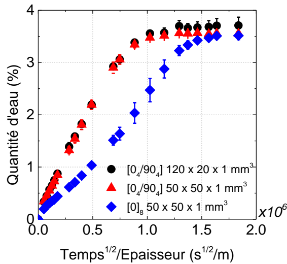
Comparaison des cinétiques de diffusion d'eau dans des échantillons asymétriques et unidirectionnels
