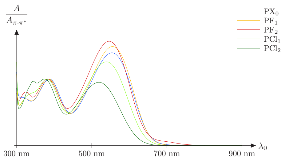
Fig. 29 – Spectres d'absorption des terpolymères de la série benzothiadiazole/thiophène/thiénothiophène en solution à 95\text{ °C}
