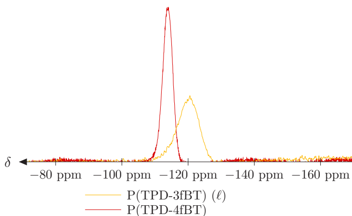
Fig. 33 – Spectres RMN-MAS ^{19}\text{F} des copolymères thiényrroledione/bithiophène fluorés
