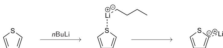
Fig. 4 – Lithiation du thiophène par le n -butyllithium
