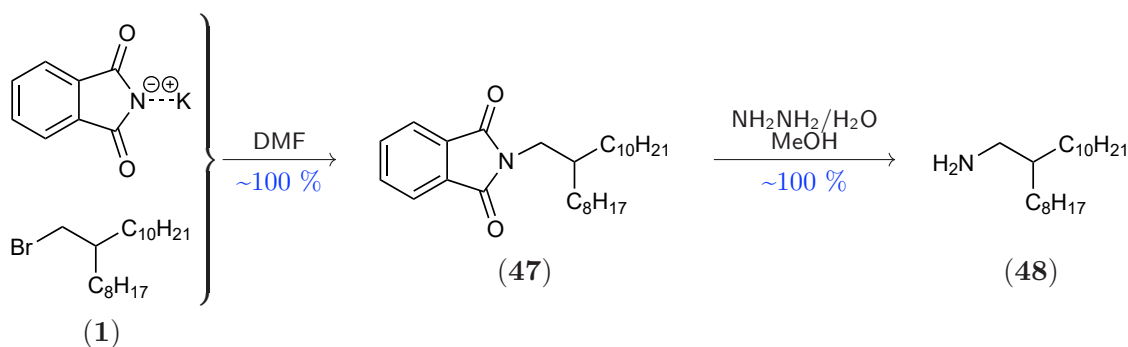
Fig. 1 – Synthèse du 1-amino-2-octyldodécane
