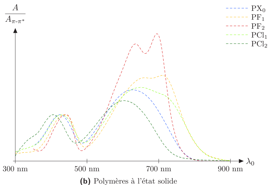
Fig. 26 – Spectres d'absorption des terpolymères benzothiadiazole/thiophène/thiénythiophène à température ambiante
