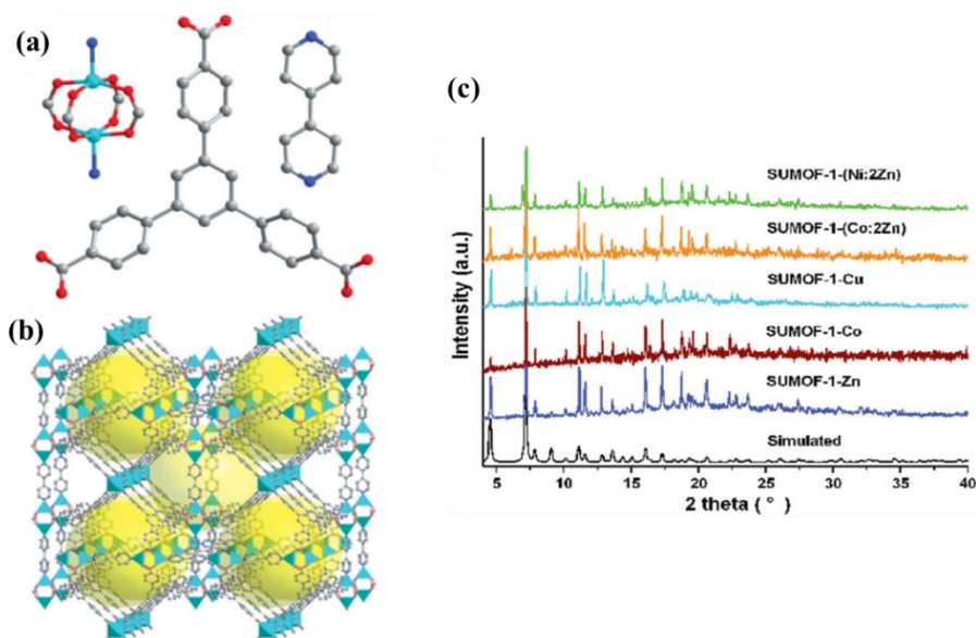
Figure 21 : (a) représentation du cluster métallique de type « paddle-wheel », du ligand BTB et du ligand Bpy (b) et de la totalité du réseau [Zn_6(BTB)_4(Bpy)_3]_{x}[(Sol)_x] ou SUMOF-1 (les polyèdres de coordination sont en turquoise et les ligands en gris), (c) comparaison du diffractogramme pour le réseau de départ SUMOF-1-Zn aux diffractogrammes obtenus pour les composés issus des réactions d'échange avec les ions Co^{2+} (SUMOF-1-Co), Cu^{2+} (SUMOF-1-Cu) et aux diffractogrammes issus de la réversibilité des réactions d'échange SUMOF-1- Co:2Zn et SUMOF-1-Ni:2Zn. D'après référence 92 .
