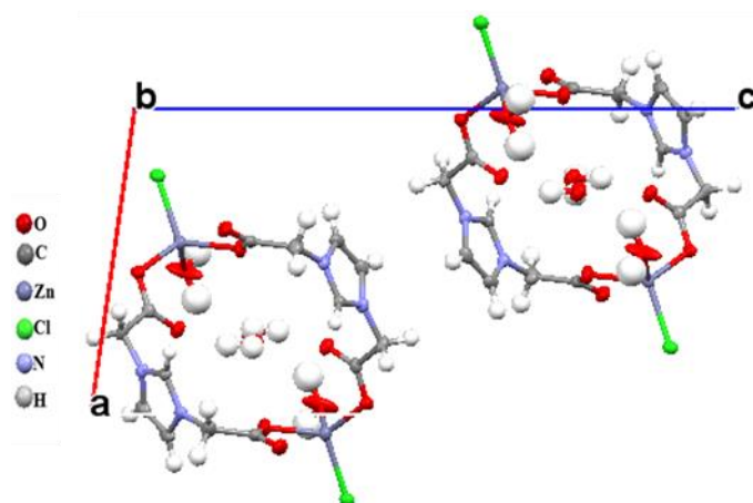
Figure 2 : représentation de la structure du réseau [\text{Zn}(\text{L1})(\text{Cl})(\text{H}_2\text{O})].(\text{H}_2\text{O}) .
