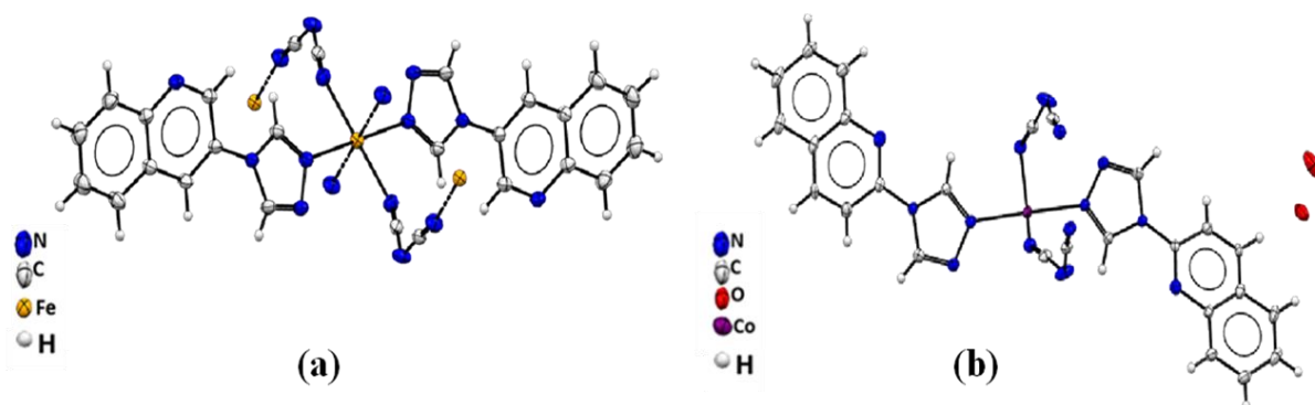
Figure 43 : représentation Ortep des deux composés (a) [Fe(Quino-Triaz) 2 (dca) 4 ] ( 4 ) et (b) [Co(Quino-Triaz) 2 (dca) 4 ].2 H 2 O ( 5 ).
