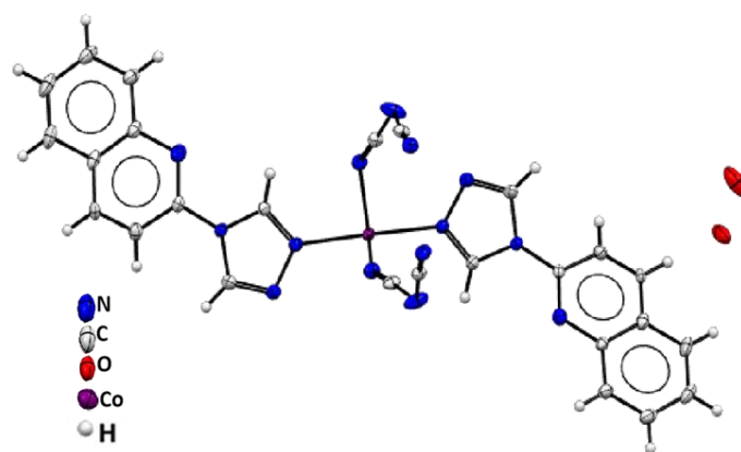
Figure 44 : représentation Ortep de l'unité asymétrique du composé [Co(Quino-Triaz) 2 (dca) 4 ].2 H 2 O ( 5 ).
