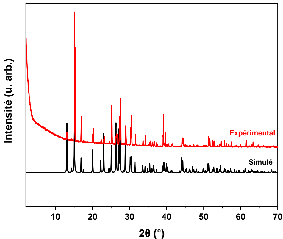
Figure 11 : comparaison du diffractogramme simulé à partir de la structure obtenue sur monocristal (en noir) et du diffractogramme sur poudre pour le composé [BiIm][FeCl 4 ] (en rouge).
