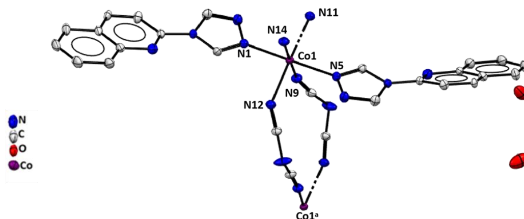
Figure 45 : représentation Ortep de l'environnement autour de l'ion Co 2+ dans le composé [Co(Quino-Triaz) 2 (dca) 4 ].2 H 2 O ( 5 ). Position équivalente : (a) x-1, y, z.
