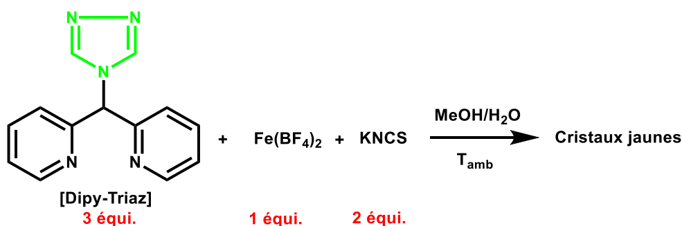
Figure 3 : schéma indiquant les conditions de réaction pour la formation du composé [Fe_2(\text{Dipy-Triaz})_3(\text{NCS})_4(\text{H}_2\text{O})_2] \cdot 3,94 \text{ H}_2\text{O} ( 1 ).
