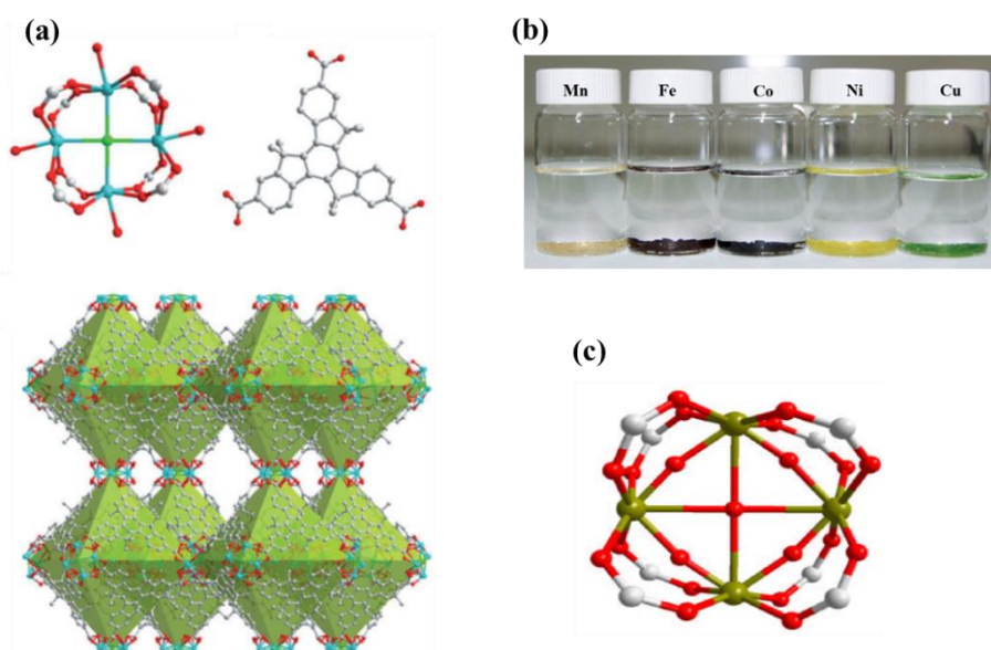
Figure 20 : (a) représentation de l'unité métallique constituant le réseau POST-65-Mn, du ligand hmt et de la structure du réseau POST-65, (b) photographie indiquant les changements de couleur liés à l'insertion des ions Mn^{2+}, Fe^{3+}, Co^{2+}, Ni^{2+} et Cu^{2+} dans le réseau préformé POST-65 et (c) représentation de l'unité métallique présente dans le réseau après insertion des ions Fe^{3+} . D'après référence 96 .
