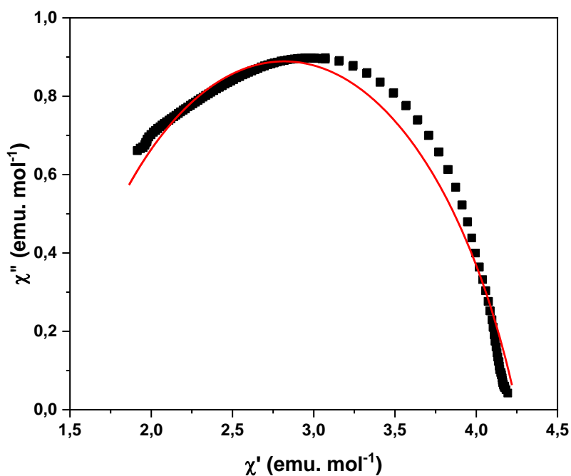
Figure 29 : courbe Cole-Cole pour le composé [\text{BiIm}]_3[\text{DyCl}_6] à 1,8 K sous un champ de statique de 500 Oe, avec un champ ac de 2 Oe pour 10 \text{ Hz} < \nu < 120 \text{ Hz} et 10 Oe pour 120 \text{ Hz} < \nu < 1000 \text{ Hz} . La ligne représente le meilleur ajustement en considérant un modèle de Debye généralisé.
