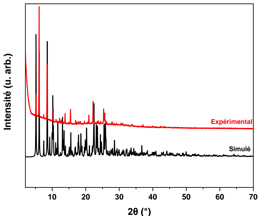
Figure 17 : comparaison du diffractogramme simulé à partir de la structure obtenue sur monocristal (en noir) et du diffractogramme expérimental sur poudre du composé [\text{Co}_2(\text{Dipy-Triaz})_6(\text{NCS})_4(\text{H}_2\text{O})_2] \cdot 2,4 \text{ H}_2\text{O} ( 2 ) (en rouge).
