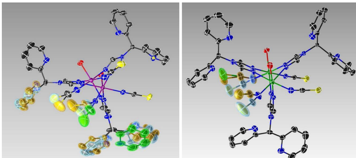
Figure 14 : représentation Ortep des deux composés [\text{Co}_2(\text{Dipy-Triaz})_3(\text{NCS})_4(\text{H}_2\text{O})_2].2,4 \text{ H}_2\text{O} ( 2 ) (à droite) et [\text{Fe}_2(\text{Dipy-Triaz})_3(\text{NCS})_4(\text{H}_2\text{O})_2].3,94 \text{ H}_2\text{O} ( 1 ) (à gauche) soulignant le désordre sur le ligand thiocyanate et/ou cycles pyridiniques.
