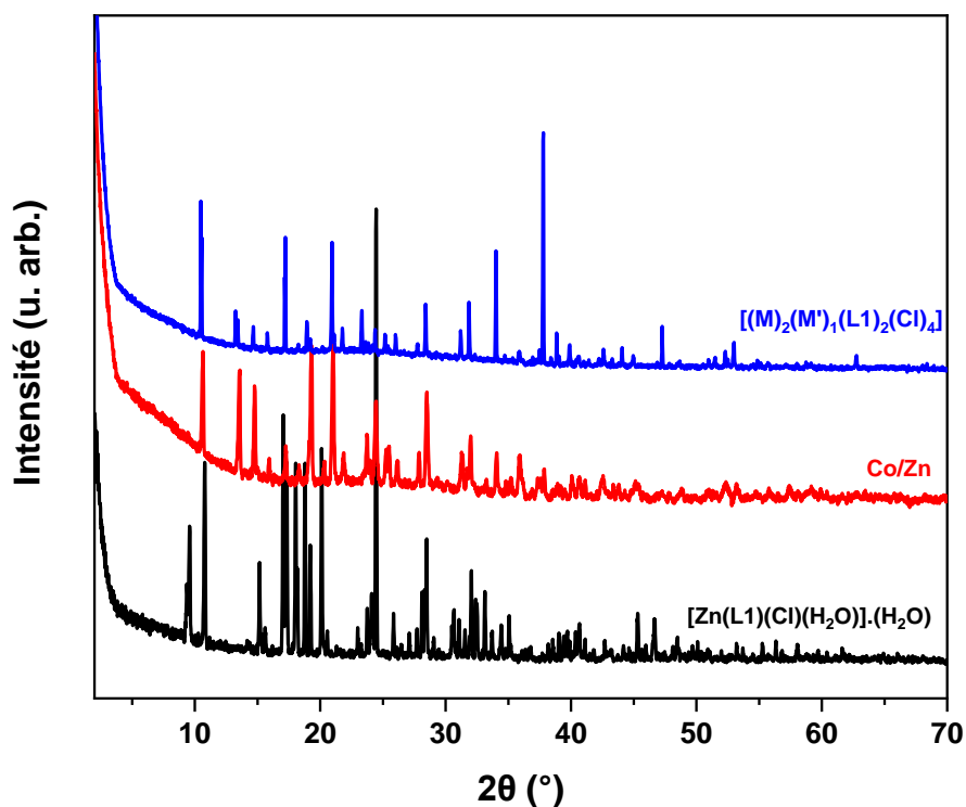
Figure 13 : comparaison des diffractogrammes du réseau de départ [Zn(L1)(Cl)(H_2O)].(H_2O) (en noir), du composé issu de l'échange métallique Co/Zn (en rouge) et du composé hétérométallique obtenu par voie solvothermale et noté [(M)_2(M')_1(L1)_2(Cl)_4(H_2O)_4] (en bleu).
