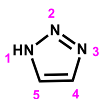
Tautomère 1H
