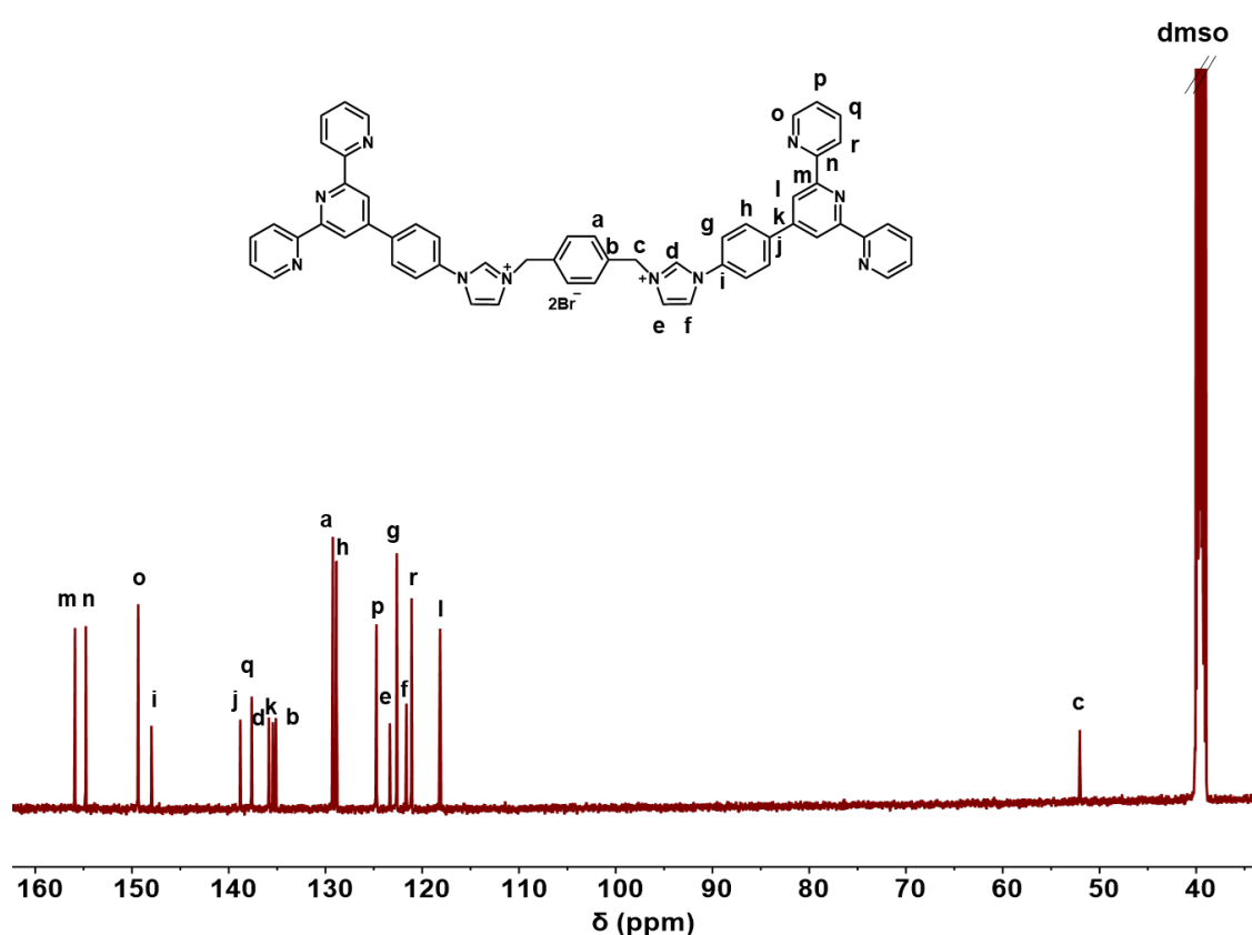
Figure 19 : Spectre RMN ^{13}\text{C} du sel d'imidazolium [(\text{CH}_2)_2\text{Ph}(\text{ImPhTerpy})_2][\text{Br}]_2 réalisé dans le DMSO- \text{d}_6 sur un spectromètre 500 MHz.
