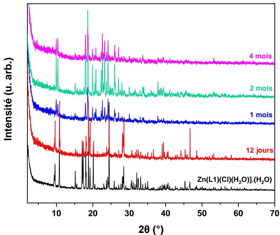
Figure 8 : comparaison du diffractogramme du réseau de départ [\text{Zn}(\text{L1})(\text{Cl})(\text{H}_2\text{O})] \cdot (\text{H}_2\text{O}) (en noir) et des diffractogrammes expérimentaux obtenus pour les composés après imprégnation pendant 12 jours (en rouge), 1 mois (en bleu), 2 mois (en vert) et 4 mois (en rose).
