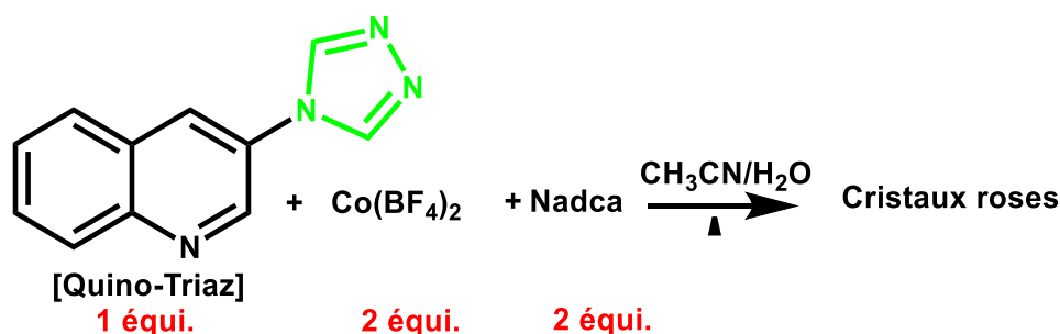
Figure 42 : schéma indiquant les conditions de réaction pour la formation du composé [Co(Quino-Triaz) 2 (dca) 4 ].2 H 2 O ( 5 ).
