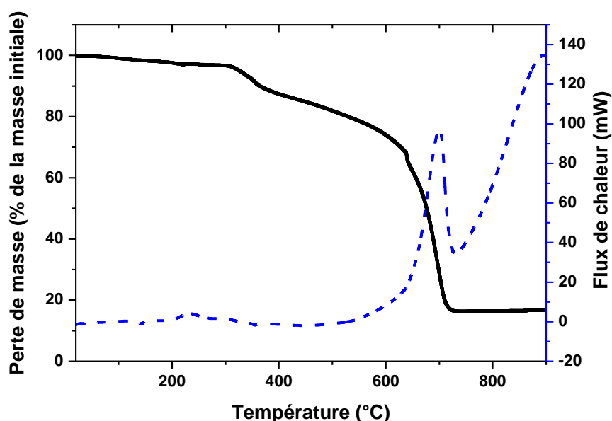
Figure 5 : courbe ATG (en noir) et ATD (en pointillés bleus) du composé [\text{BiIm}]_2[\text{CoCl}_4] .
