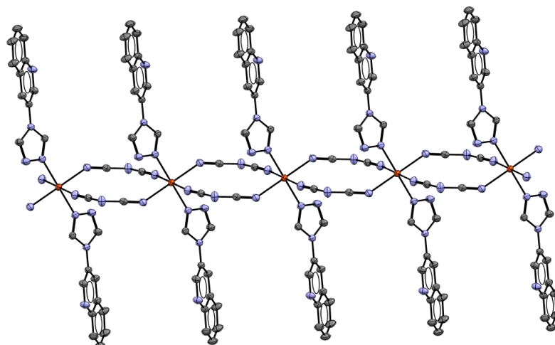
Figure 36 : représentation des chaînes générées le long de l'axe b par la coordination des ions \text{Fe}^{2+} aux ligands \text{dca}^- .
