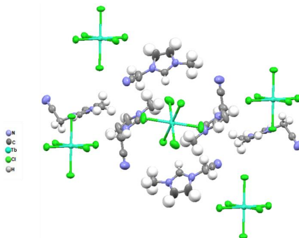
Figure 2 : représentation en mode ellipsoïde de la structure du composé [MonoIm] 3 [TbCl 6 ].
