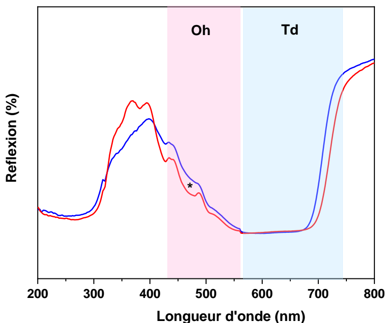
Figure 16 : spectres UV-Visible du composé issu de l'échange Co/Zn (en bleu) et du composé hétérométallique obtenu par voie solvothermale (en rouge) dans la gamme comprise entre 200 nm et 800 nm. Le rectangle en rose indique la zone de prédominance de la transition électronique {}^4T_{1g}(F) \rightarrow {}^4T_{1g}(P) d'ions Co^{2+} en géométrie octaédrique et celui en bleu de la transition {}^4A_2(F) \rightarrow {}^4T_1(F) d'ions Co^{2+} en géométrie tétraédrique.
