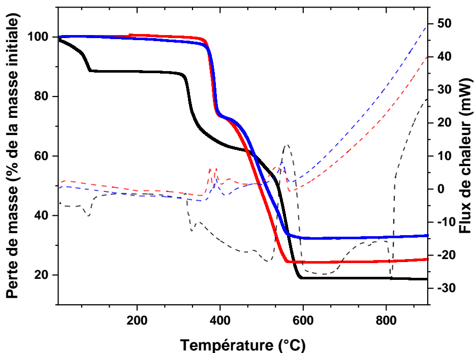
Figure 18 : courbes ATG (trait plein) et ATD (trait en pointillés) du composé issu de l'échange Co/Zn (en rouge), du réseau de départ [Zn(L1)(Cl)(H_2O)].(H_2O) (en noir) et du composé hétérométallique obtenu par voie solvothermale (en bleu).
