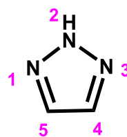
Tautomère 2H
