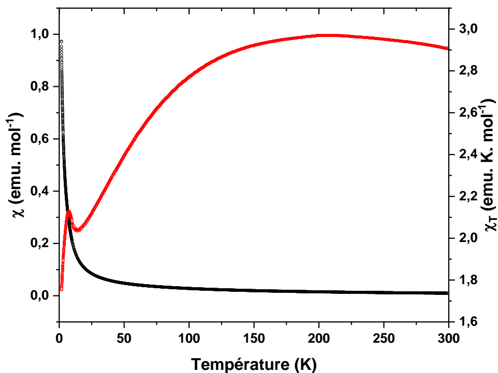
Figure 49 : représentation de la courbe de susceptibilité magnétique \chi (en noir) et du produit \chi T (en rouge) en fonction de la température pour le composé [\text{Co}(\text{Quino-triaz})_2(\text{dca})_4] \cdot 2 \text{H}_2\text{O} ( 5 ).
