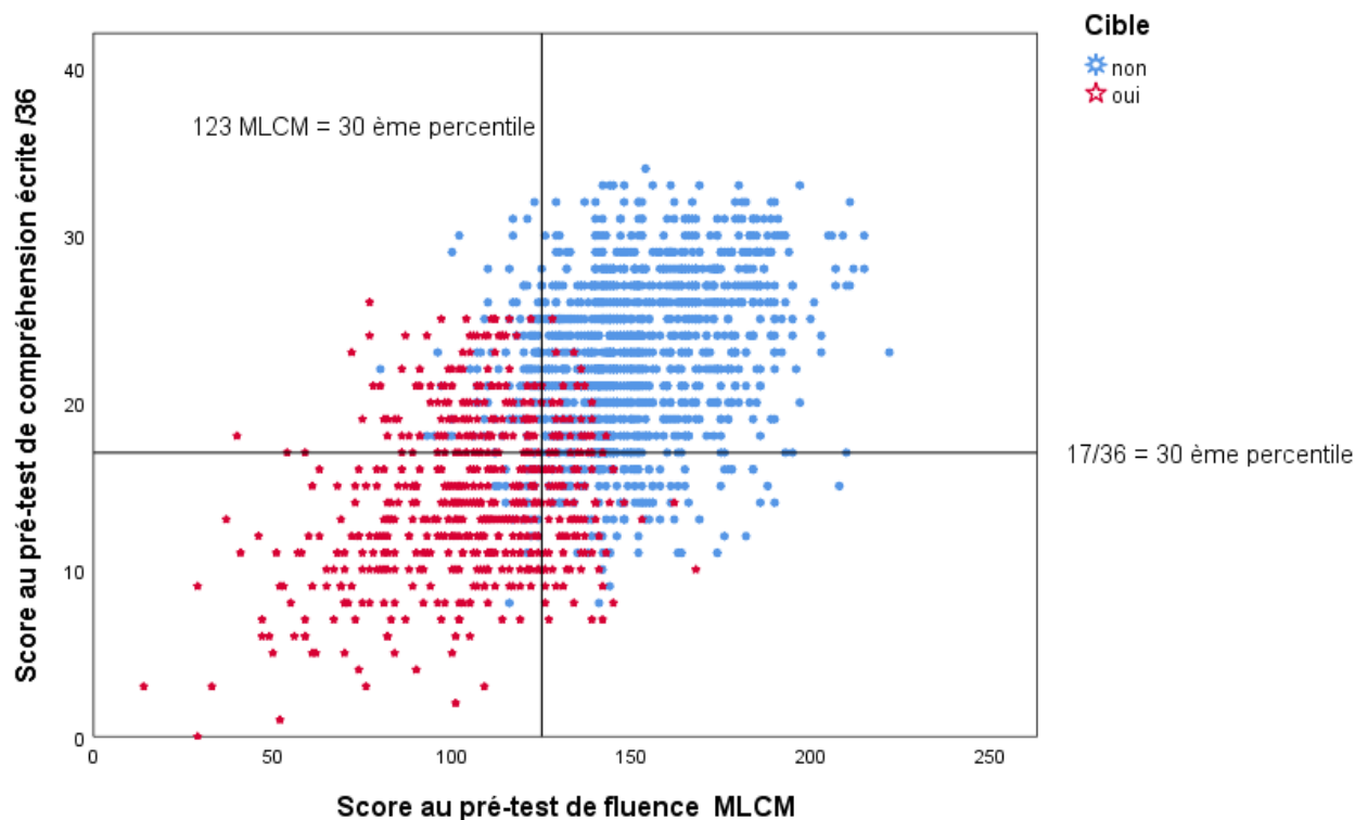
Figure 9 : Dispersion croisée des scores en fluence et en compréhension écrite
