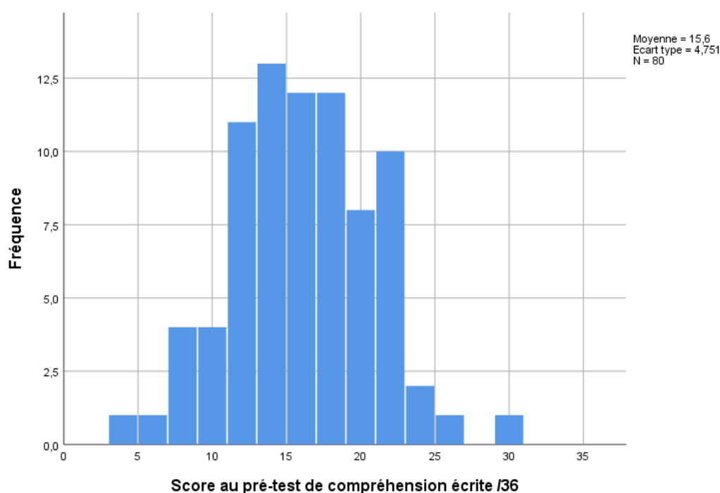
Figure 10 : Histogramme des scores en compréhension écrite pour les élèves ayant un score de fluence compris entre 90 et 100 MCLM
