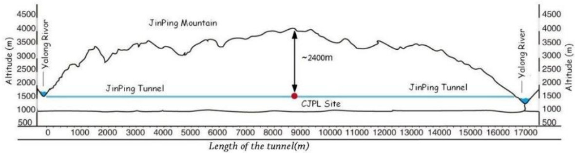
Figure 2-3 : Positionnement du Laboratoire CJPL dans les montagnes du JinPing. Le laboratoire est protégé des rayonnements cosmiques par une épaisseur de 2400 mètres de roches, l'accès au site se réalise par le tunnel JinPing creusé dans la montagne. [29]
