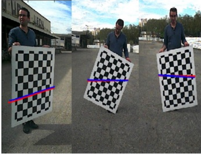
FIGURE III.14: Projection des points LIDAR sur la mire de calibration (Les lignes rouges : solution initiale, Les lignes bleues : la solution optimisée)
