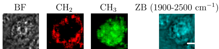
Figure 4.8 – Images d'une cellule HEK en prophase en lumière blanche (BF), celles issues des raies \text{CH}_2 et \text{CH}_3 et celle issue de toute la zone blanche (1900-2500 \text{cm}^{-1} ). Barre d'échelle, 5 \mu\text{m} .
