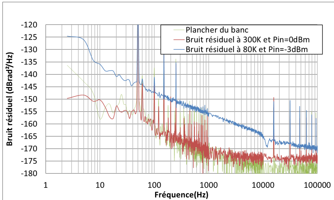
Figure III-9 : Comparaison entre le bruit de phase résiduel du BFU790 à 300K (courbe rouge) et celui à 80K (courbe bleue). Composant sur 50\ \Omega . Fréquence 1 GHz. I_C = 26\text{mA} et V_{CE} = 2\text{V}
