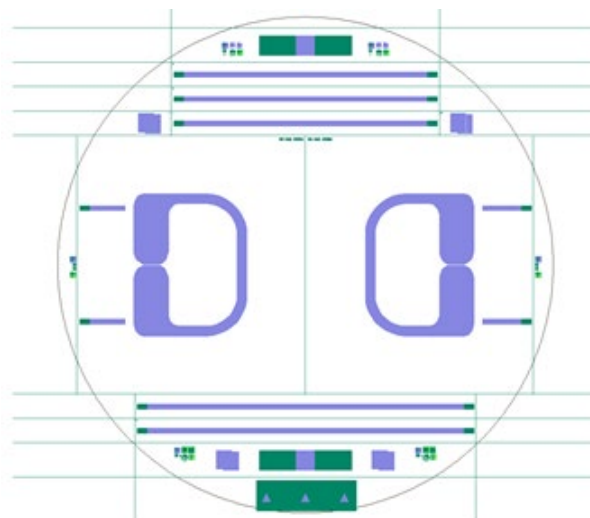
Figure II-8: Schéma du résonateur utilisé pour les premiers tests (cavité de cuivre plongée dans l'azote).
