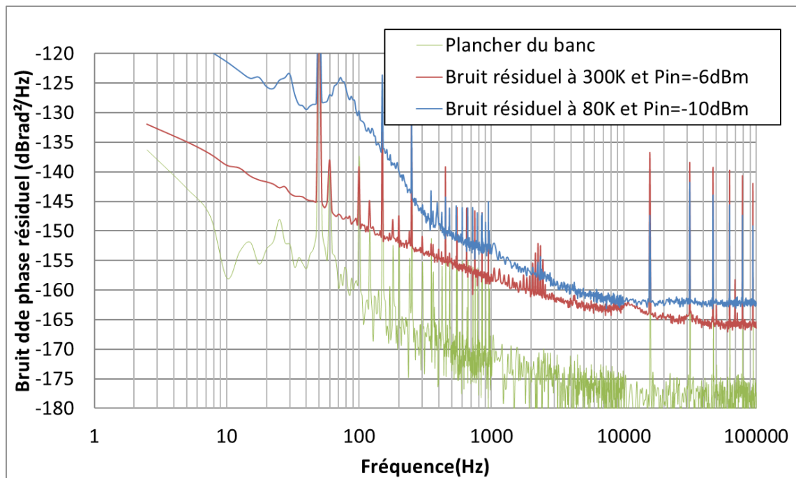
Figure III-10: Comparaison entre le bruit de phase résiduel du BFP620 à 300K (courbe rouge) et celui à 80K (courbe bleue). Composant sur 50\ \Omega . Fréquence 1 GHz. I_C = 26\text{mA} et V_{CE} = 2\text{V} à température ambiante et I_C = 11\text{mA} et V_{CE} = 2\text{V} à basse température.
