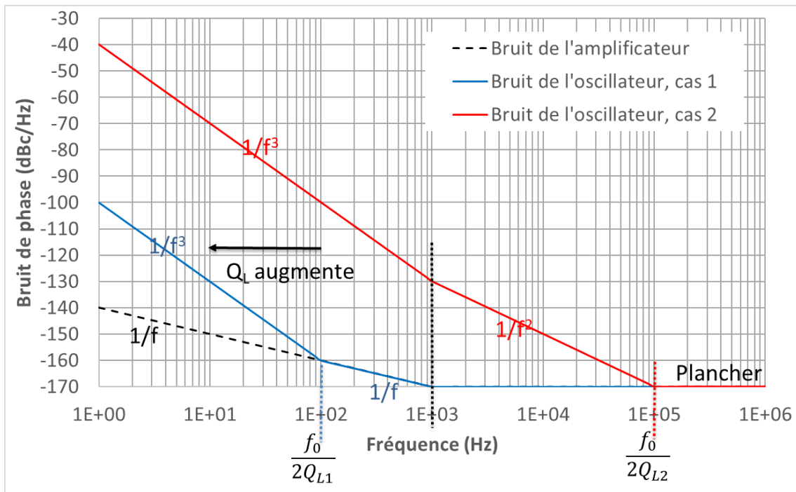
Figure I-9: Illustration du phénomène de conversion du bruit de phase dans une boucle d'oscillation (Equ.1.21) pour différents facteurs de qualités (Courbe bleue : Q_L=5\,000\,000 ; Courbe rouge : Q_L = 5\,000 ). Avec f_0=1 GHz, niveau de bruit en 1/f = -157 dBrad 2 /Hz @ 100 Hz (amplificateur de boucle), et un plancher de bruit PL = -167 dBrad 2 /Hz.
