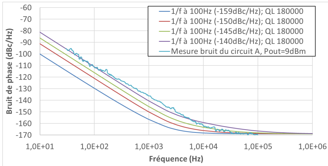
Figure IV-23: Modèle de Leeson du circuit A avec variation du bruit de l'amplificateur
