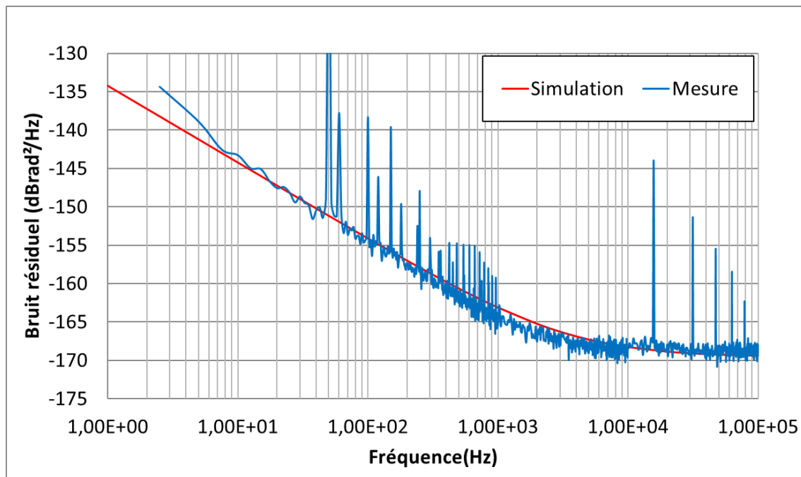
Figure III-22: Comparaison mesures-modèle du bruit de phase résiduel du transistor BFP650 à 1 GHz et à 80 K ( I_c = 20 mA et V_{ce} = 2 V)
