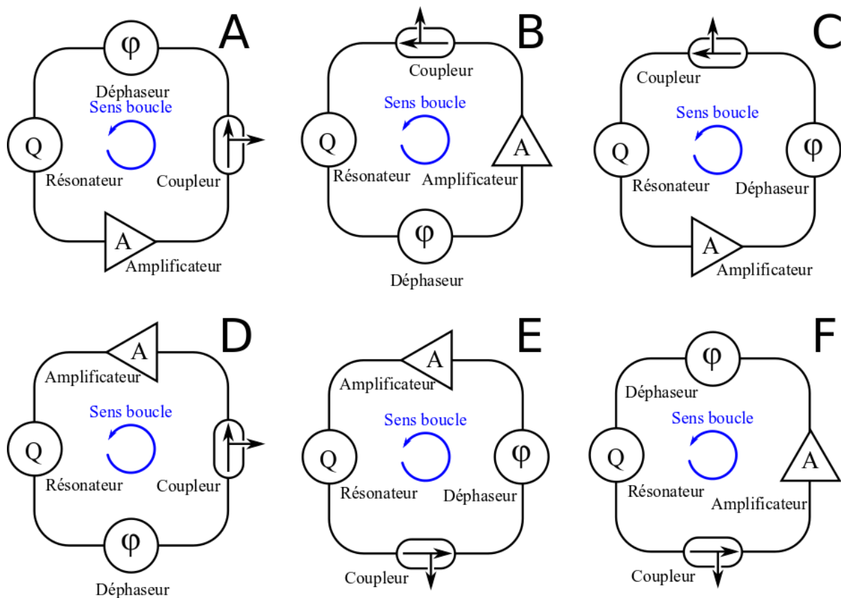
Figure IV-7: Différentes possibilités de boucles d'oscillation
