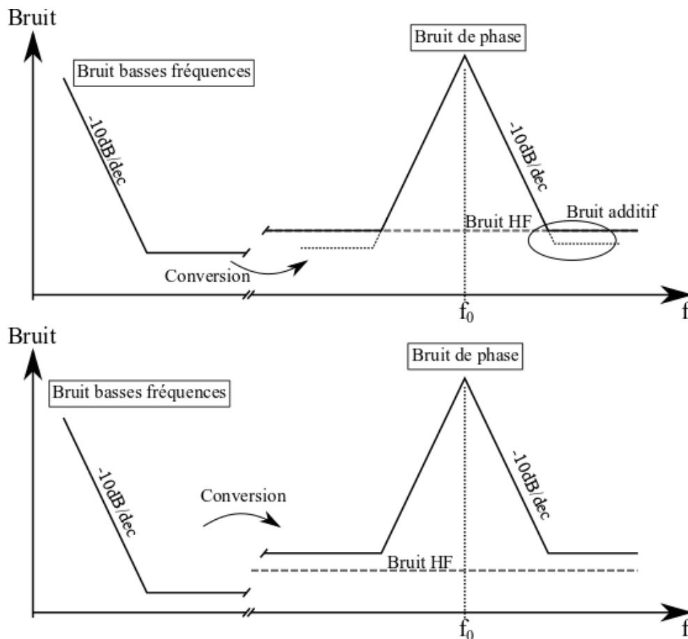
Figure I-12: Principe de conversion du bruit basse fréquence en bruit de phase. Cas A : contribution majeure du bruit additif HF loin de la porteuse ; Cas B : contribution majeure du bruit basse fréquence converti loin de la porteuse.
