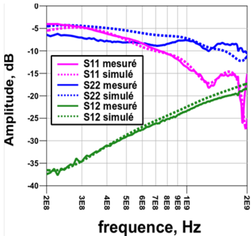
Figure III-31 : Comparaison mesures-modèle en amplitude des paramètres S de l'amplificateur, T = 80\text{K} , I_c = 10\text{mA} , V_{CE} = 2\text{V}
