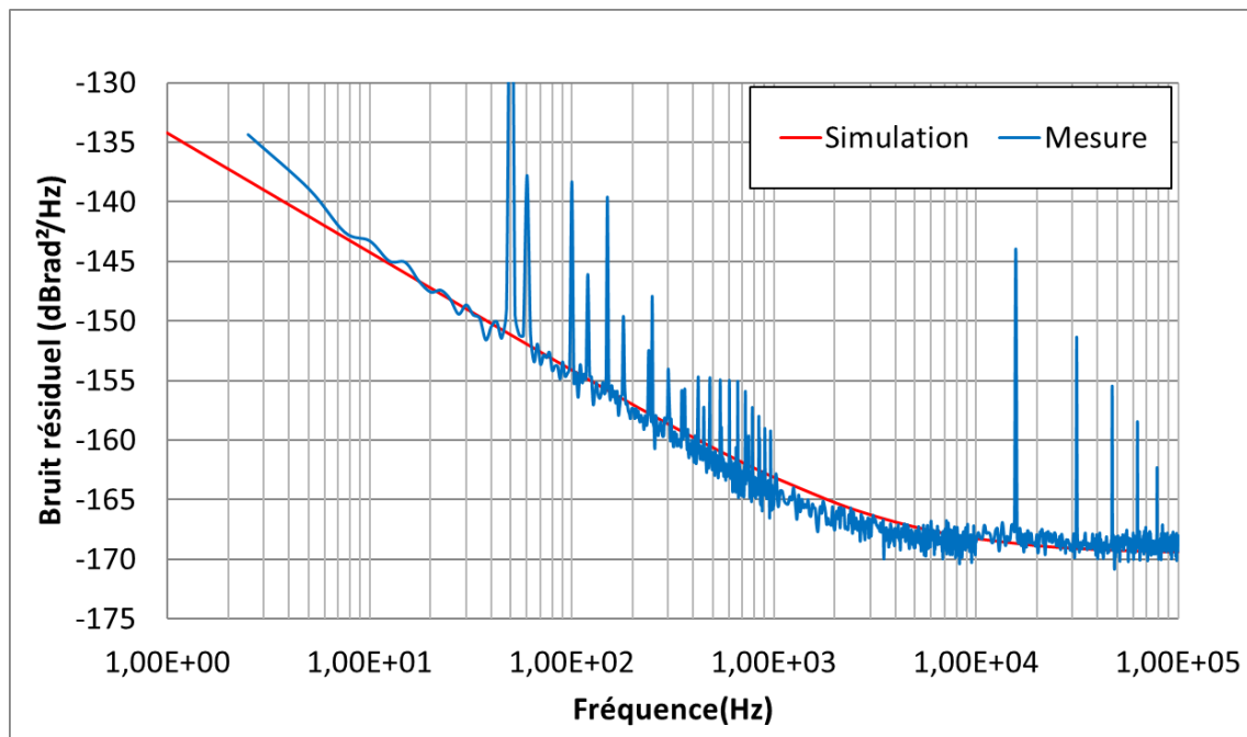
Figure III-22: Comparaison mesures-modèle du bruit de phase résiduel du transistor BFP650 à 1 GHz et à 80 K ( I_c = 20 \text{ mA} et V_{ce} = 2 \text{ V} )
