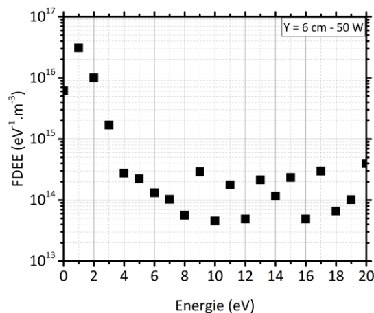
Figure I-16 FDEE expérimentale déterminée à 50 W aux positions X = 0 cm et Y = 6 cm à partir de la formule de Druyvesteyn
