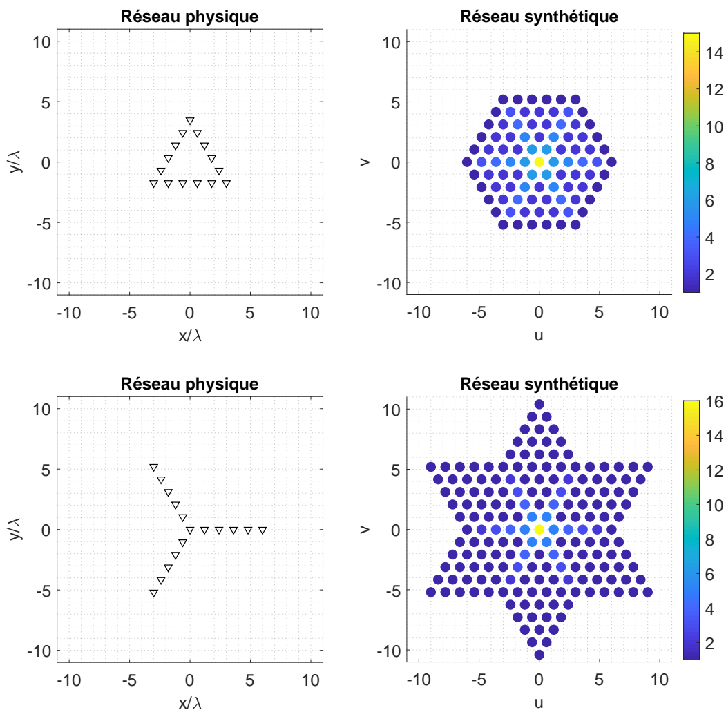
FIGURE 1.31 – Étude des réseaux en forme de triangle et de "Y" et des réseaux synthétiques associés. La redondance des éléments rayonnants fictifs est représentée en couleur.
