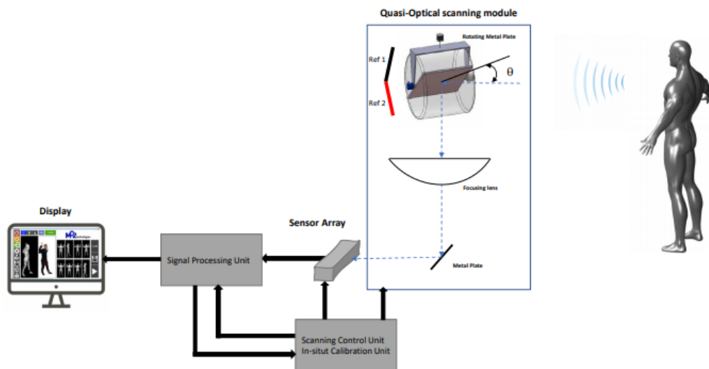
FIGURE 1.24 – Prototype du système quasi optique MM-imager fonctionnel à 90 GHz [36].
