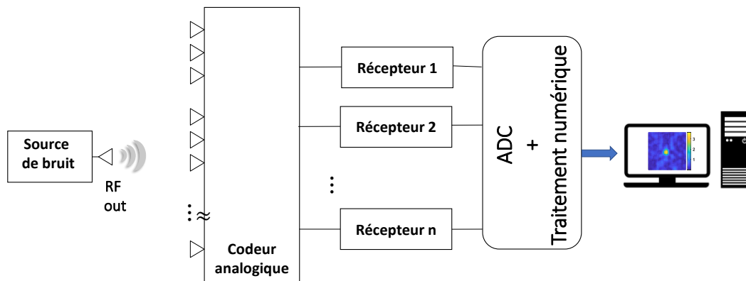
FIGURE 3.24 – Schéma d'un système d'imagerie computationnelle interférométrique opérant dans le domaine temporel.
