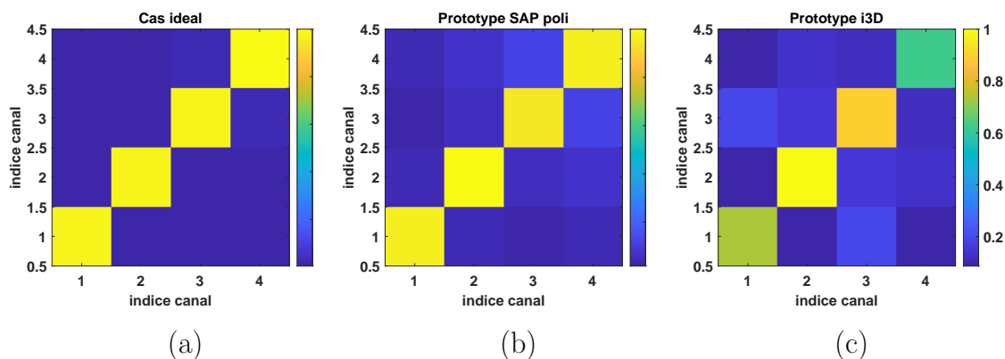
FIGURE 2.7 – Comparaison des matrice de corrélation des fonctions de transfert d'une cavité chaotique 4 \times 1 (Prototype SAP et 3D) avec le cas idéal.
