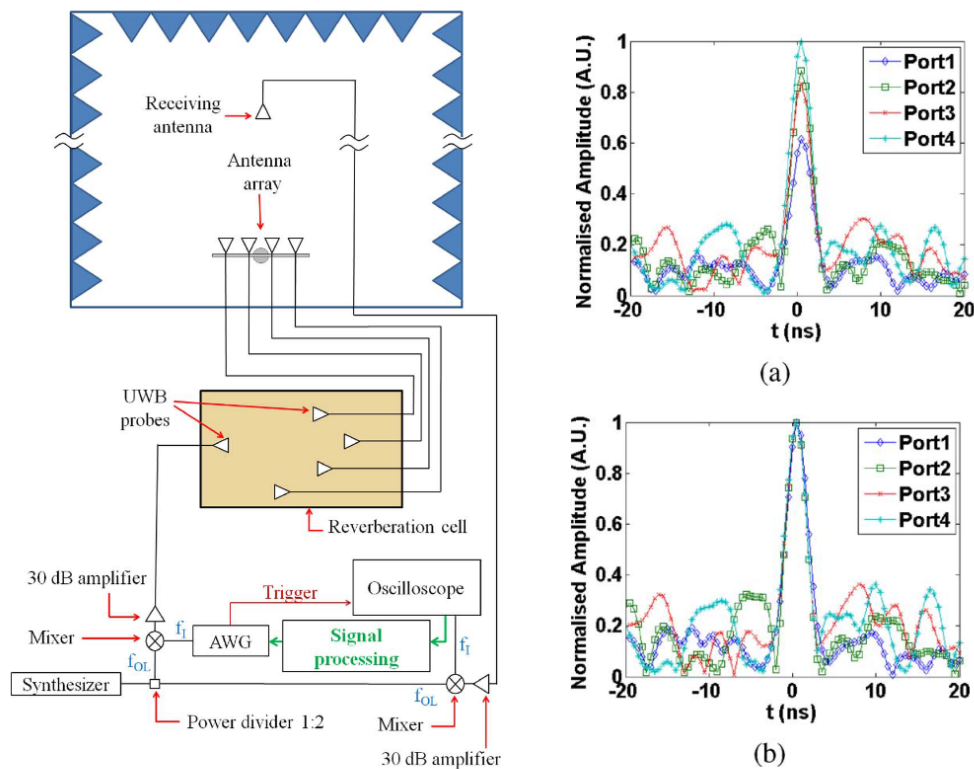
FIGURE 1.38 – Validation d'une technique de pré-correction permettant d'améliorer les reconstructions réalisées. Les distorsions déterministes causées par des réponses impulsionnelles précaractérisées sont corrigées à l'instant de focalisation afin d'améliorer le processus de formation de faisceau numérique réalisé par technique computationnelle [102].
