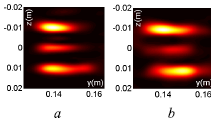
FIGURE 1.49 – Comparaison des résultats d'imagerie de simulation (a) et de mesures (b) d'une cible à trois bandes avec la configuration une cavité en transmission et une en réception [117].
