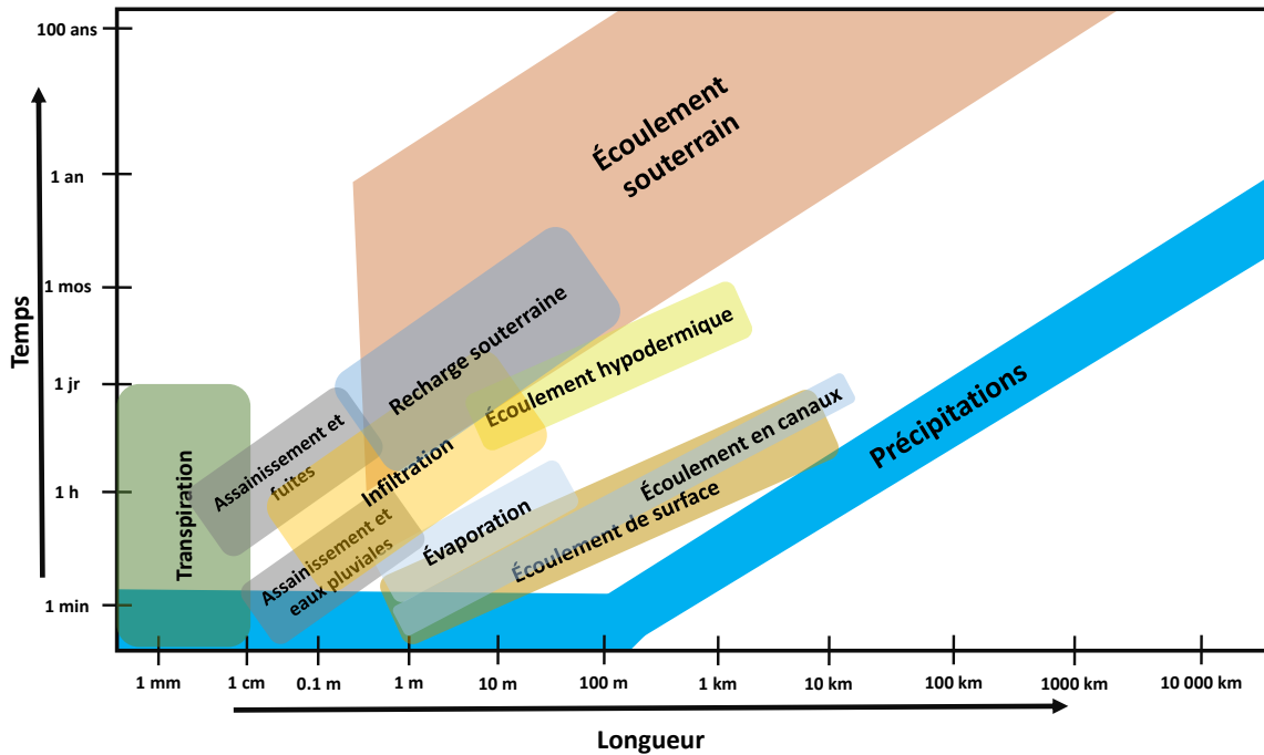
Figure 1.1. Échelle spatiale et temporelle des processus hydrologiques en milieu urbanisé. Cette figure est reprise de Salvatore, Bronders et Batelaan (2015). On définit l'échelle spatiale ou temporelle caractéristique comme la région dans l'espace ou dans le temps dans laquelle le processus prend place, où ses flux varient, ou alors la résolution spatiale ou temporelle avec laquelle il est le mieux mesuré.
