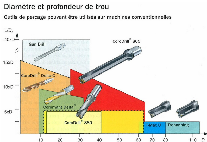
FIGURE 1.5 – Typologie d'outils de perçage en fonction de la longueur et du diamètre du trou à réaliser [2]
