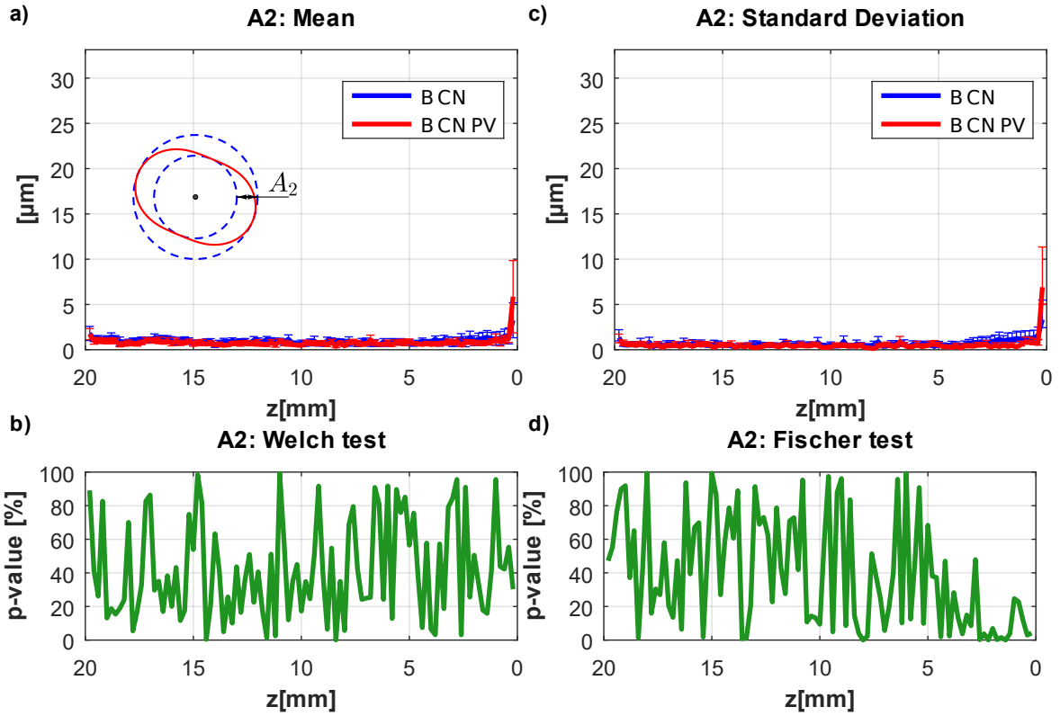
FIGURE D.6 – Comparaison de l'amplitude du second harmonique A_2 g n r  par l'outil B en per age conventionnel versus per age vibratoire   oscillations forc es.
