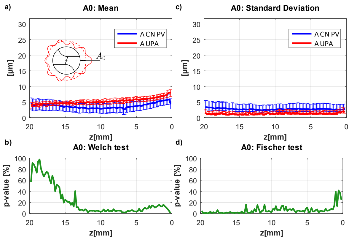
FIGURE D.17 – Comparaison de l’agrandissement A_0 généré par l’outil A en perçage vibratoire à oscillations forcées versus perçage avec UPA.
