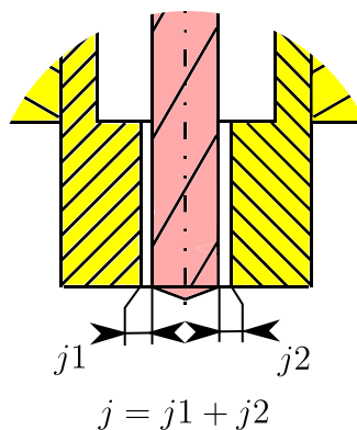
FIGURE 2.8 – Illustration du jeu canon j
