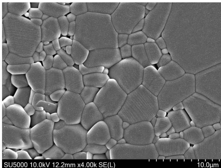
Figure III-36 : Micrographie du mélange d'alumines 6G4P mis en forme par SLA et fritté de manière conventionnelle
