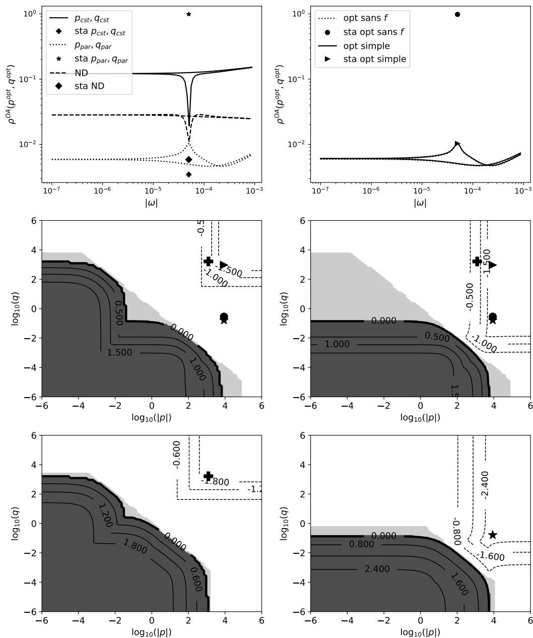
FIGURE 4.11 – En haut à gauche : taux de convergence théorique \rho^{KPP}(\omega, p^{opt}, q^{opt}) pour les différents coefficients de Robin. \rho(\omega, p_{cst}^{opt}, q_{cst}^{opt}) , \rho(\omega, p_{par}^{opt}, q_{par}^{opt}) et \rho_{ND}(\omega) sont indiqués. En haut à droite : \rho(\omega, p^{opt}, q^{opt}) et \rho(\omega, p^{opt}, q^{opt}) . Au milieu et en bas : différents profils de \max(\rho(\omega, p, q)) pour |\omega| \in [\pi/T, \pi/\delta t] en fonction de |p| et q . Sur les panneaux du milieu, on ne considère pas les fréquences |\omega + f| < 10^{-11} à droite, et on les considère à gauche. Sur les panneaux du bas : \max(\rho_{z^\infty-h}^{cst}(\omega, p, q)) à gauche, et \max(\rho_h^{par}(\omega, p, q)) à droite.
