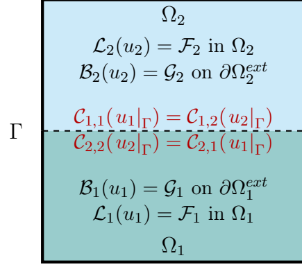
FIGURE 2.8 – Schéma d'un problème multiphysique décomposé en deux sous-problèmes dans le cadre stationnaire
