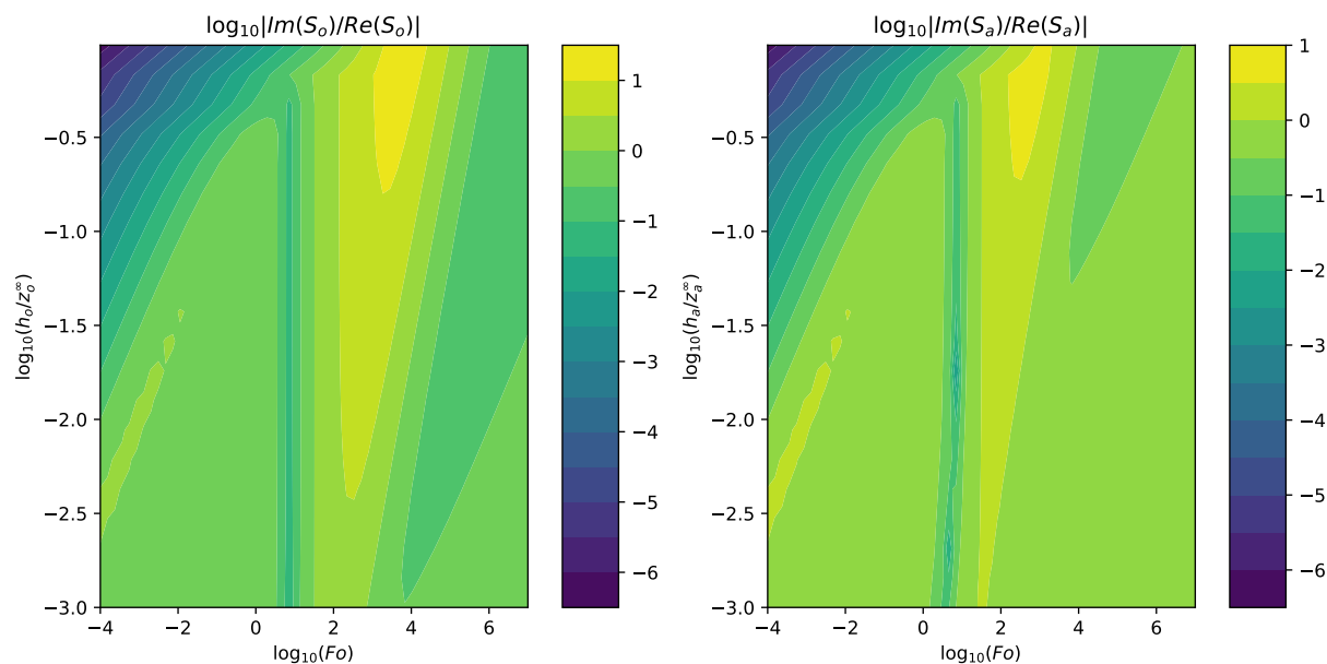
FIGURE 4.9 – Profil de \log_{10}(|\text{Im}(\mathcal{S}_\alpha)|/|\text{Re}(\mathcal{S}_\alpha)|) en fonction de \log_{10}(Fo) et de \log_{10}(h_\alpha/z_\alpha^\infty) , pour déterminer y_\alpha . À gauche : domaine océan ; à droite : domaine atmosphère.
