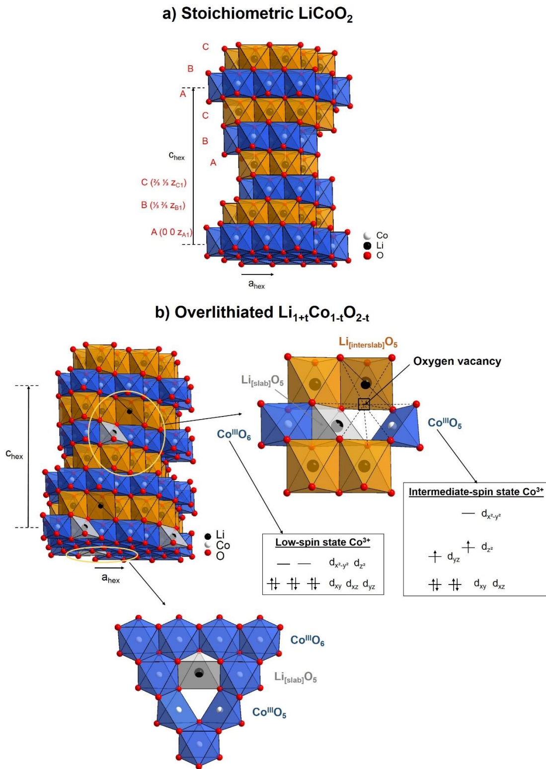
Figure 1. a) Représentation schématique de la structure de \text{LiCoO}_2 dit “stoechiométrique” ( \text{Li}/\text{Co} = 1.00 ) et de son équivalent surlithié (b), de formule « \text{Li}_{1+t}\text{Co}_{1-t}\text{O}_{2-t} » ( \text{Li}/\text{Co} > 1.00 ).
