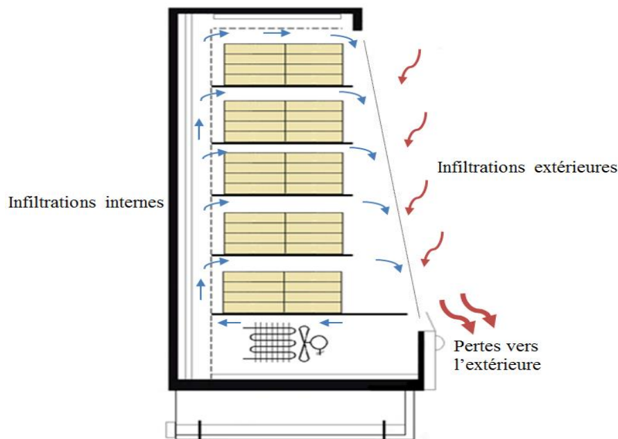
Figure 2 : Ecoulements dans un meuble frigorifique ouvert
