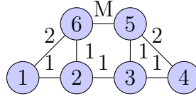
Figure 1: Exemple d'une instance avec une solution optimale différente pour Min p-Center et RpCP pour p = 2 .
