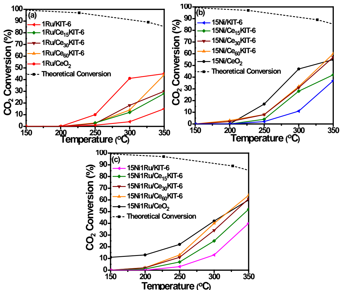
Figure 3.2: Conversion de \text{CO}_2 en fonction de la température en présence des différents catalyseurs (a) 1\text{Ru}/\text{Ce}_x\text{KIT-6} , (b) 15\text{Ni}/\text{Ce}_x\text{KIT-6} , et (c) 15\text{Ni}1\text{Ru}/\text{Ce}_x\text{KIT-6}
