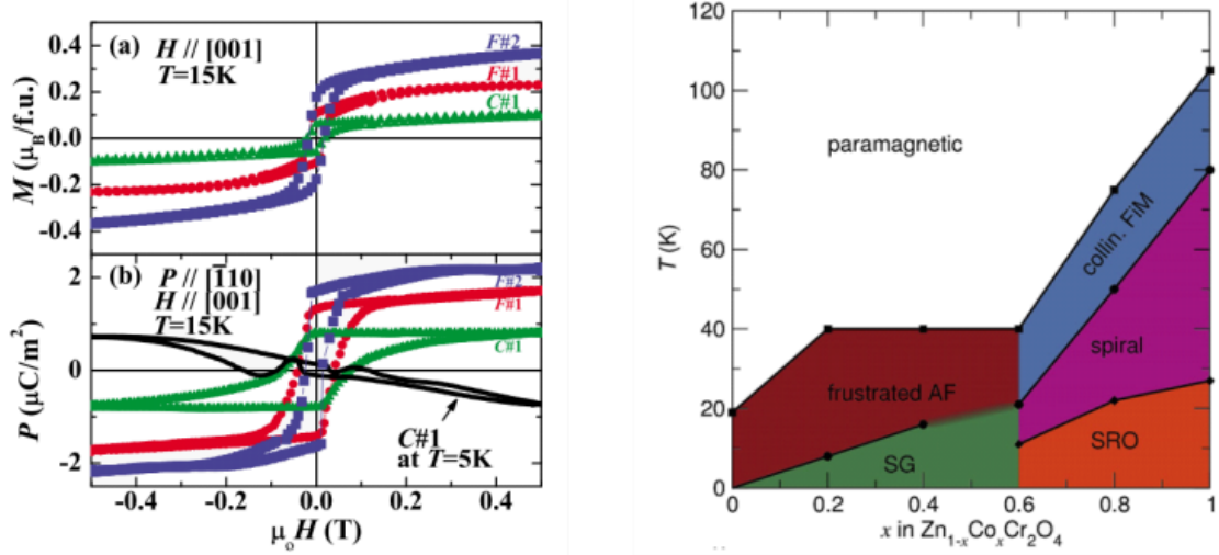
Figure B.5: À gauche: dépendance du champ magnétique de a) Magnétisation selon la direction [001] b) Polarisation selon la direction [\bar{1}10] mesurée à T = 15 K pour \text{Co}(\text{Cr}_2 - x\text{Co}_x)\text{O}_4 . C#1, F#1 et F#2 désignent respectivement x = 0, 0,14 et 0,18 [149]. À droite: diagramme de phase magnétique d'une famille \text{Zn}_{1-x}\text{Co}_x\text{Cr}_2\text{O}_4 . Les acronymes suivants signifient AF - antiferromagnétisme, FiM - ferrimagnétisme, SG - spin-glass, SRO - commande à courte portée [150].
