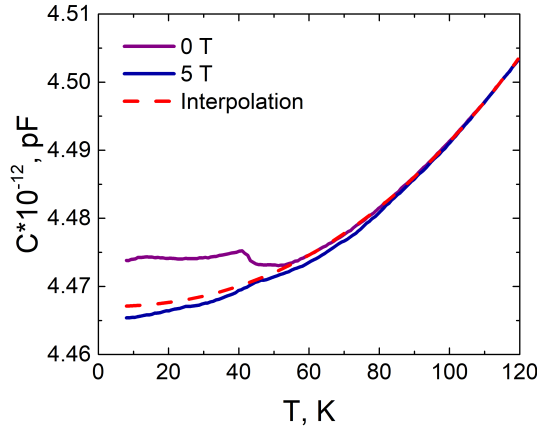
Figure B.25: Evolution de la température de la capacité de champ zéro (courbe violette), de la capacité à B = 5 T (courbe bleue) et de l'interpolation haute température de la capacité de champ zéro de \text{Co}_{3,99}\text{Zn}_{1,01}\text{TeO}_8
