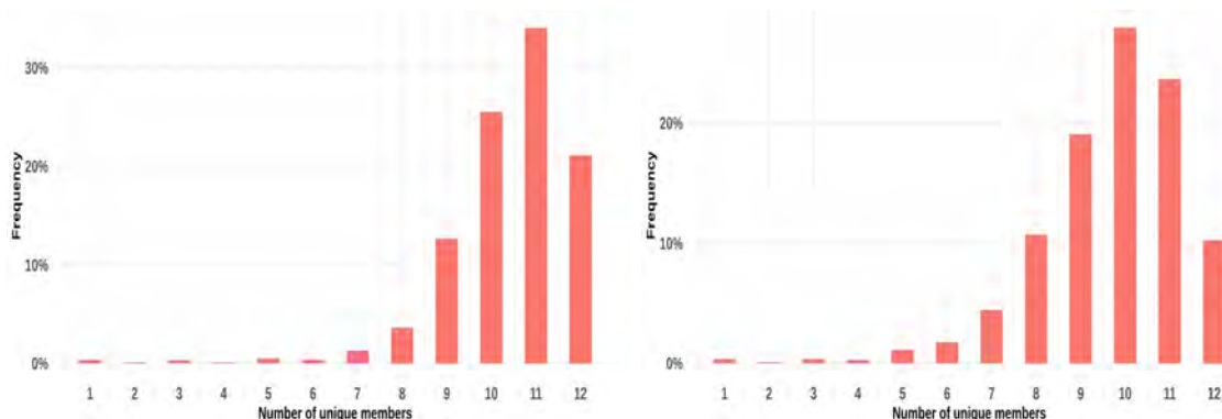
FIGURE 9.4 – Distribution de la taille effective des ensembles NN, calculée pour 11 sites du tableau 7.1 sur la période 06/01/2018-31/05/2019, gauche : après le raccordement à 48h et droite : après le raccordement à 96h.
