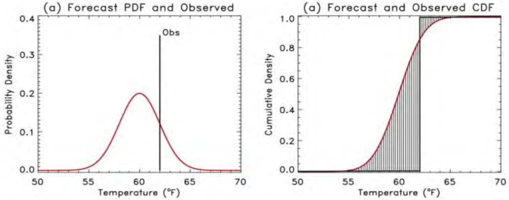
FIGURE 6.1 – A gauche la distribution de probabilité de la prévision (courbe rouge) et la référence (trait vertical noir), à droite les fonctions de répartition associées. Le CRPS correspond à l’aire entre les deux fonctions de répartition (surface grisée). L’axe horizontal représente la variable à prévoir. Source : Hersbach, 2000
