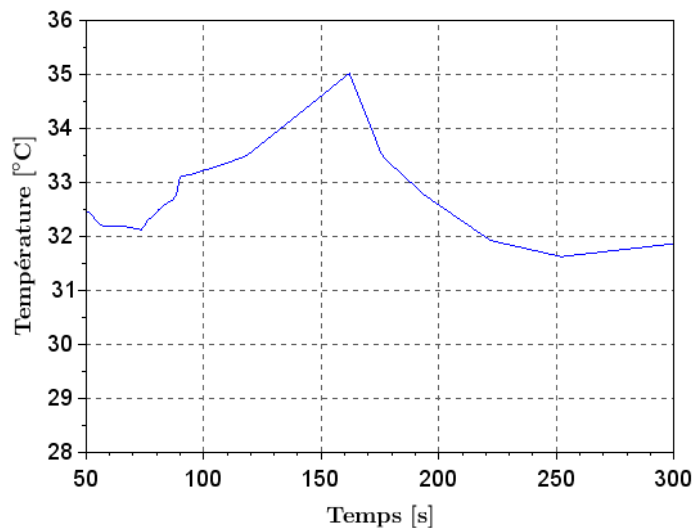
Figure 5.16 : Variation de type aléatoire de la température du thermorécepteur
