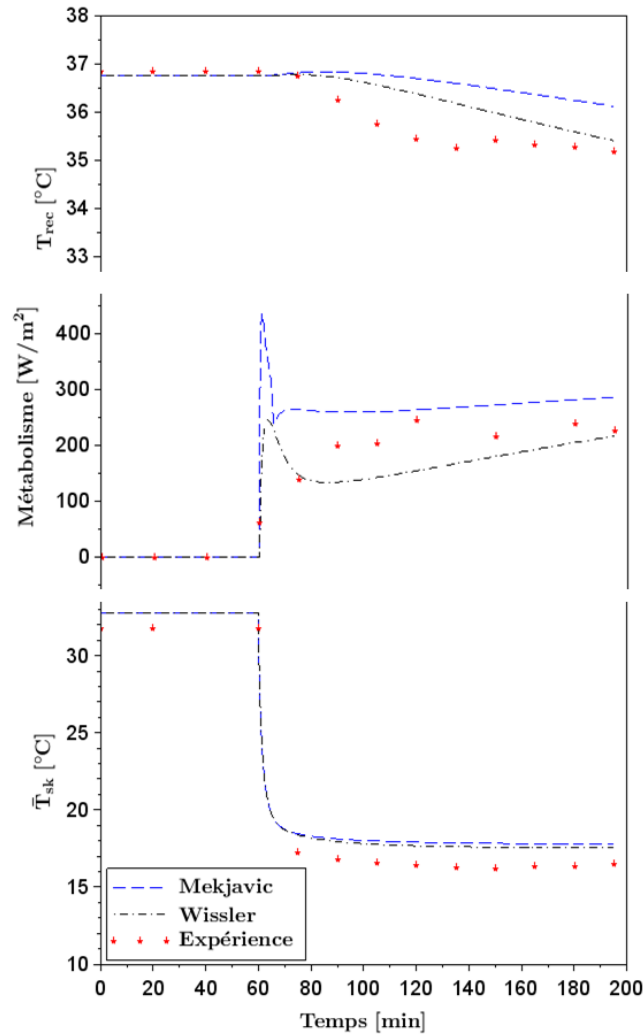
Figure 5.21 : Température rectale, métabolisme de frissonnement et température moyenne cutanée mesurés par Lee et al. [178] et calculés par les modèles de frissonnement de Wissler [11] et de Mekjavic et Morrisson [16] couplé au modèle passif de Wissler (Equation (181))
