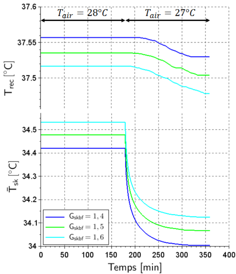
Figure 6.8 : Effet du gain G_{skbf} sur la température rectale T_{rec} et la température moyenne cutanée T_{sk}
