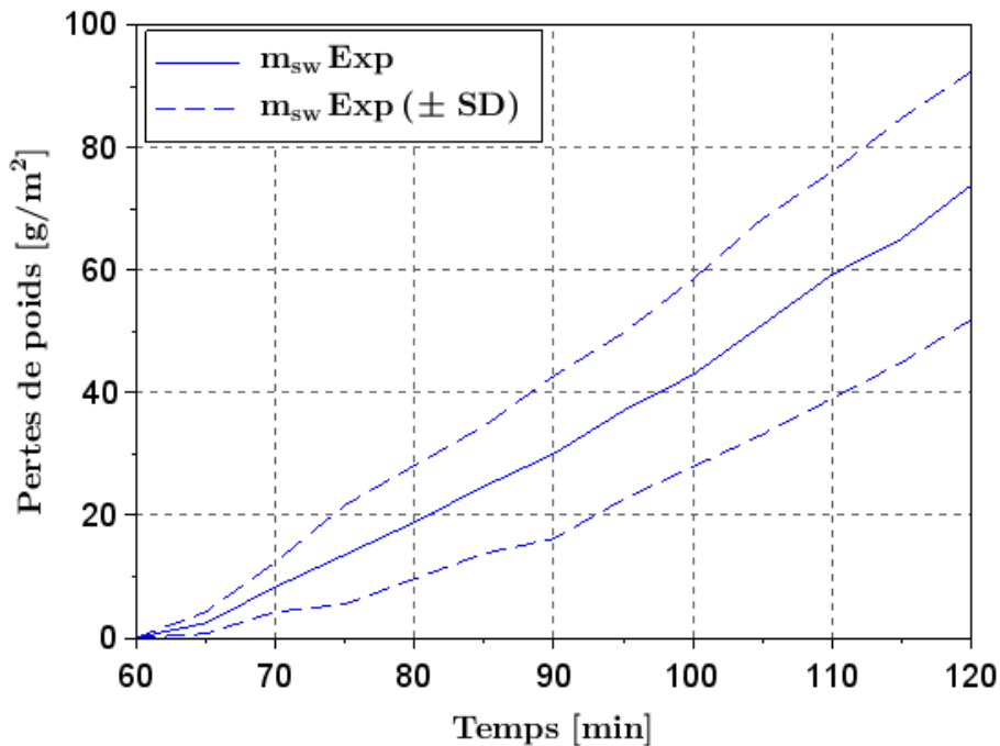
Figure 5.34 : Perte de poids mesurée pour les expérimentations d'Ooka et al. [193]. m_{sw} Exp : Perte de poids moyenne mesurée ; m_{sw} Exp ( \pm SD) : Perte de poids moyenne mesurée \pm un écart-type
