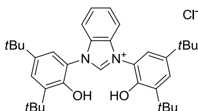
1,3-bis(3,5-di-tert-butyl-2-hydroxyphenyl)-1H-benzo[d]imidazol-3-ium chloride
