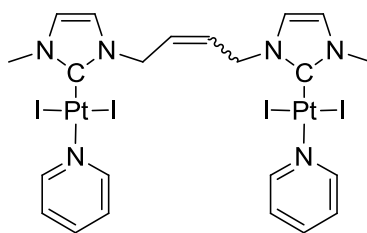
105 : mixture E/Z 1.6/0.4
