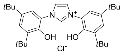
1,3-bis(3,5-di-tert-butyl-2-hydroxyphenyl)-1H-imidazol-3-ium chloride
