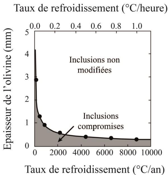
Figure II.1-11 : Épaisseur de l'olivine (i.e. rayon de l'olivine moins le rayon de l'inclusion) en fonction du taux de refroidissement du système. Ce graphique montre la transition entre un comportement en système fermé et ouvert d'une inclusion magmatique. La position de la transition est établie à partir des résultats de simulations numériques (cercles) et calculée à partir de l'équation Dt/x^2 \approx 0.00429 (D est la diffusivité, t le temps et x l'épaisseur de l'olivine entourant l'inclusion ; courbe) pour un intervalle de refroidissement de 100 °C. Figure modifiée de Laubier (2006), modifiée de Gaetani et Watson (2002).
