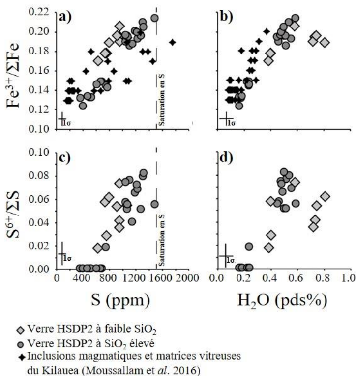
Figure I.3-5 : Rapports \text{Fe}^{3+}/\Sigma\text{Fe} et \text{S}^{6+}/\Sigma\text{S} des verres sous-marins d'Hawaii en fonction de leurs teneurs en \text{H}_2\text{O} et S. (a) \text{Fe}^{3+}/\Sigma\text{Fe} des verres en fonction de leurs teneurs en S, (b) \text{Fe}^{3+}/\Sigma\text{Fe} des verres en fonction de leurs teneurs en \text{H}_2\text{O} (c) \text{S}^{6+}/\Sigma\text{S} des verres en fonction de leurs teneurs en S et (d) \text{S}^{6+}/\Sigma\text{S} des verres en fonction de leurs teneurs en \text{H}_2\text{O} . La ligne pointillée verticale des graphiques (a) et (c) représente la teneur approximative de S à la saturation de sulfure des verres de HSDP2 ayant les plus hautes teneurs en \text{FeO}^* . Figure modifiée de Brounce et al. (2017).
