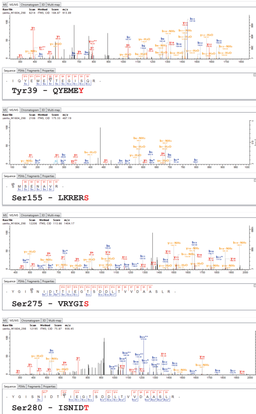
Figure 2. Spectre "MaxQuant" des sites de phosphorylation de PKD pour MFF identifié par spectrométrie de masse. Les produits du dosage de l'activité kinase in vitro (10 µg de protéine humaine recombinante MFF avec 500 ng de protéine humaine recombinante PKD1) ont été digérés avec de la trypsine et soumis à une analyse LC-MS/MS par Oribtrap XL. Les fichiers bruts ont été traités avec le logiciel MaxQuant (version 1.5.2.8). L'identification des peptides a été réalisée en utilisant le moteur de recherche Andromeda contre la base de données humaine SwissProt. Les peptides identifiés ont ensuite été visualisés par Viewer dans MaxQuant et analysés dans le logiciel Skyline. Le site de phosphorylation est marqué en rouge et sa position en acides aminés est indiquée sur toute la longueur de la protéine MFF humaine.
