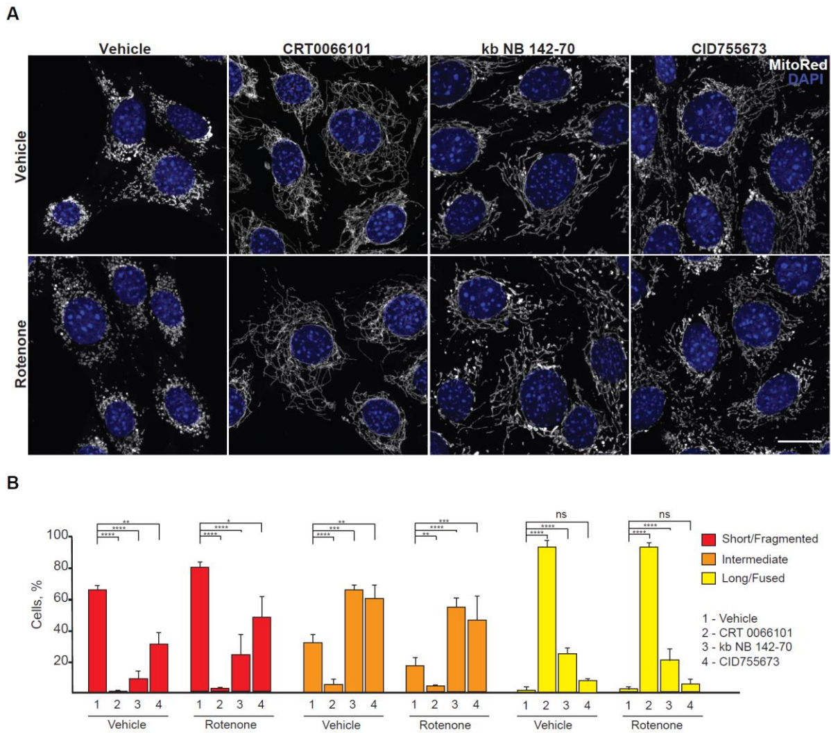
Figure 10. L'activité PKD est requise pour la fission mitochondriale dans les cellules NIH 3T3 de souris. (A) Images de microscopie confocale à fluorescence de cellules NIH 3T3 traitées avec le véhicule (DMSO) ou l'un des trois inhibiteurs de PKD différents (10 \mu M CRT 0066101, 10 \mu M kb-NB 142-70 ou 30 \mu M CID 755673) en combinaison avec le véhicule ou 1 \mu M roténone. Les mitochondries ont été marquées avec du "MitoTracker Red" (pseudocoloré en blanc) et les noyaux ont été marqués avec du DAPI. Barre d'échelle: 20 \mu m. (B) Quantification de la morphologie mitochondriale des cellules présentées en (A). La forme mitochondriale a été classée comme fragmentée (pas de forme claire, moins de 2 \mu m de long), intermédiaire (2 \mu m - 5 \mu m de long) ou longue (tubulaire ou fusionnée, plus de 5 \mu m) et exprimée en pourcentage de cellules selon la catégorie respective des mitochondries. Pour chaque groupe, au moins 300 cellules ont été comptées. Les données sont représentées comme la moyenne \pm SD de trois expériences indépendantes. ****: p < 0,0001 , par ANOVA à deux voies en utilisant le test de comparaison multiple de Dunnett.
