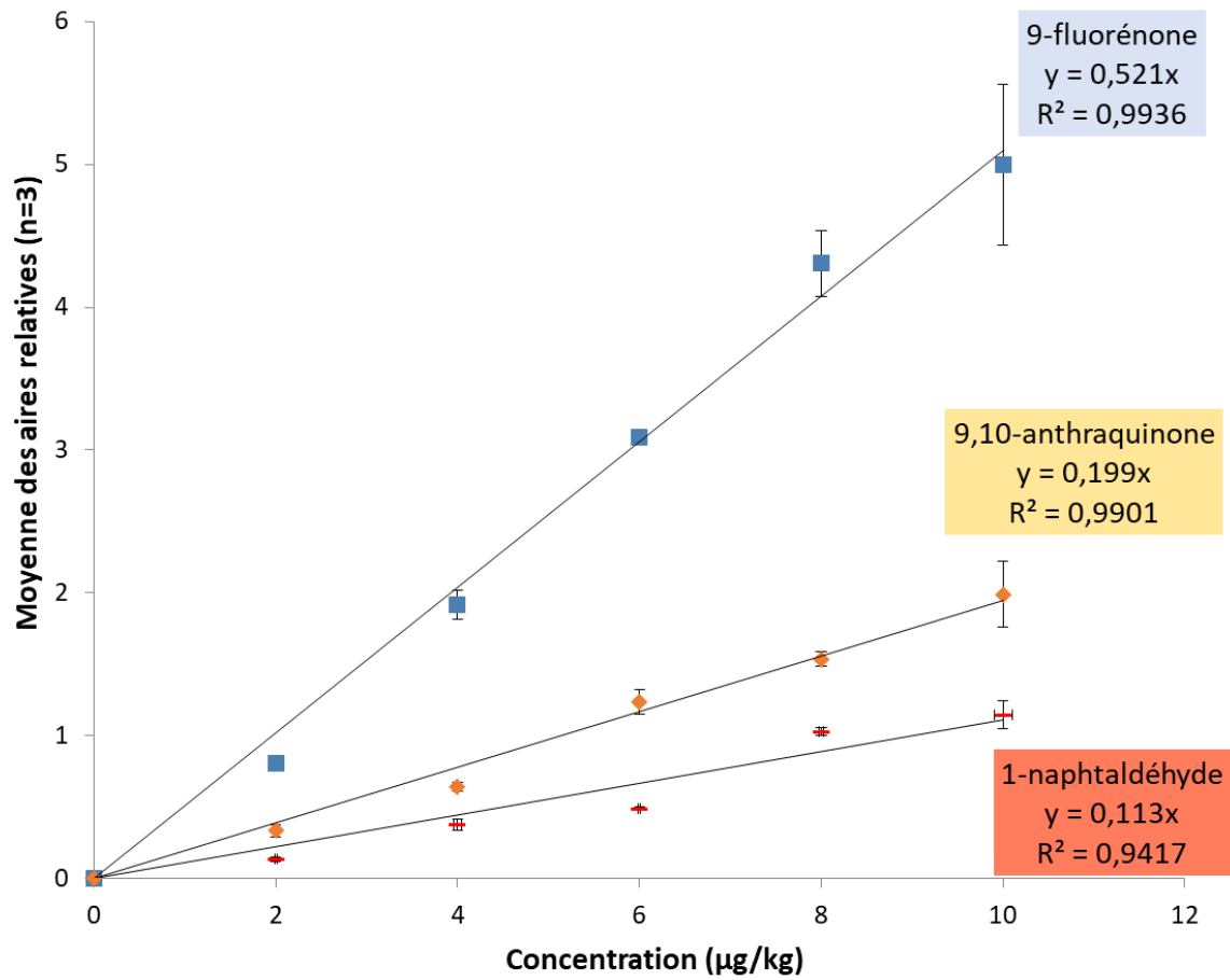
Figure 63 : Droites d'étalonnage pour le 1-naphtaldéhyde, la 9-fluorénone et la 9,10-anthraquinone pour des ajouts compris entre 0 et 10 \mu\text{g}/\text{kg} à un broyat de salade
