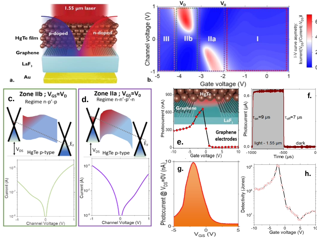
Figure 5 – Schéma du transistor à grille de \text{LaF}_3 , les électrodes de drain et de source sont constituées d'électrodes de graphène interdigitées et le canal est constitué d'un réseau de NC HgTe. (b) Carte 2D de l'asymétrie de la courbe IV, quantifiée par le rapport du courant sous une polarisation donnée et du courant sous la polarisation opposée, en fonction de la tension de canal entre les électrodes de source et de drain, et la tension de grille V_{GS} . Les régions en rouge correspondent aux domaines existants pour une jonction p-n au sein de l'hétérostructure graphène/HgTe/graphène. (c) Alignement de bande de l'hétérostructure dans la configuration n-p'-p et la courbe I-V de rectification associée, dans la zone IIb de la partie b. (d) Alignement de bande de la de l'hétérostructure dans la configuration n-n'-p'-n et la courbe I-V de rectification associée, dans la zone IIa de la partie b. (e) Photocourant en fonction de la tension de grille de l'hétérostructure. (f) Temps de réponse la jonction. (g) Photocourant sous 0 V, lorsque la lumière est chopée à 1 kHz, en fonction de la tension de la grille. (h) Défectivité (rapport signal/bruit) de l'hétérostructure à 1 kHz et à 220 K en fonction de la tension de grille.
