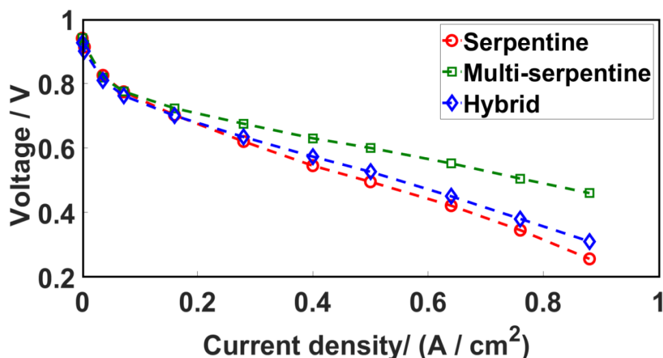
Figure 6 : Courbe de polarisation pour la comparaison de trois géométries (serpentin, multi-serpentine et hybride)
