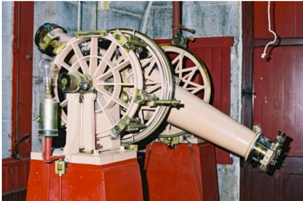
Figure 7.13 – Les deux lunettes Gautier de « seconde génération », de haut en bas : Lyon, Hendaye.
