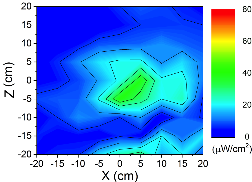
FIGURE 92 – Fuites de champ mesurées sur la face (1) avec 20 W de puissance incidente, une puissance réfléchie de 7 W (mesurés au générateur) et en présence d'un plasma jet d'argon.
