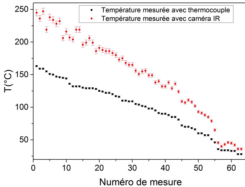
FIGURE 36 – Comparaison des mesures de température de surface de tube entre la caméra IR et le thermocouple.
