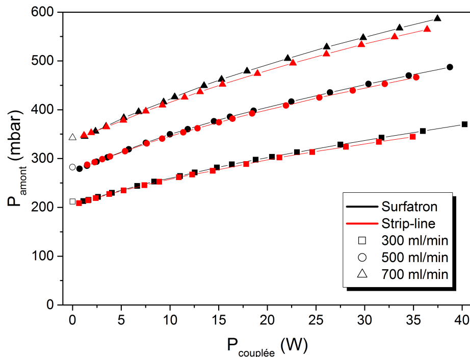
FIGURE 61 – Pression mesurée en amont du capillaire en fonction de la puissance couplée pour les deux applicateurs. Basse pression, fréquence pour le strip-line : 2,45 GHz, pour le surfatron : 2,427 GHz.
