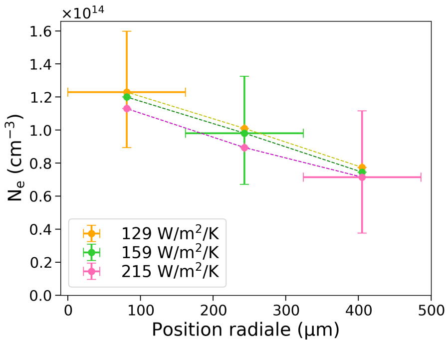
FIGURE 147 – Densité électronique obtenue par élargissement Stark de H_\beta , en fonction de la position radiale pour différentes valeurs du coefficient de transfert thermique imposé, puissance consigne de 50 W.
