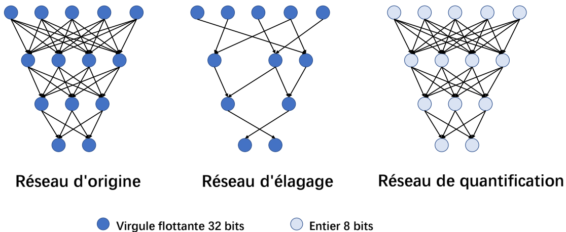
Figure B.1: Réseau d'élagage et Réseau de quantification
