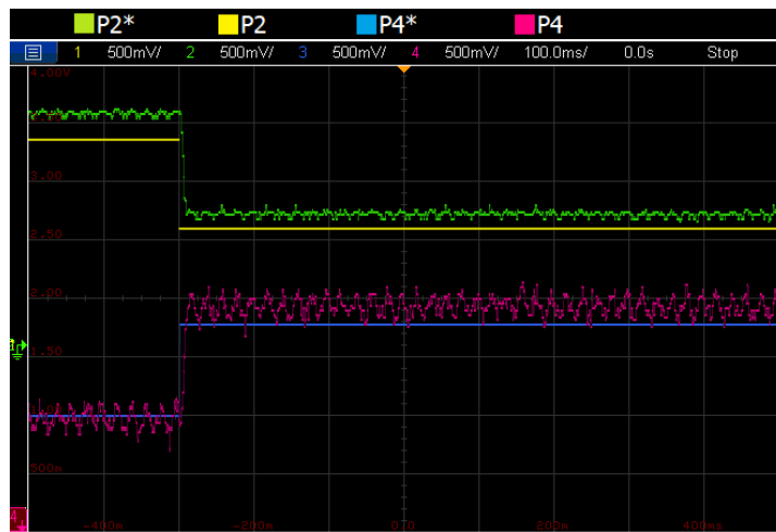
Figure 32: Résultats en boucle ouverte d'une variation en échelon des puissances de référence. Les valeurs de référence ( P2^* et p4^* ) sont indiquées avec les valeurs mesurées correspondantes ( P2 et P4 ).
