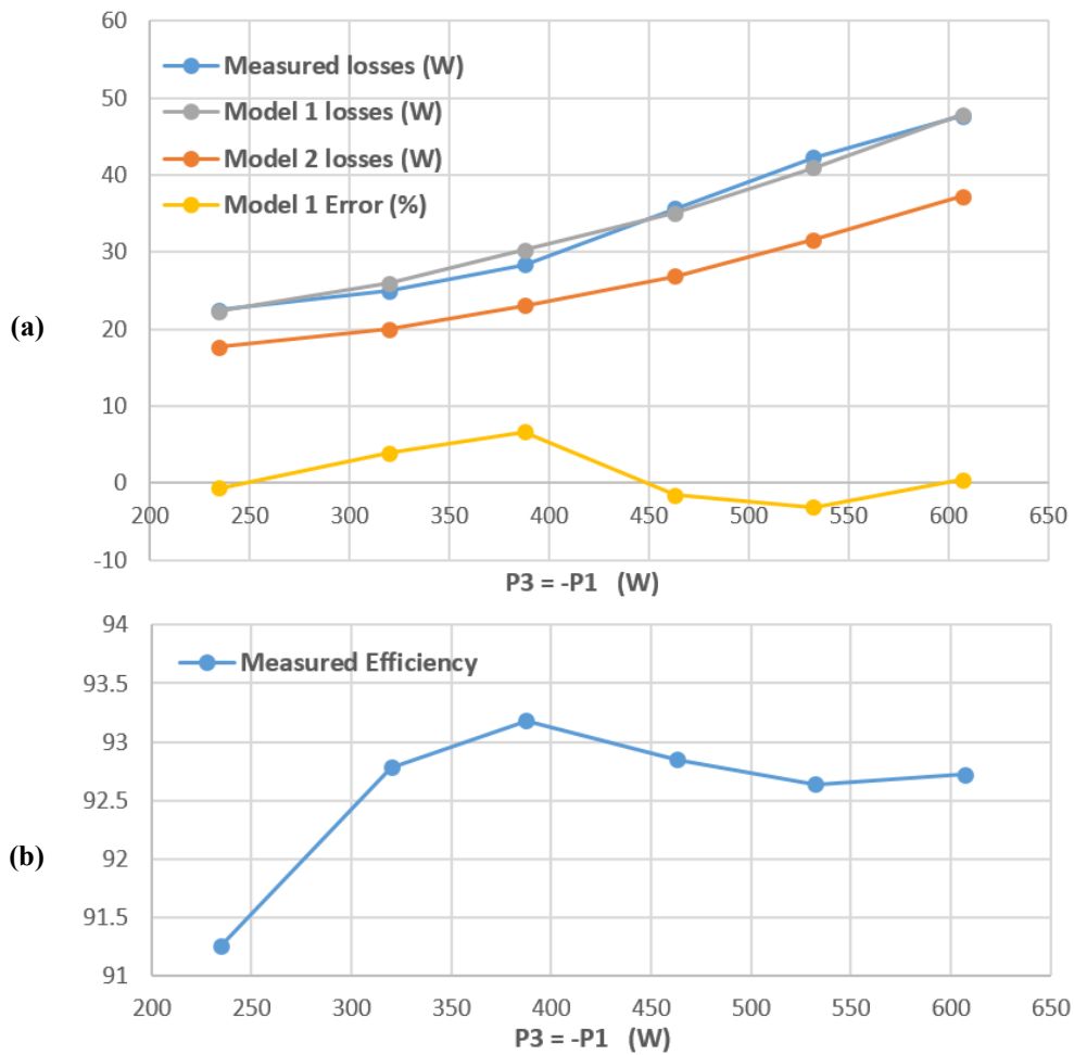
Figure 37: (a) Comparaison des pertes mesurées avec les prédictions des modèles de pertes. (b) Evolution du rendement au fur et à mesure que les puissances augmentent. Le port 1 est la source d'énergie et alimente le port 3. Les transferts de puissance des ports 2 et 4 sont maintenus proches de zéro.
