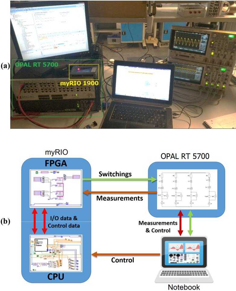
Figure 30: Configuration de la simulation en temps réel avec le simulateur OPAL RT 5700.
