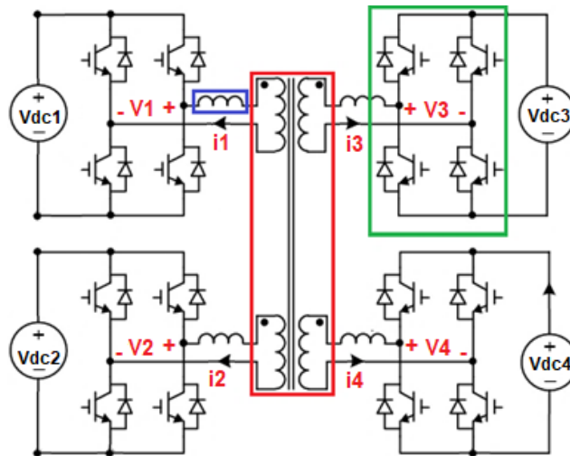
Figure 25: Un convertisseur QAB : la boîte verte montre un active-bridge ; la boîte rouge est un transformateur à enroulements multiples ; la boîte bleue est une inductance, qui peut être soit une inductance externe, soit l'inductance de fuite du transformateur.
