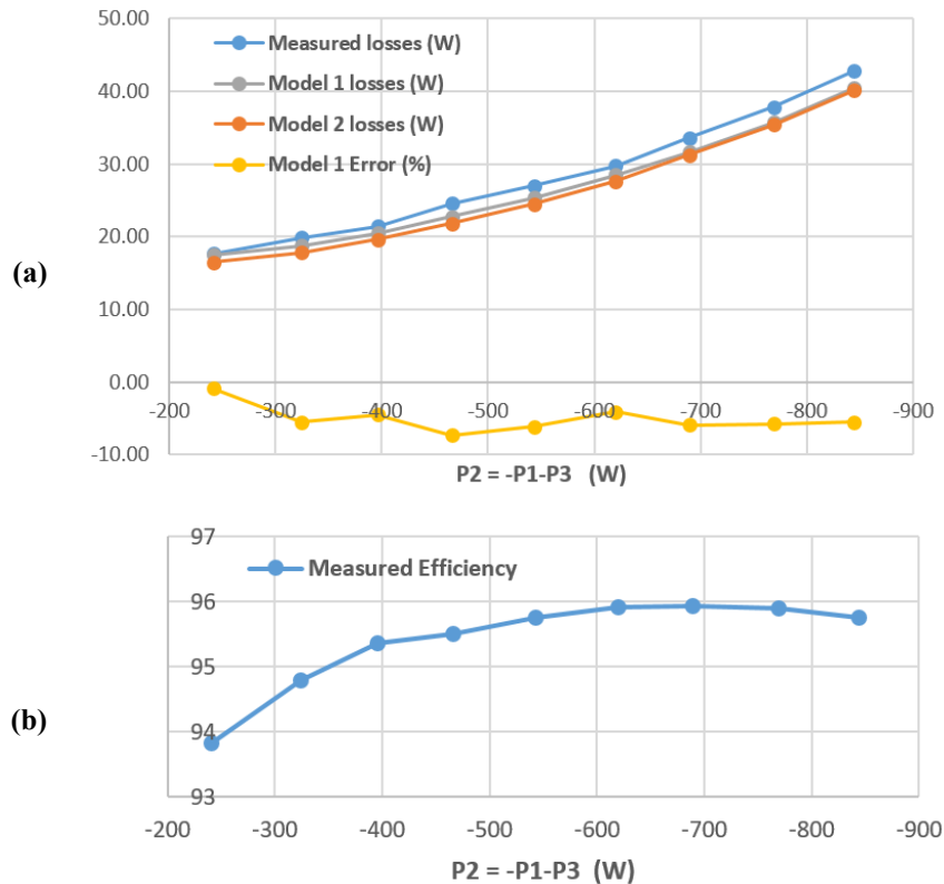
Figure 35: (a) Comparaison des pertes mesurées avec les prédictions des modèles de pertes. (b) Evolution du rendement au fur et à mesure que les puissances augmentent. Le port 2 est la source d'énergie et alimente les ports 1 et 3 de manière égale. Le transfert de puissance du port 4 est maintenu proche de zéro.
