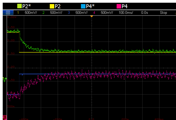
Figure 33: Résultats en boucle fermée du même test que la Figure 0.5. Le système de contrôle est composé d'une boucle de rétroaction PI seule.
