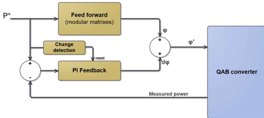
Figure 31: Schéma de commande en boucle fermée avec une boucle feed-forward et une boucle feed-back.
