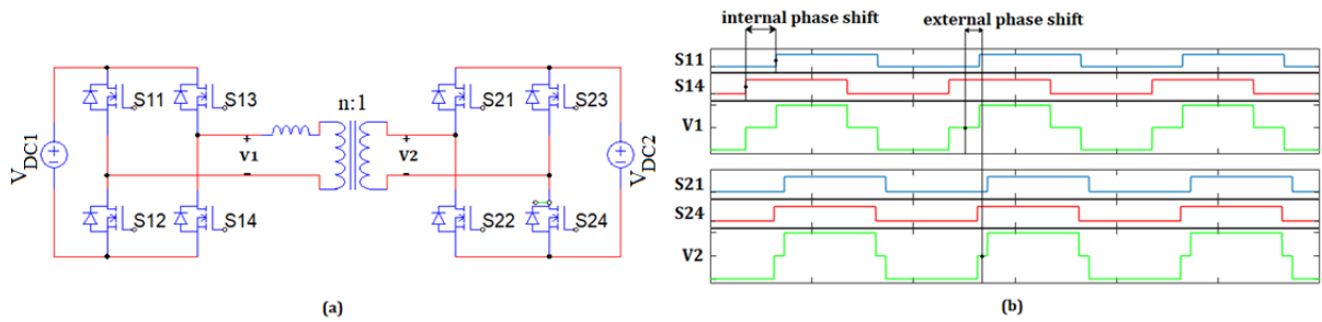
Figure 26: déphasages interne et externe dans la commutation d'un DAB. Les interrupteurs d'un même bras sont commutés de manière complémentaire.
