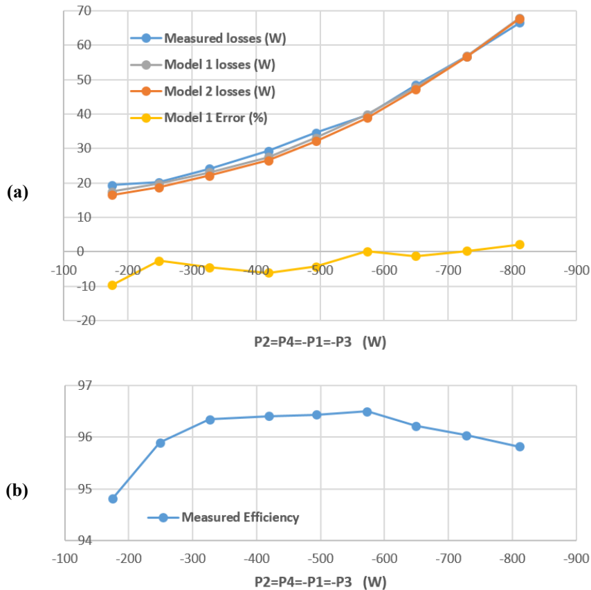
Figure 36: (a) Comparaison des pertes mesurées avec les prédictions des modèles de pertes. (b) Evolution du rendement au fur et à mesure que les puissances augmentent. Le port 2 est la source d'énergie et alimente le port 1 et le port 3 de manière égale. Le transfert de puissance du port 4 est maintenu proche de zéro.
