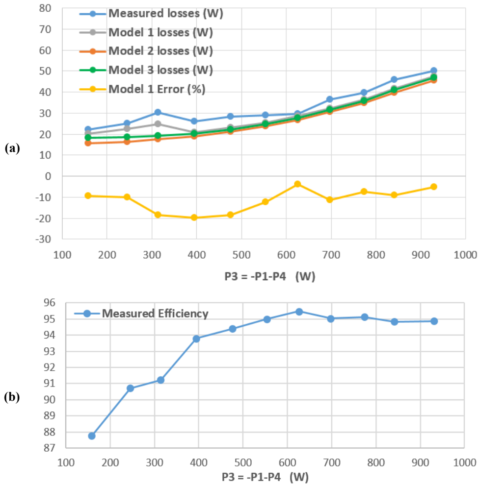
Figure 38: (a) Comparaison des pertes mesurées avec les prédictions des modèles de pertes. (b) Evolution du rendement au fur et à mesure que les puissances augmentent. Les ports 1 et 4 sont les sources d'énergie et alimentent également le port 3. Le transfert de puissance du port 2 est maintenu proche de zéro.
