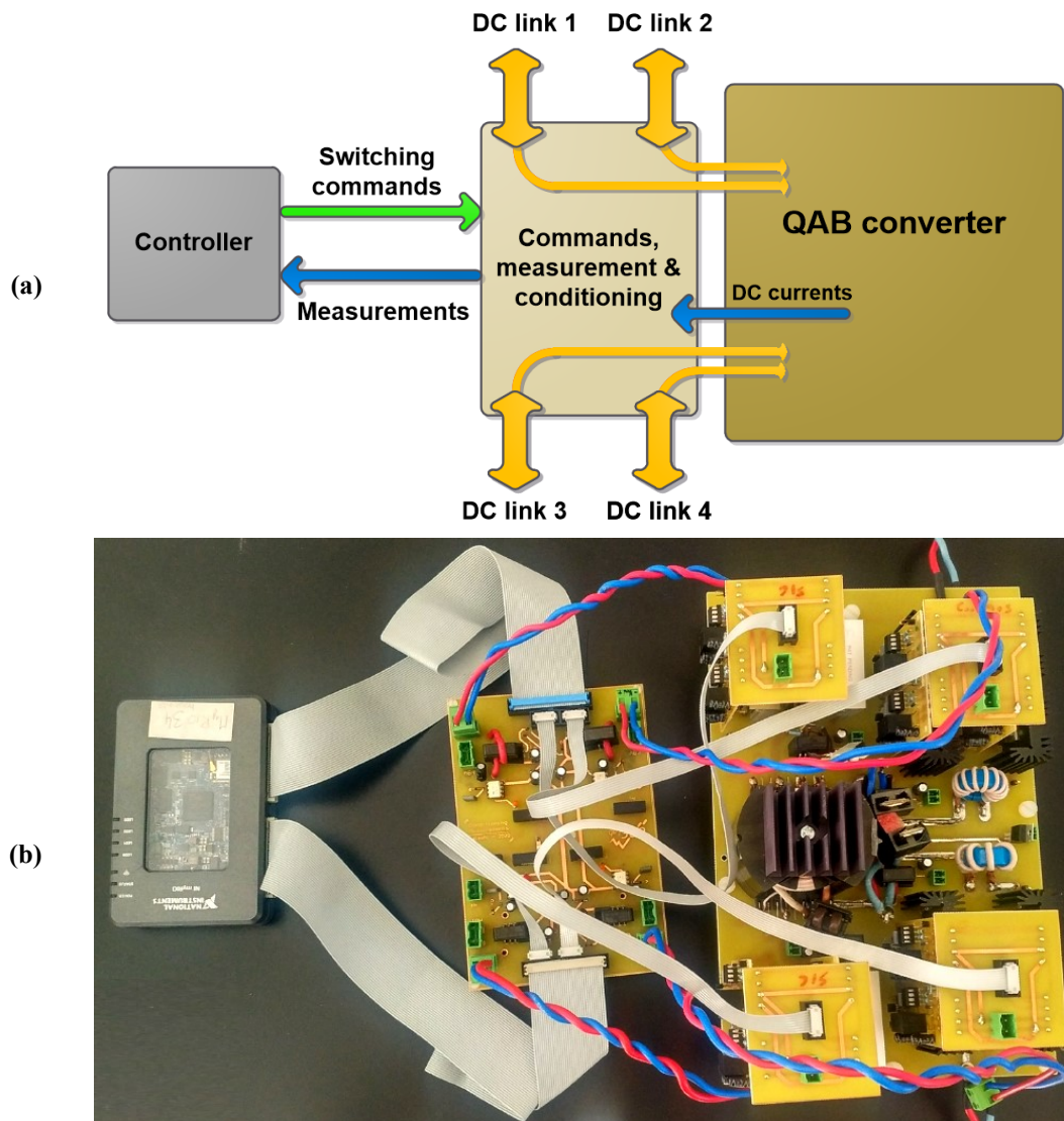
Figure 29: Le banc de test : (a) les schémas et (b) le montage d'essai réel, y compris le convertisseur QAB, la carte de mesure et de conditionnement et le contrôleur. Les flèches jaunes dans (a) indiquent les connexions d'alimentation, et les autres sont des signaux de commande et de mesure.
