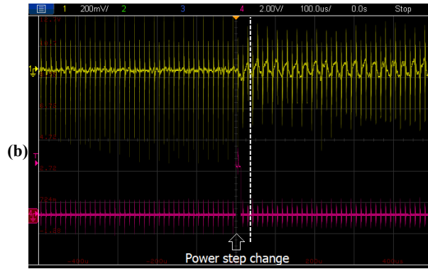
Figure 39: Performance de l'annulation du courant continu pendant les transitoires de puissance. (a) Formation de courant continu pendant les transitoires de puissance lorsque l'annulation est désactivée ; et (b) Prévention de la formation de courant continu lorsque la commande d'annulation est activée. La courbe jaune montre la sortie de la configuration du capteur de courant continu. La ligne pointillée blanche indique le changement du flux de puissance et donc le déphasage, activant la commande de déphasage en deux étapes pour éviter la formation d'un courant continu.
