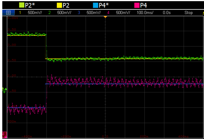
Figure 34: Résultats de la boucle fermée du même test que la Figure 0.5. Le système de contrôle comporte des boucles de rétroaction PI et de rétroaction matricielle activées.
