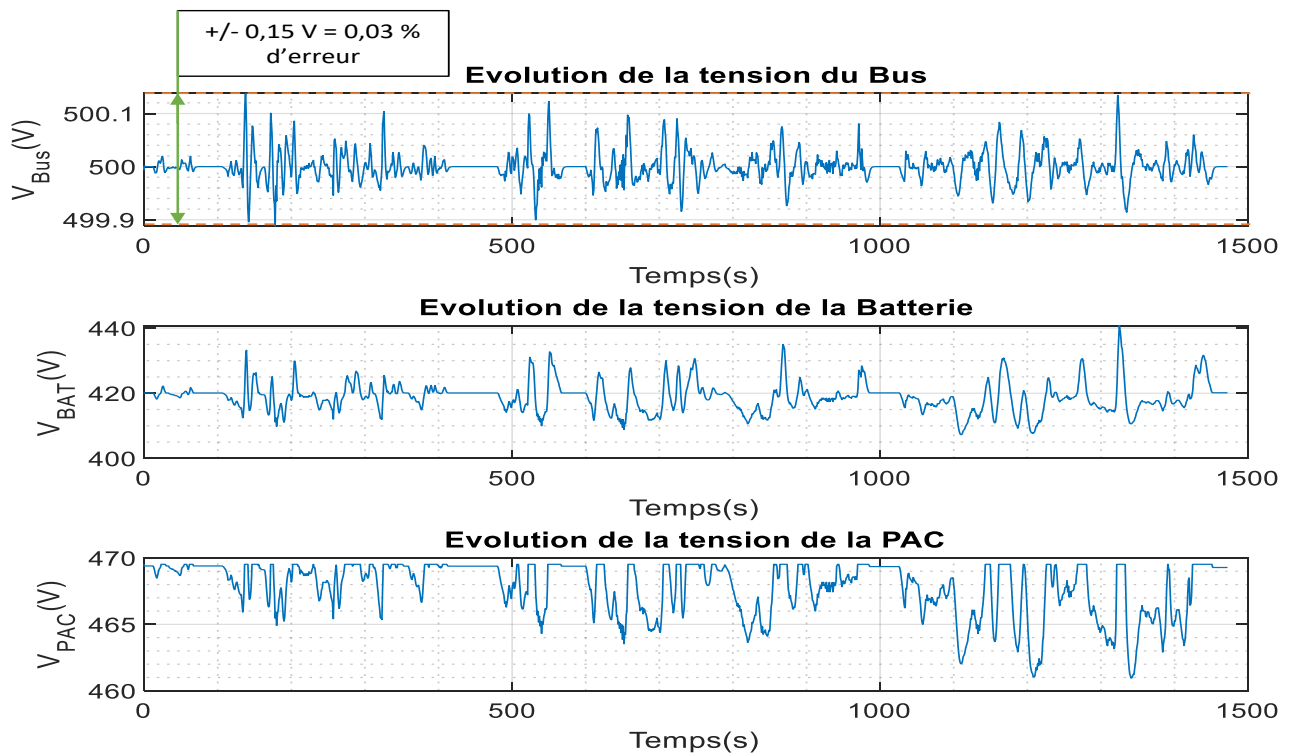
Figure 5-21 Evolution des tensions de l'architecture (rural/classique)
