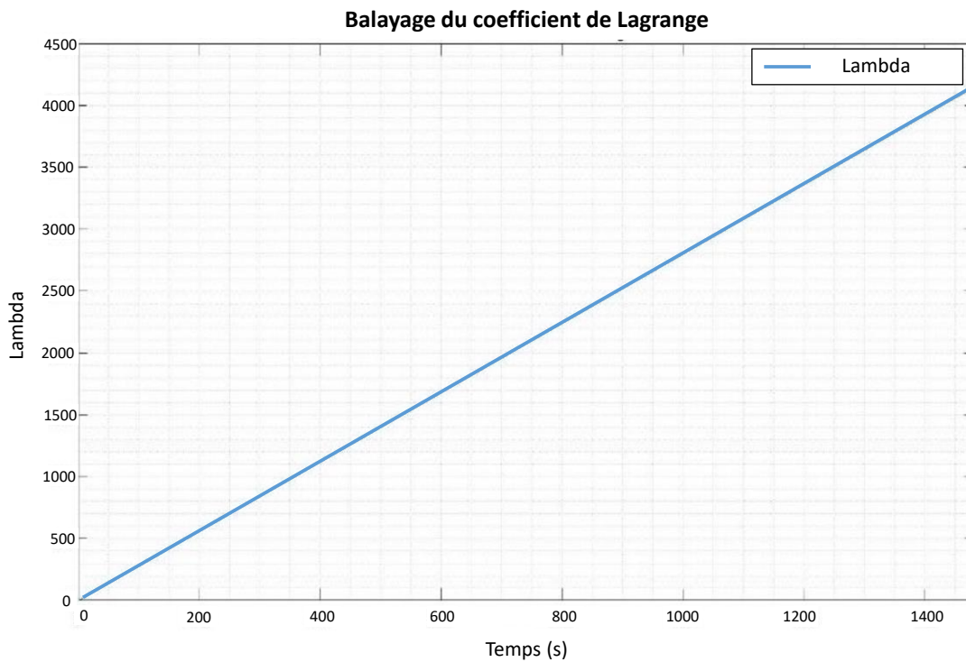
Figure 5-11 Balayage des coefficients de Lagrange ( \lambda ) pour un cycle autoroutier
