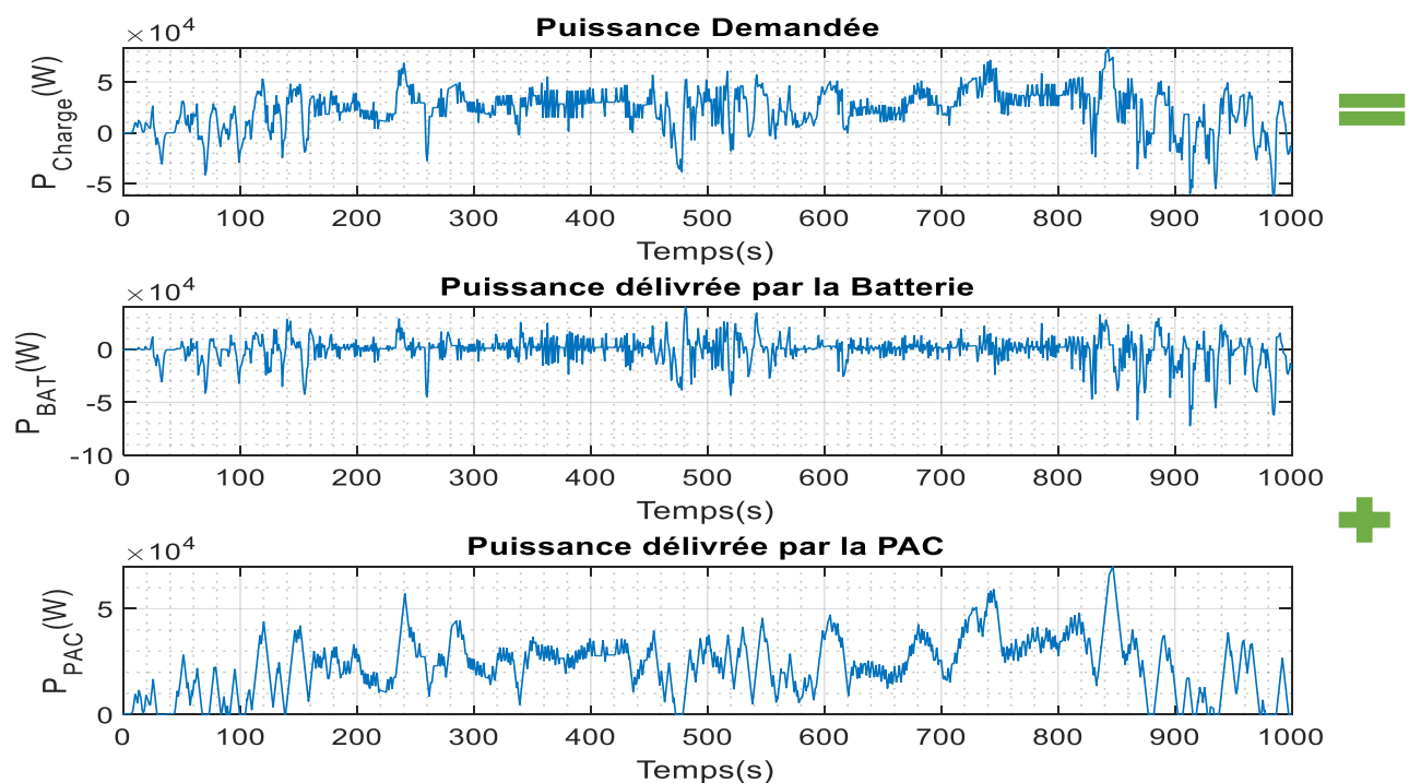
Figure 5-22 Distribution de la puissance (autoroutier/classique)
