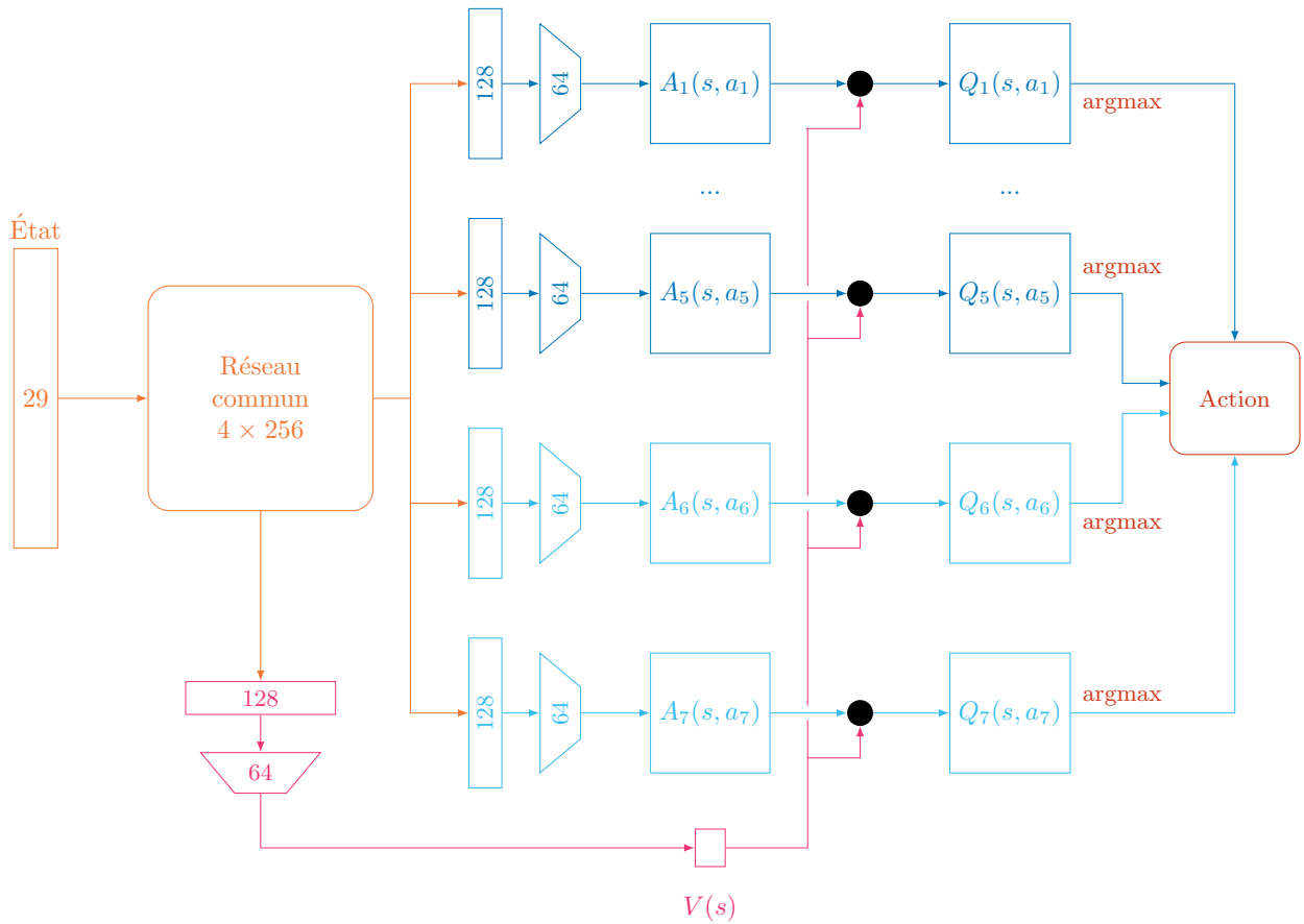
FIGURE 4.7 – Architecture BDQ : le réseau commun (en orange) est partagé entre les huit branches. La partie bleue représente les branches dédiées à l’estimation des Q -values des actions liées aux types. La partie cyan traite les actions relatives à la gestion de l’énergie. La branche en magenta calcule la state -value. À la fin, la sélection des meilleures actions de chaque branche permet de former l’action finale.
