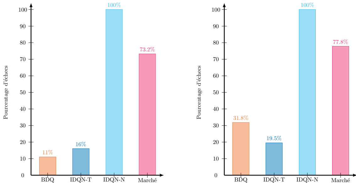
FIGURE 4.13 – Taux d'échecs de la mission pour le jeu n°2 (graphique de gauche) et n°3 (graphique de droite) pour une capacité initiale de batterie de 6500.
