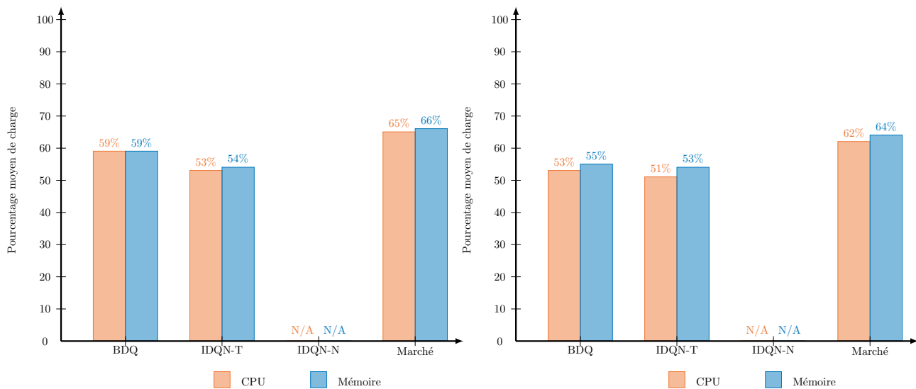
FIGURE 4.16 – Niveaux moyens de CPU (orange) et de mémoire (bleue) pour chaque approche lors d'une mission utilisant le jeu de tâches n°2 (graphique de gauche) et n°3 (graphique de droite). Échouant à terminer la mission, la solution "IDQN-N" n'offre aucun indice de performance.
