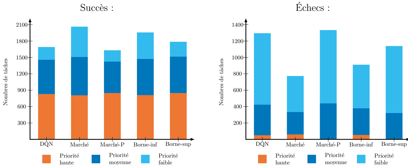
FIGURE 3.6 – Le graphique de gauche présente le nombre de tâches complétées selon leur niveau de priorité par chaque solution et celui de droite, le nombre de tâches échouées.
