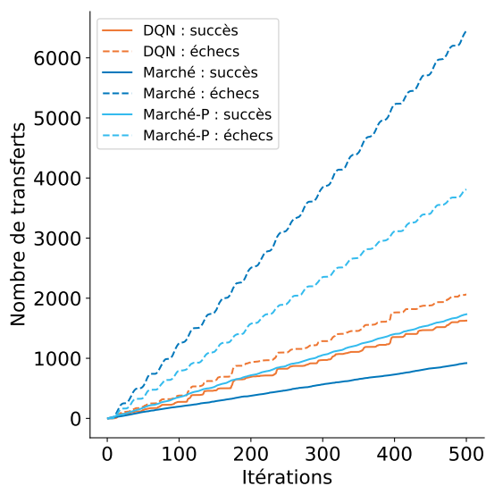
FIGURE 3.9 – Nombres cumulés de succès et d'échecs de transfert sans limitation de portée au cours des 500 itérations pour chaque solution distribuée.
