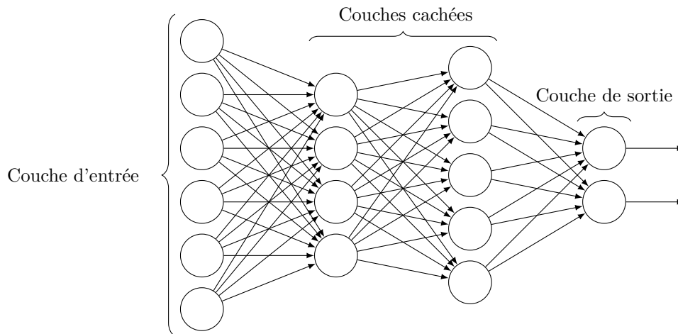
FIGURE 1.5 – Exemple de réseau de neurones artificiels feed-forward composé d’une couche d’entrée de sept neurones, de deux couches cachées de respectivement quatre et cinq neurones et d’une couche de sortie de deux neurones. Toutes les couches sont de type fully connected .
