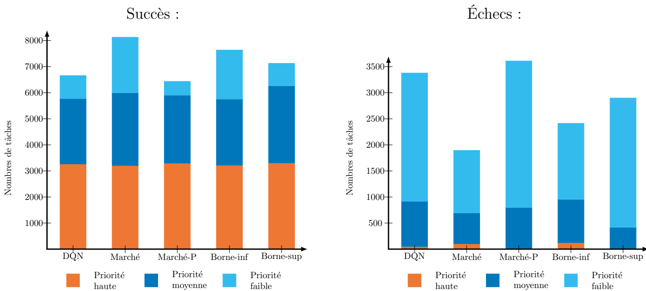
FIGURE 3.11 – Le graphique de gauche présente le nombre de tâches complétées par chaque solution utilisant 20 robots selon leur niveau de priorité. Celui de droite représente le nombre de tâches échouées.
