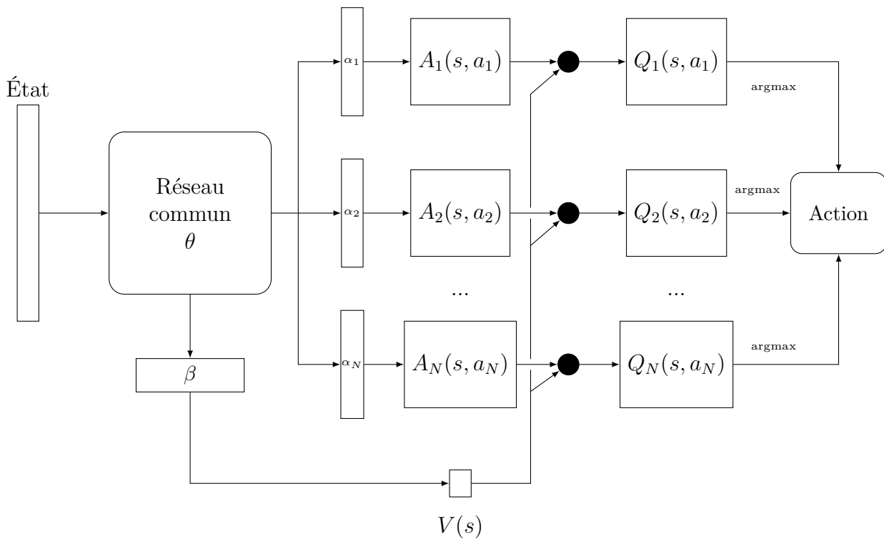
FIGURE 2.6 – Architecture BDQ : nous retrouvons le réseau partagé du 3DQN duquel N + 1 branches émergent. N branches calculent chacune les action-advantage d'une dimension de l'espace d'action pendant qu'une branche estime la state-value commune à tout le réseau. Une agrégation est ensuite réalisée entre chaque branche action-advantage et la branche de state-value afin de produire les Q-values de chaque dimension de l'espace d'action. L'action finale est ensuite obtenue par combinaison des meilleures sous-actions.
