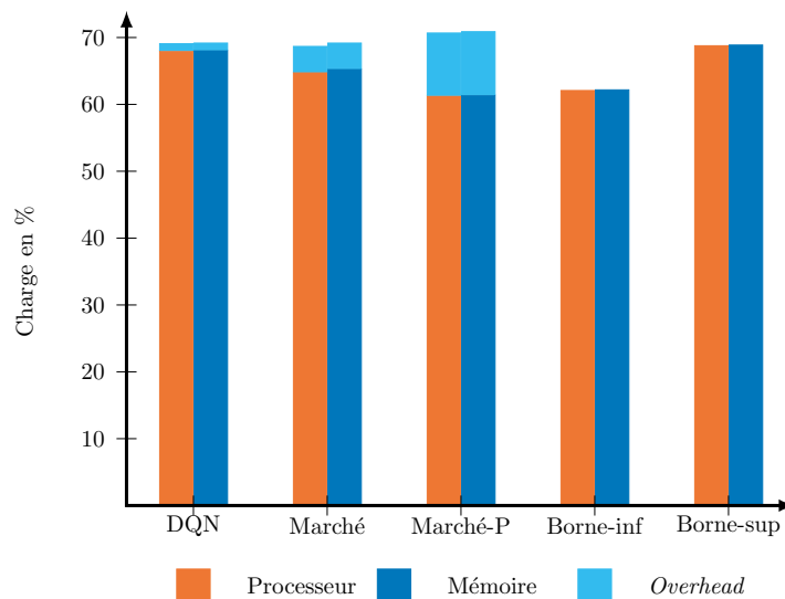
FIGURE 3.7 – Taux d'utilisation moyen des ressources calculatoires de chaque robot en fonction de la solution utilisée. La partie colorée en cyan représente l'overhead généré par l'utilisation du mécanisme de transfert.
