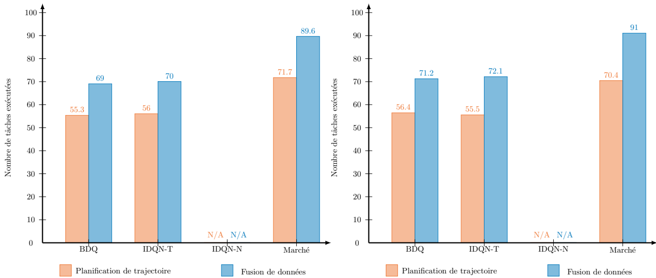
FIGURE 4.20 – Nombre de tâches non-essentiels exécutées par chaque solution pour les jeux de tâches n°2 (graphique de gauche) et n°3 (graphique de droite) : la partie orange représente le type planification de trajectoire et la bleue décrit le type fusion de données
