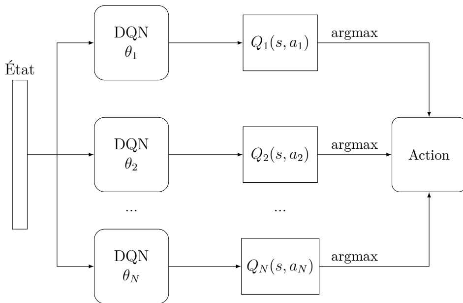
FIGURE 2.5 – Schéma de N DQN indépendants (IDQN) disposés en parallèle où chaque agent (DQN) prédit indépendamment des autres, les Q -values relatives à sa dimension. La sélection des meilleures Q -values, pour chaque dimension à l'aide de l'opérateur argmax, forme l'action finale.
