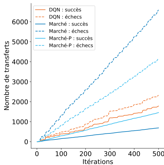
FIGURE 3.8 – Nombres cumulés de succès et d'échecs de transfert au cours des 500 itérations pour chaque solution distribuée.
