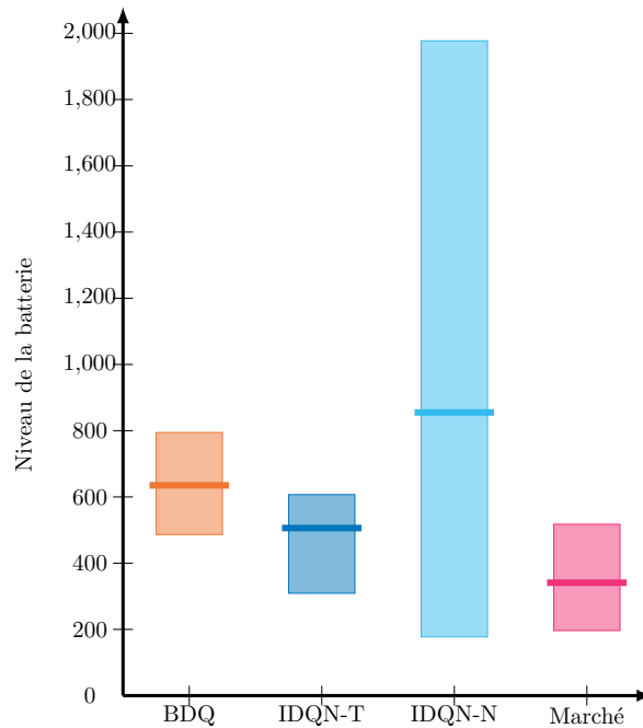
FIGURE 4.21 – Niveaux de batterie à l'issue de la mission pour le jeu de tâches n°1 : les rectangles représentent l'amplitude entre les niveaux de batteries finaux du drone possédant la batterie la plus déchargée et celui qui possède la plus chargée pour les missions terminées avec succès et ceux pour chaque approche. La barre représente le niveau de batterie moyen du système.
