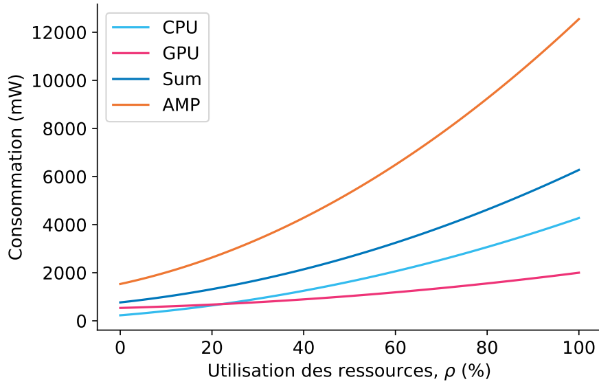
FIGURE 4.3 – Consommation d’un processeur mobile en fonction de l’utilisation. La courbe cyan représente la consommation du CPU. La magenta celle du GPU. Leur agrégation permet d’obtenir la courbe bleue qui peut être amplifiée par un facteur 2 afin de produire la courbe orange proche de la consommation d’une Jetson TX2.
