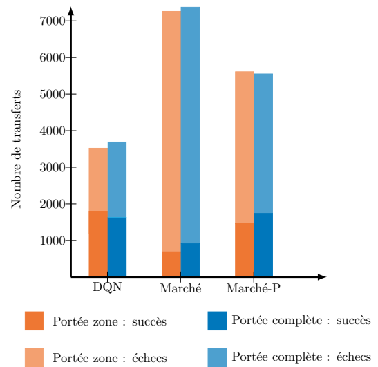
FIGURE 3.10 – Comparaison des succès et échecs des transferts en fonction de la portée du mécanisme.
