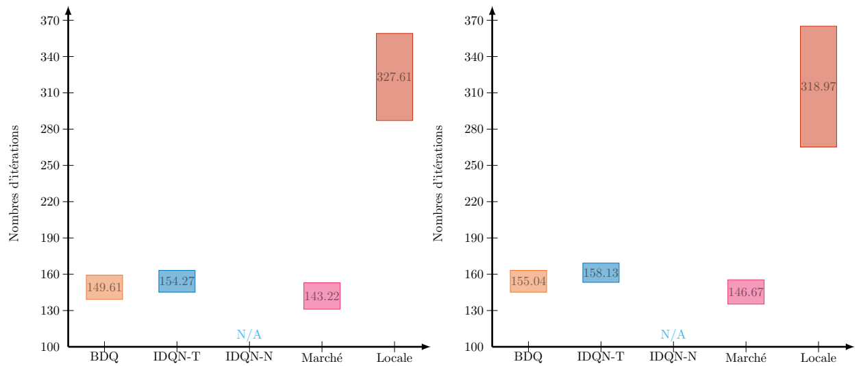
FIGURE 4.11 – Vitesses de résolution pour les jeux n°2 et n°3 : chaque rectangle représente l’amplitude de vitesse entre la mission terminée le plus rapidement et celle terminée le plus lentement pour chaque approche. Les valeurs présentes dans les rectangles indiquent les vitesses moyennes.
