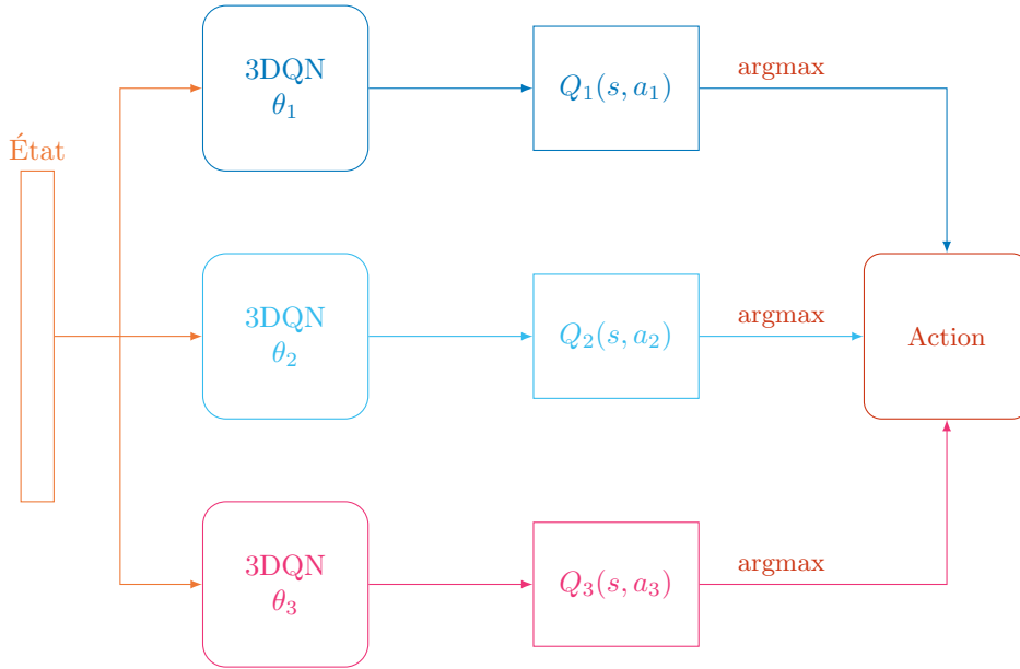
FIGURE 4.9 – Architecture multi-agents travaillée : trois sous-agents indépendants sont déployés. Ils traitent chacun une des parties du problème. La réunion de leurs actions forment l’action finale.
