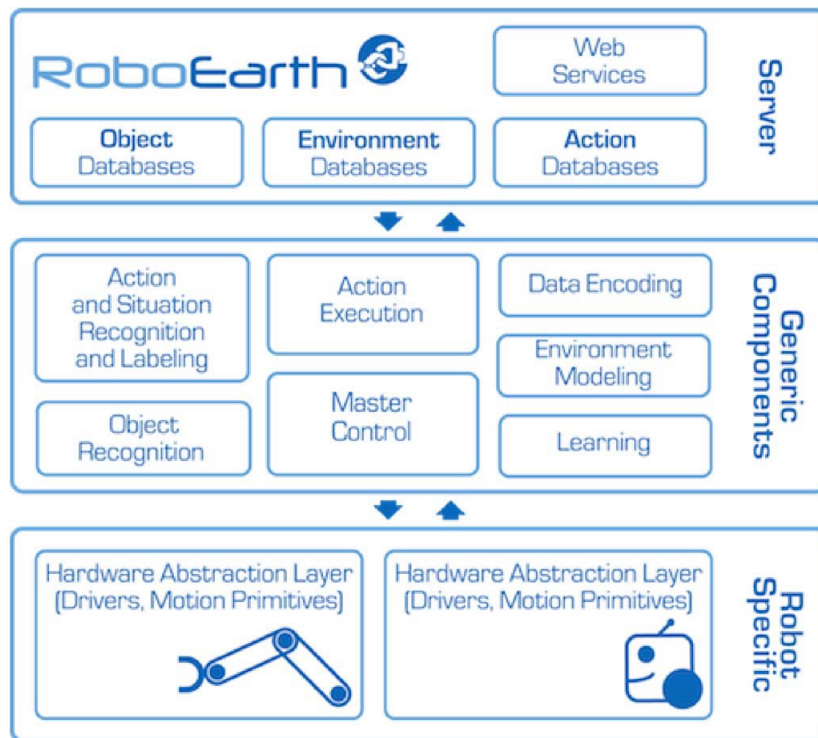
FIGURE 4 – L’architecture du system RoboEarth systems permet aux robots de partager leurs connaissances et d’apprendre les uns des autres [17].
