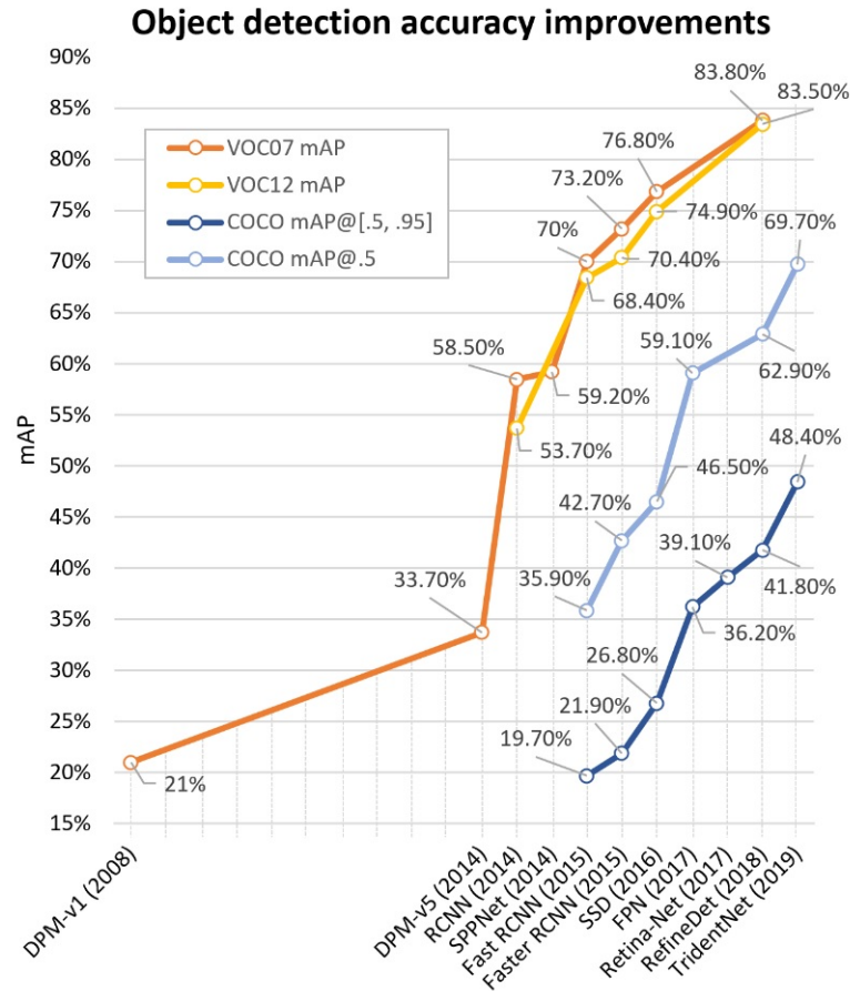
FIGURE 3 – Amélioration de la détection d’objets pour différents algorithmes de vision par ordinateur utilisant des réseaux de neurones [63].
