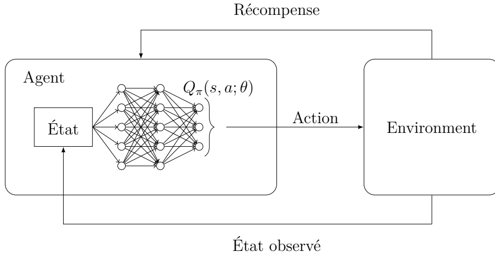
FIGURE 2.2 – Diagramme d’un agent utilisant l’algorithme de Q -Learning avec un DQN comme estimateur. Le réseau de neurones reçoit en entrée l’état observé du système par l’agent et prédit, en sortie, les Q -values relatives à l’état observé.
