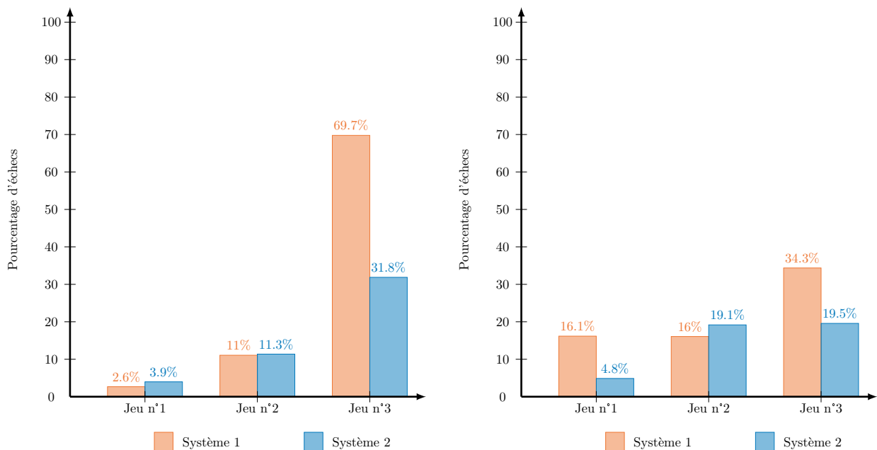
FIGURE 4.23 – Taux de succès en fonction du système de récompense utilisé pour l'approche "BDQ" (graphique de gauche) et "IDQN-T" (graphique de droite).
