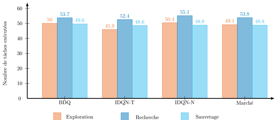
FIGURE 4.17 – Nombre de tâches essentielles exécutées par chaque solution pour une mission utilisant le jeu n°1 : la partie orange représente le type exploration, le type recherche est en bleu et le cyan décrit le type sauvetage
