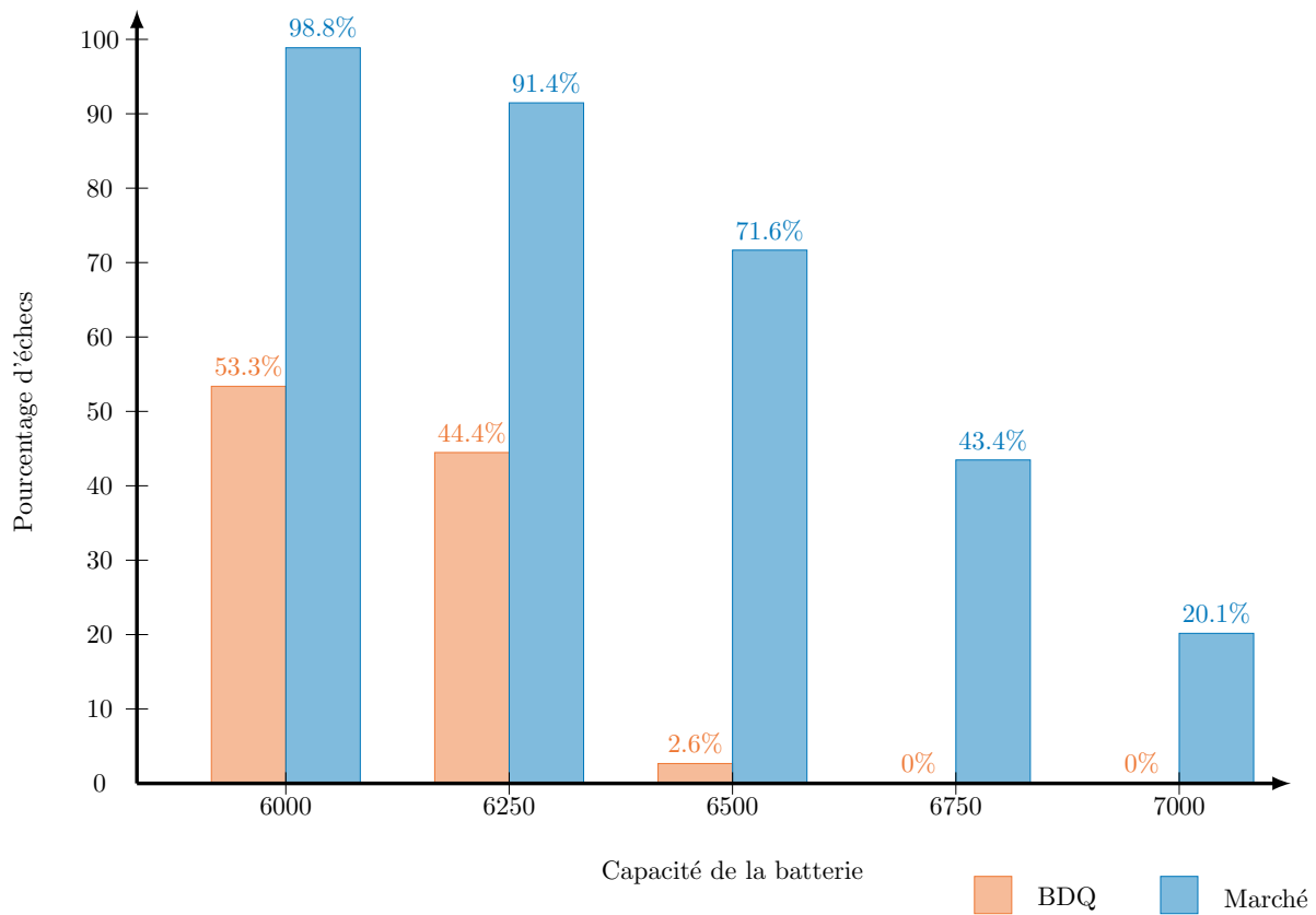
FIGURE 4.14 – Comparaison du taux d’échecs de la mission en fonction de la capacité initiale de la batterie pour les approches BDQ et marché avec le jeu de tâche n°1
