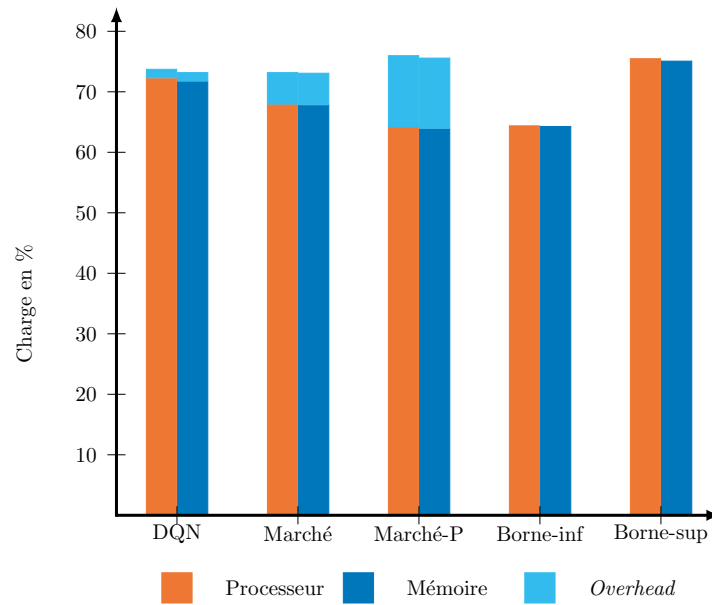
FIGURE 3.12 – Utilisation moyenne des ressources pour un système composé de 20 robots.
