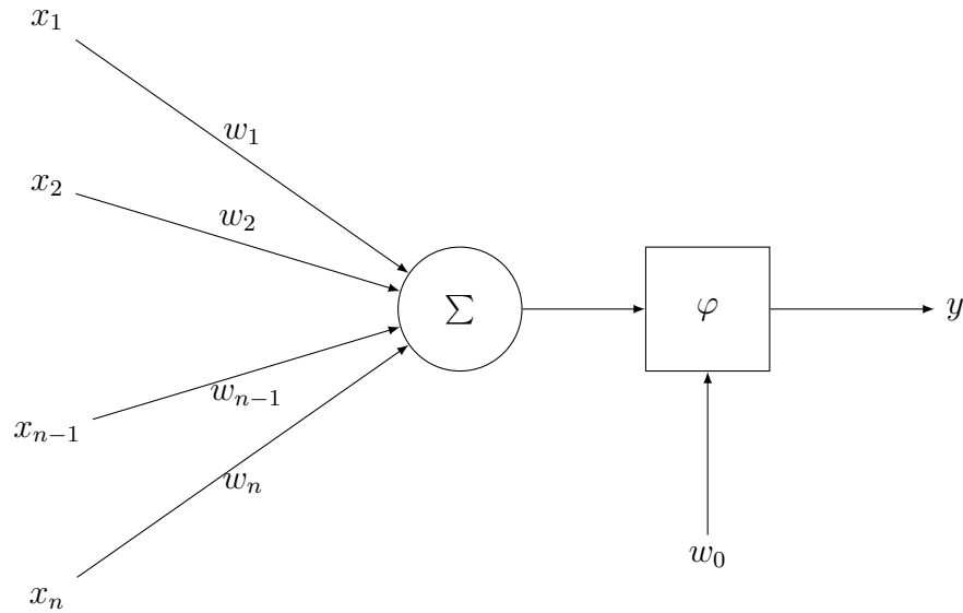
FIGURE 1.4 – Schéma d’un neurone formel : La valeur de sortie du neurone correspond à la somme pondérée des entrées injectée à travers la fonction d’activation après avoir retranché la valeur de seuil.
