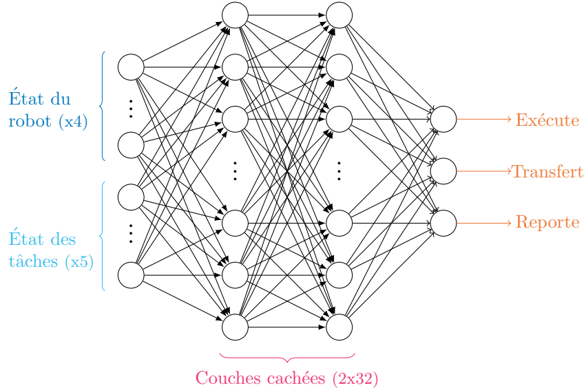
FIGURE 3.4 – L’architecture utilisée est un DQN composé d’une couche d’entrée de neuf neurones dont quatre traduisent l’état du robot et cinq l’état de la tâche sur laquelle portera l’action. Viennent ensuite deux couches cachées totalement connectées composées de 32 neurones. Puis, la couche finale contenant un neurone par action possible. Ces paramètres ont été obtenus par essais successifs afin de parvenir au meilleur ratio performance/taille possible.
