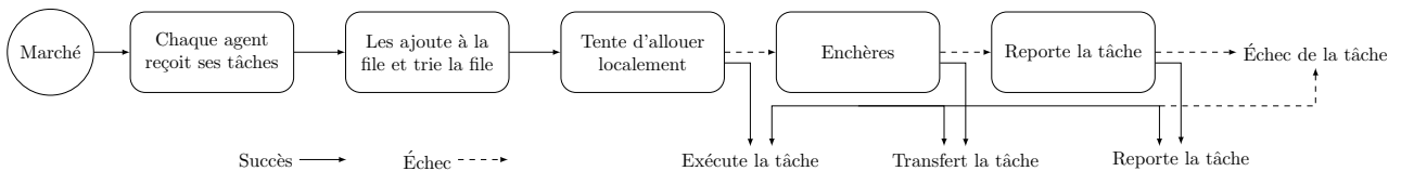
FIGURE 3.2 – Le processus décisionnel de la méthode par marché est fixe. Ainsi cette solution essaiera d’abord d’allouer localement puis en cas d’échec formulera une proposition de transfert et finalement, en cas de nouvel échec reportera, la tâche.
