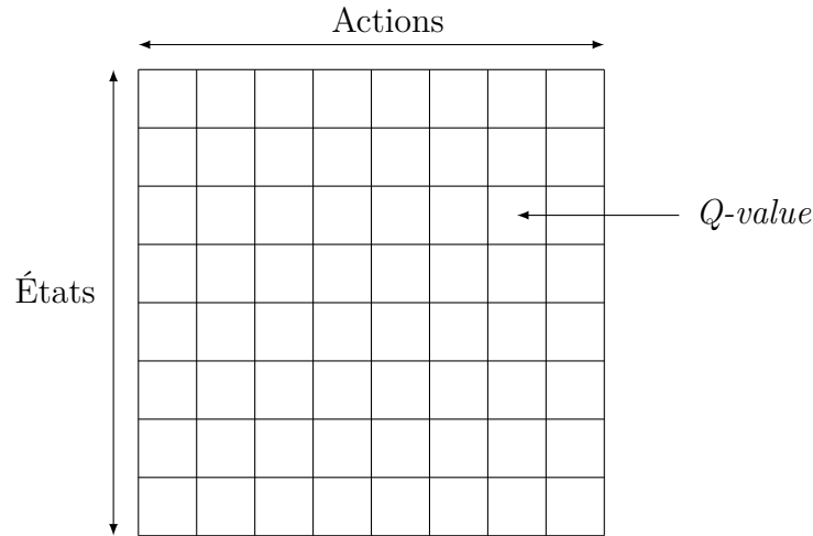
FIGURE 2.1 – Table de Q-Learning : chaque case de la Q-table contient une Q-value pour une action dans un état.
