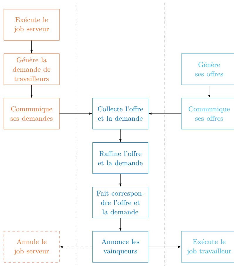
FIGURE 4.6 – Déroulement des enchères : chaque drone commençant une nouvelle tâche (en orange) génère une offre par travailleur potentiel. En parallèle, l'ensemble des drones (en cyan) formulent leurs offres d'achat. L'ensemble des propositions (offre et demande) est collecté par le commissaire-priseur (en bleu) qui conduit les enchères. À la fin, les gagnants exécutent leurs nouveaux jobs de travailleurs et les tâches ne trouvant pas suffisamment de travailleurs sont annulées, leur job serveur s'arrêtant.
