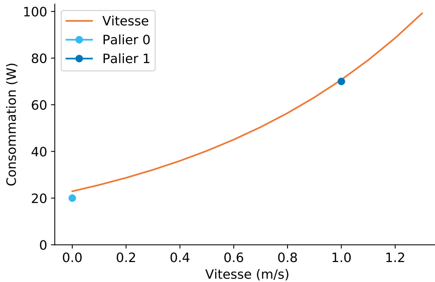
FIGURE 4.5 – Consommation liée à la propulsion en fonction de la vitesse du drone. Les paliers 0 et 1 apparaissent respectivement en cyan et bleu sur le graphique.
