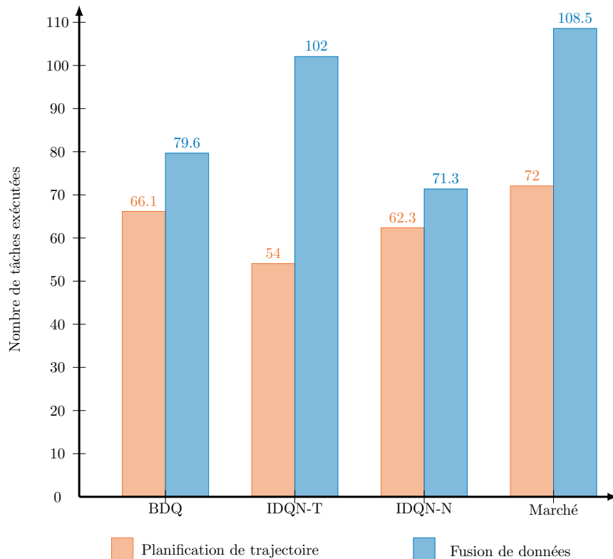
FIGURE 4.19 – Nombre de tâches non essentielles exécutées par chaque solution pour le jeu de tâches n°1 : la partie orange représente le type planification de trajectoire et la bleu décrit le type fusion de données
