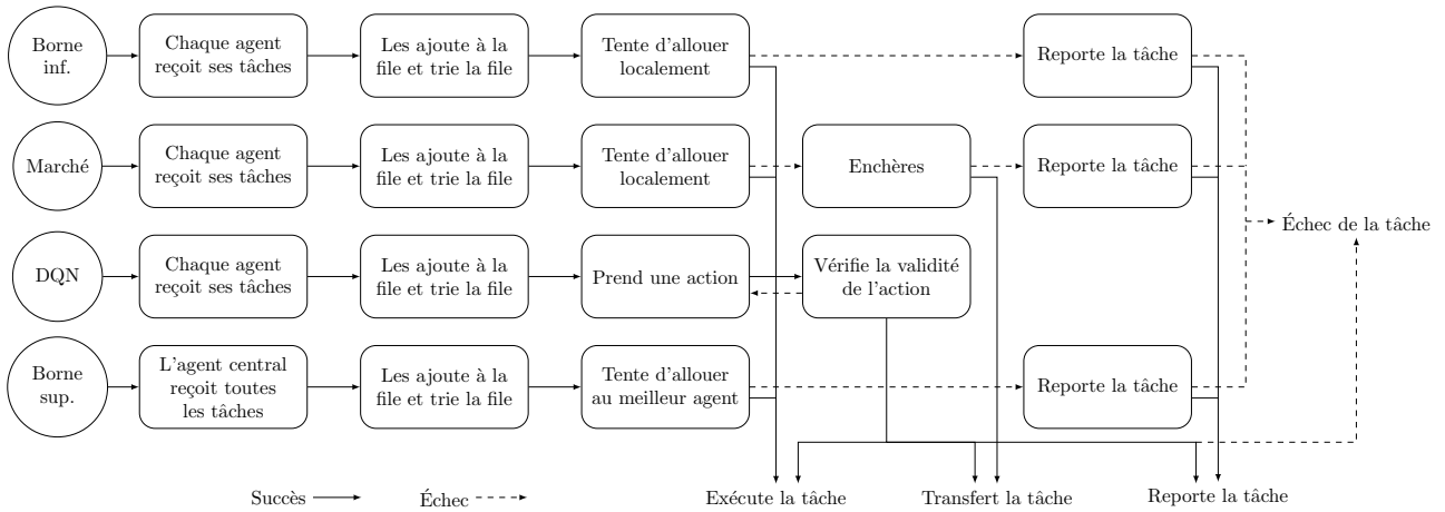
FIGURE 3.5 – Résumé de l'ensemble des processus décisionnels
