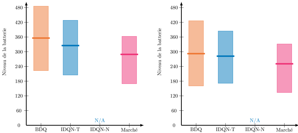
FIGURE 4.22 – Niveaux de batterie à l’issue de la mission pour le jeu de tâches n°2 (graphique de gauche) et n°3 (graphique de droite) : les rectangles représentent l’amplitude entre les niveaux de batteries finaux du drone possédant la batterie la plus déchargée et celui qui possède la plus chargée pour les missions terminées avec succès et ceux pour chaque approche. La barre représente le niveau de batterie moyen du système. Échouant à terminer la mission, la solution "IDQN-N" n’offre aucun indice de performance.
