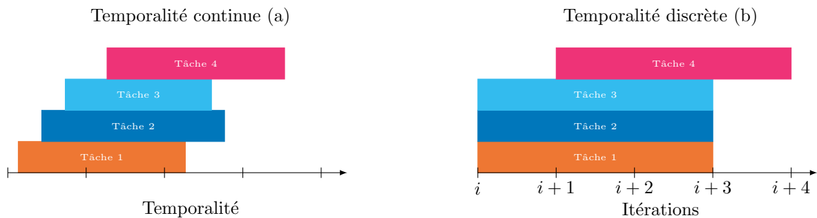
FIGURE 3.1 – Temporalité : la figure de gauche représente une temporalité continue et celle de droite une temporalité discrète. Contrairement à la temporalité continue, le cas discret comporte des tâches possédant un temps d'exécutions identiques (3 cycles) et les tâches n°1,2 et 3 commencent et terminent en même temps. Cette discrétisation implique une standardisation des temps d'exécution et de la simultanéité.
