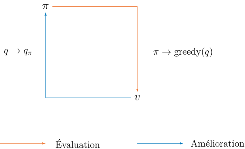
FIGURE 1.3 – GPI : cette fois-ci, l' action-value function interagit policy function jusqu'à l'optimalité.
