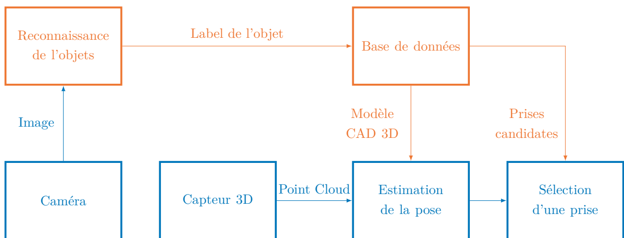
FIGURE 2.12 – Exemple d'utilisation du cloud (orange) pour assister la prise d'un objets par un robot (bleu). L'utilisation du cloud permet de détecter l'objet avec précision permettant de déterminer, à l'aide d'une base de données, les meilleures prises [18].
