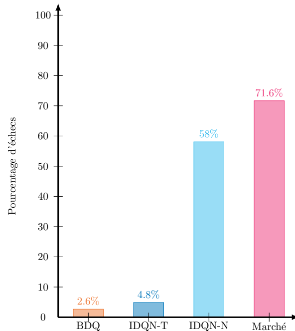
FIGURE 4.12 – Taux d'échecs de la mission pour le jeu n°1 pour une capacité initiale de batterie de 6500
