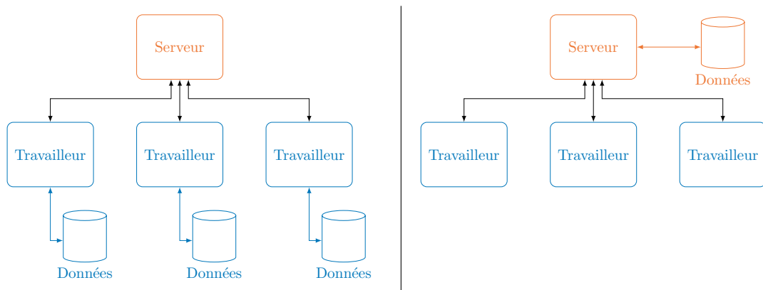
FIGURE 4.1 – Deux paradigmes de distribution : à gauche, les travailleurs possèdent les données nécessaires à l'exécution de la tâche alors qu'à droite le serveur doit transmettre les données les données aux travailleurs.
