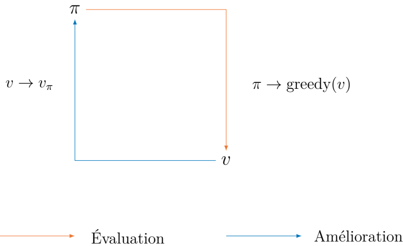
FIGURE 1.2 – GPI : Les value functions et policy functions interagissent jusqu'à être optimales et donc consistantes l'une envers l'autre.
