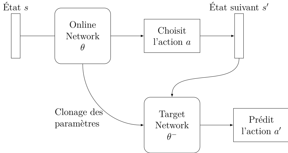
FIGURE 2.3 – Schéma d'un réseau utilisant un target network : le calcul de la cible s'effectue selon le choix d'action de l' online network , mais avec les paramètres du target network
