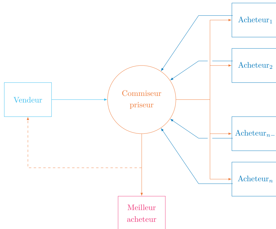
FIGURE 2.9 – Diagramme : le vendeur (cyan) transmet son offre au commissaire preneur (orange) qui la communique aux participants (bleu). Ces derniers formulent chacun une offre d’achat. Le commissaire preneur attribue alors l’objet de la vente au meilleur offrant (magenta) si la valeur de l’offre dépasse le prix de réserve
