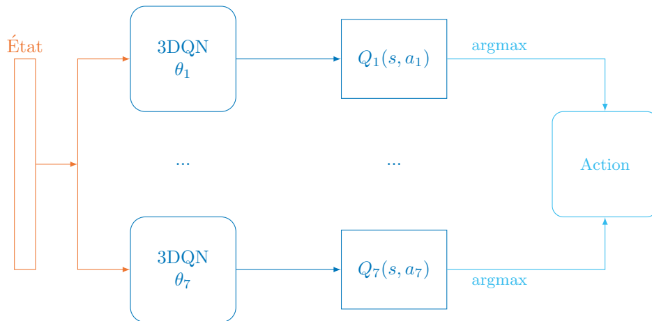
FIGURE 4.8 – Architecture multi-agents naïve : sept sous-agents sont déployés. Ils ne possèdent en commun que le signal d'état transmis par l'environnement. La combinaison des actions de chaque sous-agent permet d'obtenir l'action finale sur le système.
