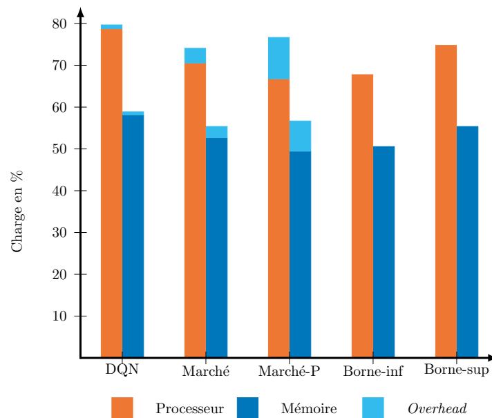
FIGURE 3.14 – Taux moyen d’utilisation des ressources lorsque le second jeu de tâches est utilisé.
