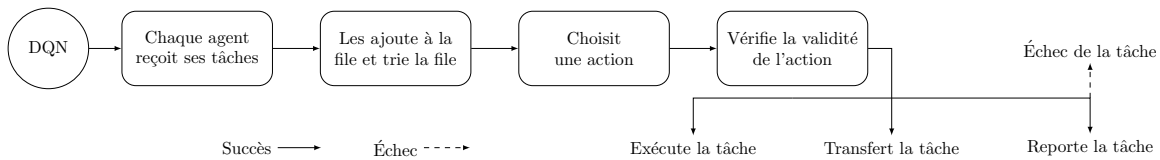
FIGURE 3.3 – Le processus décisionnel de l'approche par renforcement dépend de la politique apprise. Aucune restriction autre que la validité d'une action n'est imposée à cette approche
