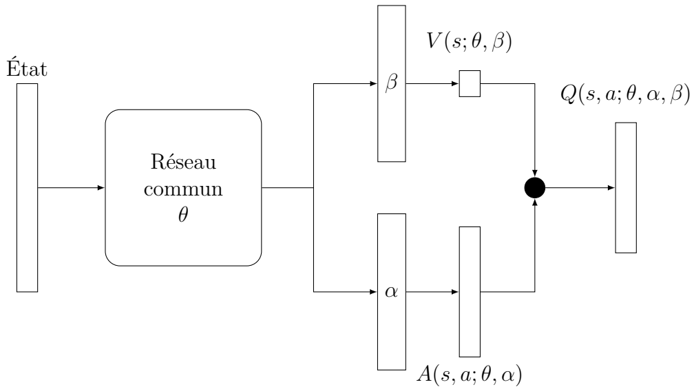
FIGURE 2.4 – Schéma d’une architecture 3DQN : Cette architecture est constituée de quatre éléments distincts. Le premier est un réseau partagé servant à l’extraction des caractéristiques communes. De ce réseau émergent deux branches. La première de paramètre \beta calcule un unique scalaire, le state value . La deuxième de paramètre \alpha produit un vecteur contenant l’ avantage de chaque action. Le dernier élément est la couche d’agrégation permettant l’estimation des Q-values
