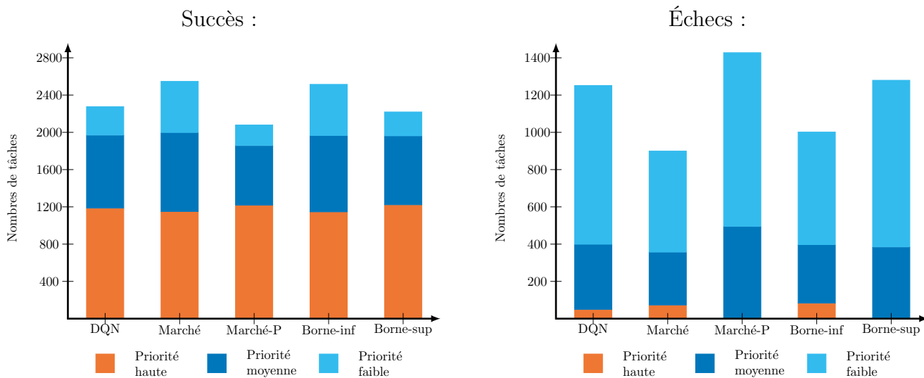
FIGURE 3.13 – Le graphique de gauche présente le nombre de tâches complétées par chaque solution selon leur niveau de priorité lors de l'utilisation d'un jeu de tâches déséquilibré. Celui de droite représente le nombre de tâches échouées.
