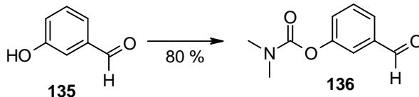
Schéma 31. Synthèse du précurseur rivastigmine.
