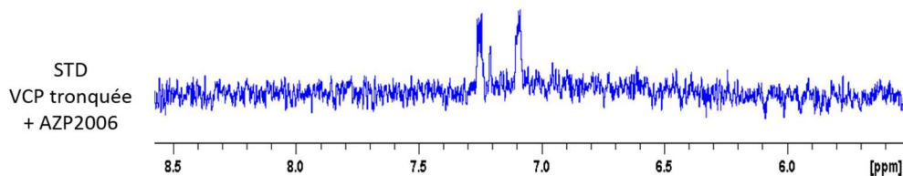
Figure 101. Zoom de la partie aromatique du spectre STD de la protéine tronquée avec l'AZP2006. (AZP2006 200 \mu M, p97/VCP tronquée 5 \mu M)
