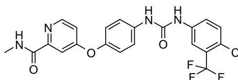
Figure 70. Sorafenib. 235
