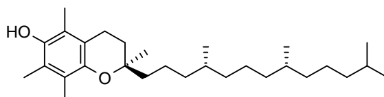
Figure 28. Vitamine E, un antioxydant.
