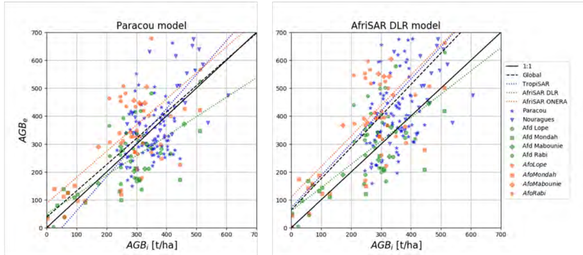
FIGURE 4.66 – Graphes de comparaison entre les biomasses estimées, AGB_e , et les mesures terrain, AGB_i dans le cas d'une inversion directe des cartes d'indicateurs polarimétriques t^0 à partir des modèles de régression de TropiSAR (à gauche) et du DLR (à droite) détaillés dans le tableau 4.19 pour l'intégralité des données disponibles. Les résultats statistiques associés sont regroupés dans les tableaux 4.22 et 4.23.
