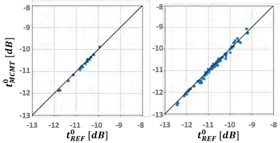
FIGURE 3.6 – Estimation des t_{MCMT}^0 = f(t_{REF}^0) obtenus pour les données PolSAR en bande P du site test de Paracou, acquises avec une bande passante de 125 MHz. La résolution des données après application des filtres REF et MCMT est équivalente à 5 m. Sur la partie gauche de la figure, 15 ROI de 6.25 ha sont considérées ainsi qu'un ROI de 25 ha. Sur la partie droite, 84 ROI de 1 ha sont considérées.
