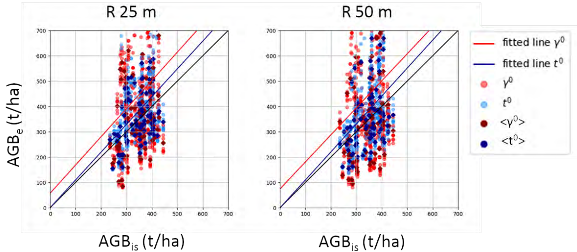
FIGURE 4.17 – Graphes de comparaison entre les biomasses estimées, AGB_e , et les mesures in situ , AGB_i . On compare les biomasses extraites après une inversion directe des cartes d'indicateurs polarimétriques \gamma^0 (en rouge) et t^0 (en bleu). Pour l'inversion directe, nous avons utilisé les paramètres du modèle issu du scénario B. Les résultats statistiques associés sont regroupés dans le tableau 4.6
