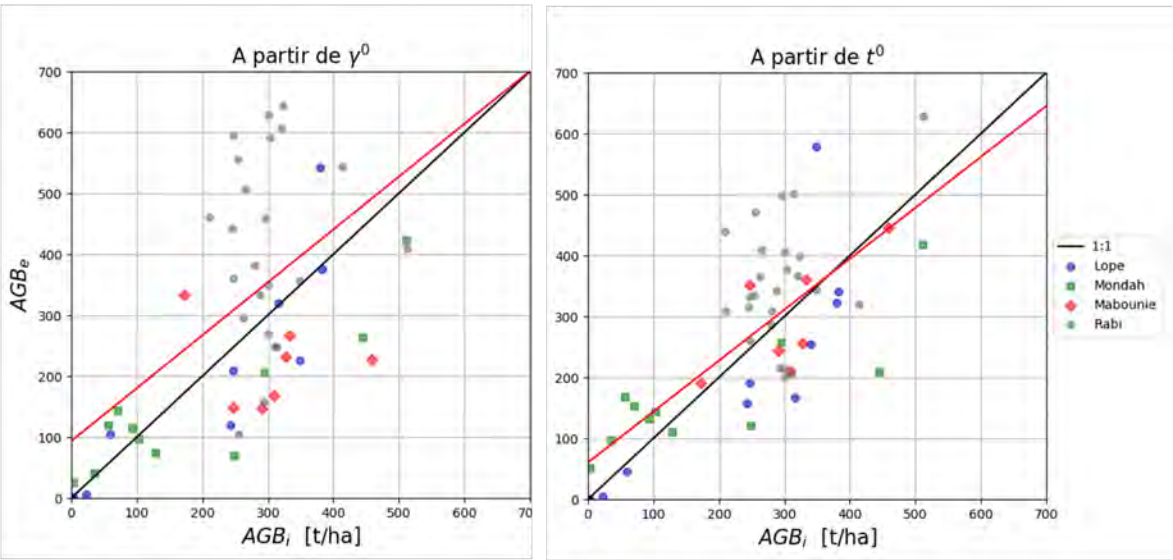
FIGURE 4.42 – Graphes de comparaison entre les biomasses estimées, AGB_e , et les mesures terrain, AGB_i dans le cas d’une inversion directe des cartes d’indicateurs polarimétriques \gamma^0 (à gauche) et t^0 (à droite) à partir des modèles de régression détaillés dans le tableau 4.12 pour les données de la campagne AfriSAR DLR. Les résultats statistiques associés sont regroupés dans le tableau 4.13.
