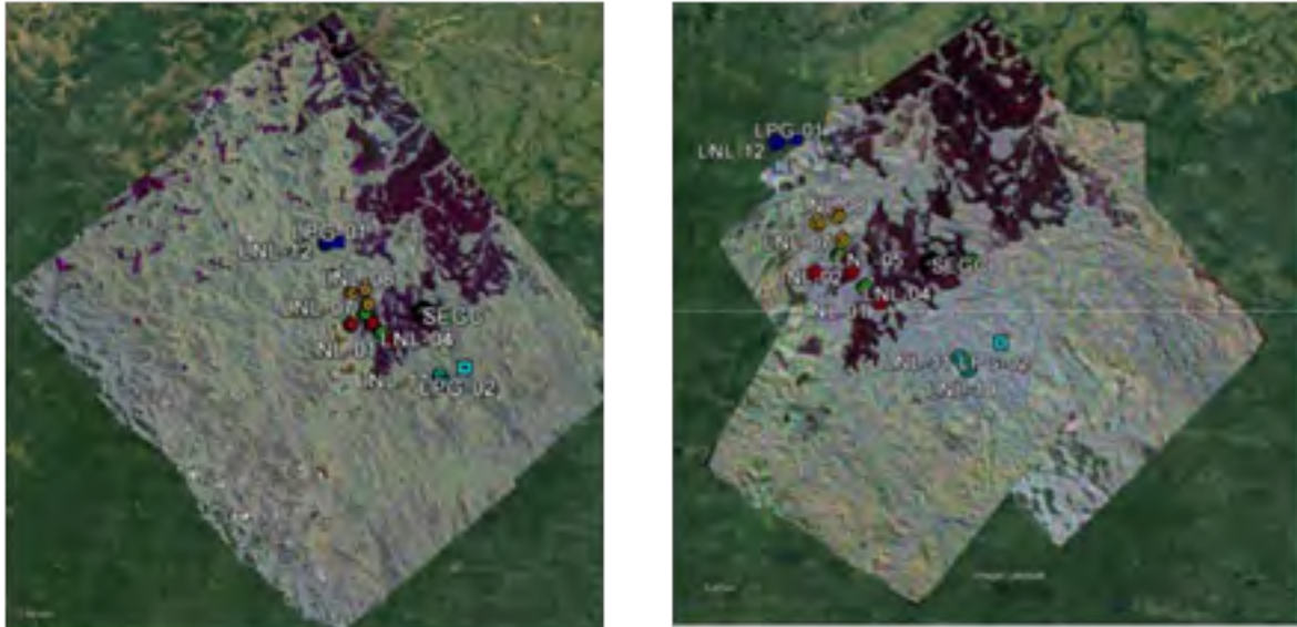
FIGURE 2.6 – Superposition des images bande P acquises sur le site de La Lopé en fausses couleurs (Rouge : HH, Vert : HV, Bleu : VV) avec une localisation des ROI. Axe azimuthal horizontal et axe vertical en range. Extrait de [11].
