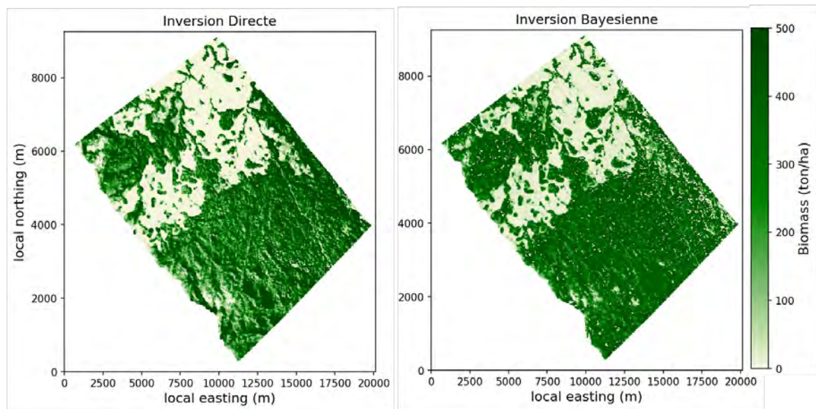
FIGURE 4.28 – Cartes de biomasse à 25 m de résolution, estimées pour le site de La Lopé à partir de la carte de \gamma^0 calculée pour les données acquises pendant la campagne AfriSAR DLR. Les paramètres du modèle d'inversion sont dans le tableau 4.12. La carte de gauche a été obtenue après une inversion directe, celle de droite après une inversion bayésienne.
