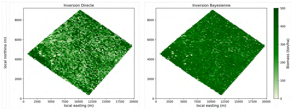
FIGURE 4.39 – Cartes de biomasse à 100 m de résolution, estimées pour le site de Rabi à partir de la carte de \gamma^0 calculée pour les données acquises pendant la campagne AfriSAR DLR. Les paramètres du modèle d'inversion sont dans le tableau 4.12. La carte de gauche a été obtenue après une inversion directe, celle de droite après une inversion bayésienne.
