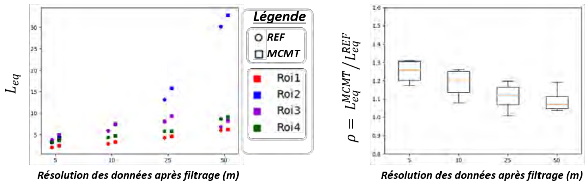
FIGURE 3.7 – Impact de la résolution de filtrage sur le nombre équivalent de vues L_{eq} (à gauche) et sur le rapport \rho = L_{eq}^{NCI} / L_{eq}^{BOX} (à droite) pour les quatre ROI représentées sur la figure 3.3
