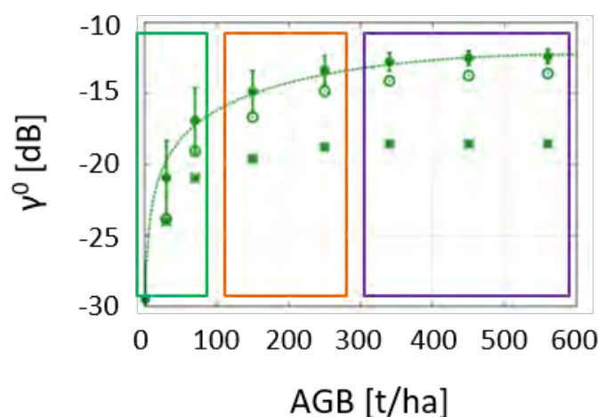
FIGURE 1.8 – Simulation du coefficient de rétrodiffusion HV en fonction de la biomasse pour mettre en valeur les contributions des 2 principaux mécanismes de rétrodiffusion. Les cercles vides montrent les interactions directes de HV avec la végétation, les losanges barrés témoignent des interactions en double rebond avec le sol. La courbe en pointillés représente le total des contributions de diffusion. Le cadre vert correspond au domaine élastique ( AGB < 100 t/ha), le cadre orange au domaine de transition ( AGB \in [100, 300] t/ha) et le cadre violet au domaine de quasi-saturation ( AGB > 300 t/ha). Extrait de [59].
