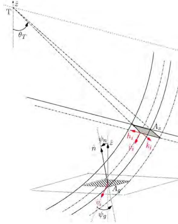
FIGURE 3.8 – Schématisation de la géométrie oblique d'un capteur SAR en fonction de l'angle d'élévation \theta_T , des surfaces inclinées et surfaces au sol A_s et A_g , de la base de transmission (\hat{k}_i, \hat{h}_i, \hat{v}_i) , des vecteurs vertical et normal \hat{z}, \hat{n} , des angles de pente \psi_n et \psi_g ainsi que du volume d'interception lié à la résolution au sol de la cellule d'acquisition. Extrait de [13].
