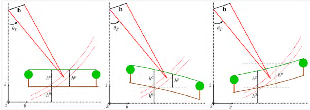
FIGURE 1.9 – Correction de l'indicateur h^v à partir de la topographie locale pour obtenir h^c . Extrait de [8].
