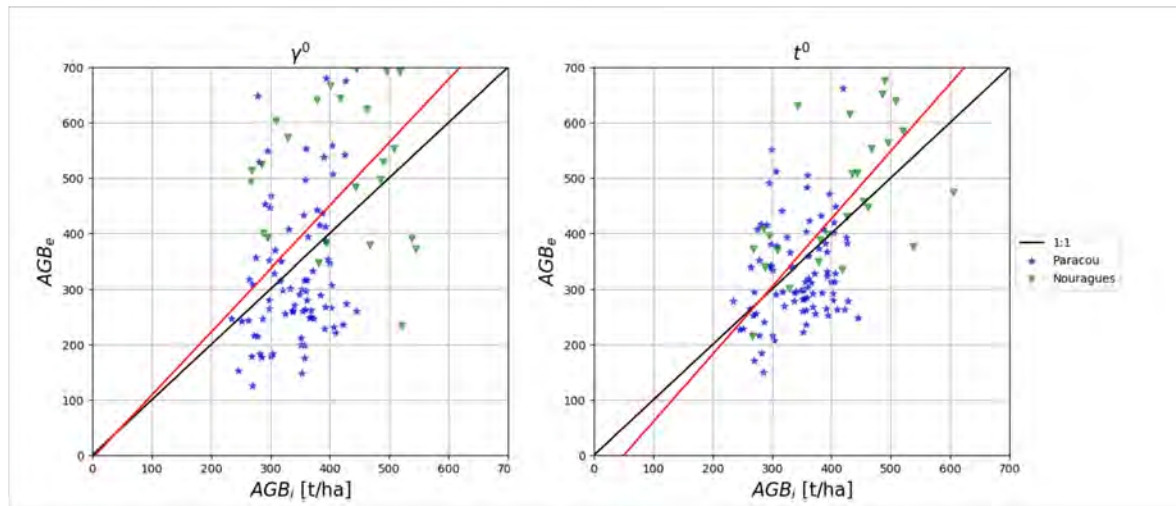
FIGURE 4.25 – Graphes de comparaison entre les biomasses estimées, AGB_e , et les mesures terrain, AGB_i , dans le cas d'une inversion directe des cartes d'indicateurs polarimétriques \gamma^0 (à gauche) et t^0 (à droite) à partir des modèles de régression détaillés dans le tableau 4.9 pour les données de la campagne TropiSAR. Les résultats statistiques associés sont regroupés dans le tableau 4.10.
