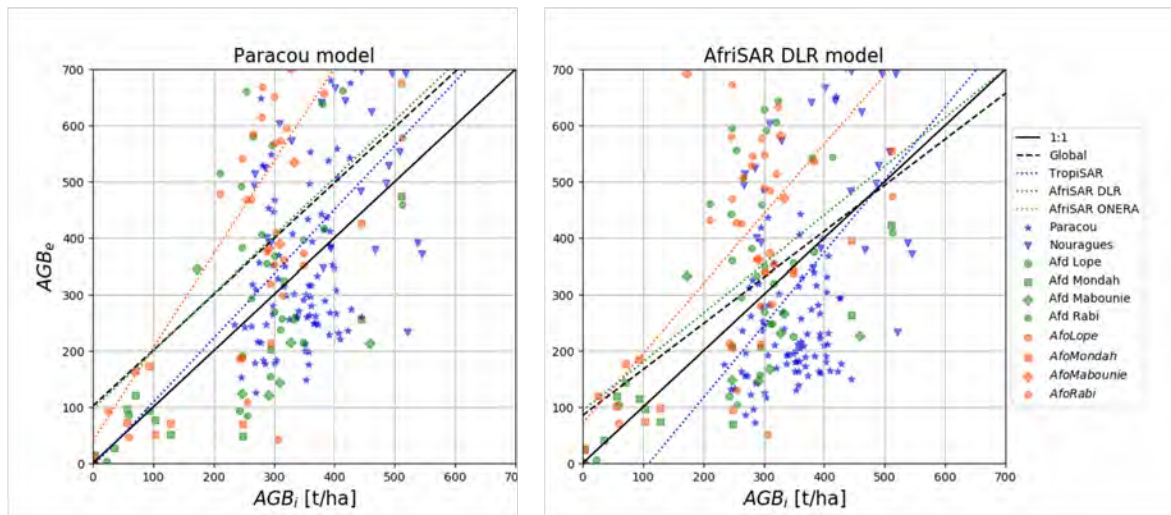
FIGURE 4.65 – Graphes de comparaison entre les biomasses estimées, AGB_e , et les mesures terrain, AGB_i dans le cas d'une inversion directe des cartes d'indicateurs polarimétriques \gamma^0 à partir des modèles de régression de TropiSAR (à gauche) et du DLR (à droite) détaillés dans le tableau 4.18 pour l'intégralité des données disponibles. Les résultats statistiques associés sont regroupés dans les tableaux 4.20 et 4.21.
