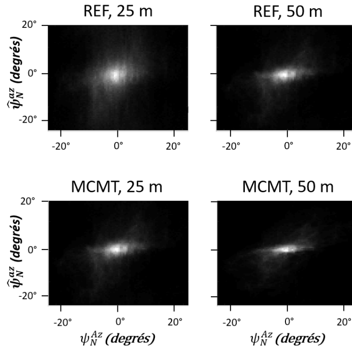
FIGURE 3.11 – Histogrammes 2D représentant la corrélation des pentes azimutales issues du DEM SRTM ( \psi_N^{Az} ) en fonction des pentes azimutales estimées à partir des données PolSAR ( \hat{\psi}_N^{az} ). Le calcul de la corrélation est réalisé pour la zone encadrée en rouge sur la figure 3.9. La première colonne correspond aux résultats obtenus après application du filtre REF, la deuxième colonne à ceux obtenus avec le filtre MCMT. Sur la première ligne, résultats obtenus avec une résolution de 25 m à la sortie du filtre, sur la deuxième ligne, résultats obtenus avec une résolution de 50 m à la sortie du filtre.
