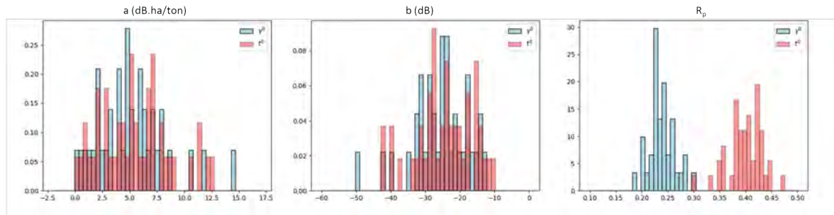
FIGURE 4.11 – Histogrammes des paramètres de régression issus de l'estimation du \gamma^0 (en bleu) et du t^0 (en rose) calculés pour chaque itération du scénario C.
