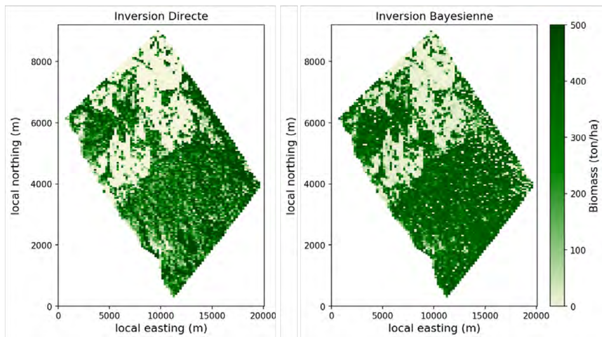
FIGURE 4.29 – Cartes de biomasse à 100 m de résolution, estimées pour le site de La Lopé à partir de la carte de \gamma^0 calculée pour les données acquises pendant la campagne AfriSAR DLR. Les paramètres du modèle d'inversion sont dans le tableau 4.12. La carte de gauche a été obtenue après une inversion directe, celle de droite après une inversion bayésienne.
