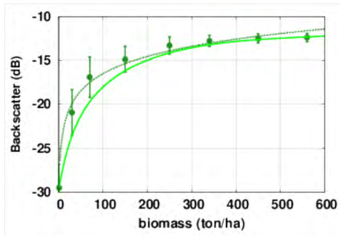
FIGURE 4.2 – Coefficients de rétrodiffusion simulés exprimés en fonction de la biomasse forestière pour deux modèles de régression polylog d'ordre 1. Extrait de [1].
