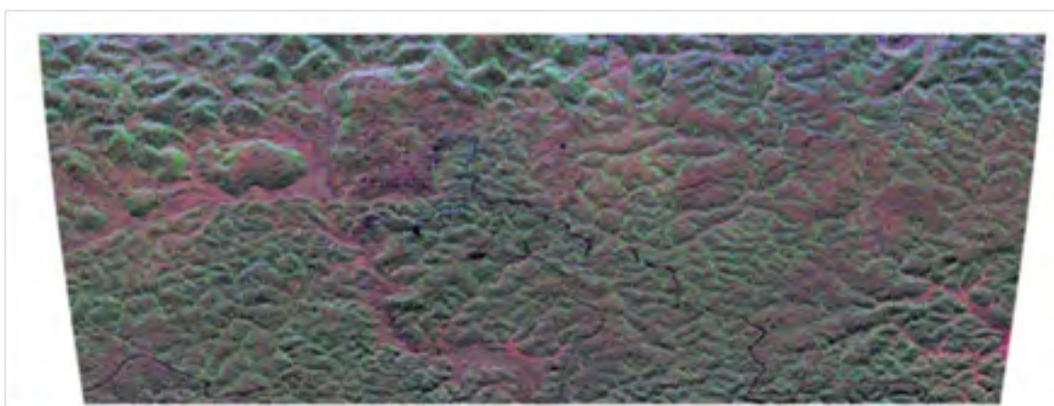
FIGURE 2.8 – Superposition des images bande P acquises sur le site de Mabounie en fausses couleurs (Rouge : HH, Vert : HV, Bleu : VV). Axe azimutal vertical et axe horizontal en range. Extrait de [11].
