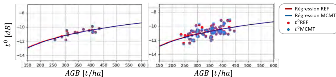
FIGURE 3.5 – Estimation de t^0 en fonction de la biomasse forestière obtenue pour les données PolSAR en bande P du site test de Paracou, acquises avec une bande passante de 125 MHz. La résolution des données après application des filtres REF et MCMT est équivalente à 5 m. Sur la partie gauche de la figure, 15 ROI de 6.25 ha sont considérées ainsi qu’une ROI de 25 ha. Sur la partie droite, 84 ROI de 1 ha sont considérées.
