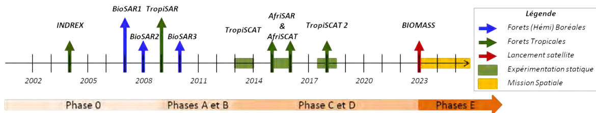
FIGURE 2.1 – Organisation chronologique des campagnes aéroportées et des expérimentations en bande P réalisées dans le cadre de la mission BIOMASS.
