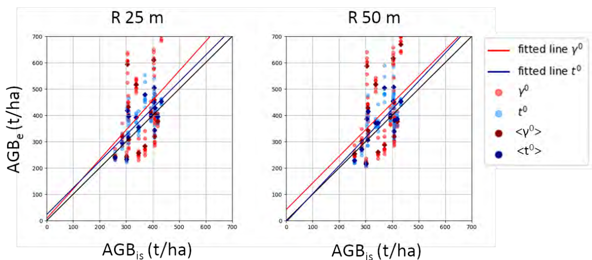
FIGURE 4.16 – Graphes de comparaison entre les biomasses estimées \text{AGB}_e et les mesures terrain \text{AGB}_i . On compare les biomasses extraites après une inversion bayésienne des cartes d'indicateurs polarimétriques \gamma^0 (en rouge) et t^0 (en bleu). Pour l'inversion directe nous avons utilisé les paramètres du modèle issu du scénario A. Les résultats statistiques associés sont regroupés dans le tableau 4.5
