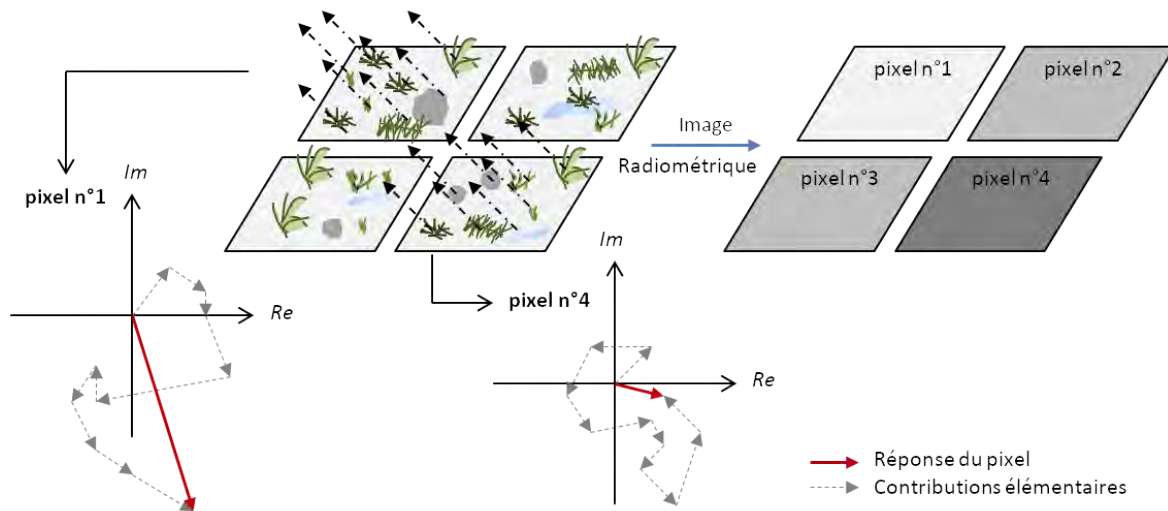
FIGURE 3.1 – (À gauche) origine physique du speckle : effets de la nature cohérente des illuminations radar avec la combinaison des contributions élémentaires dans chaque pixel. (À droite) Distribution radiométrique de l'image SAR résultante. Extrait de [2].
