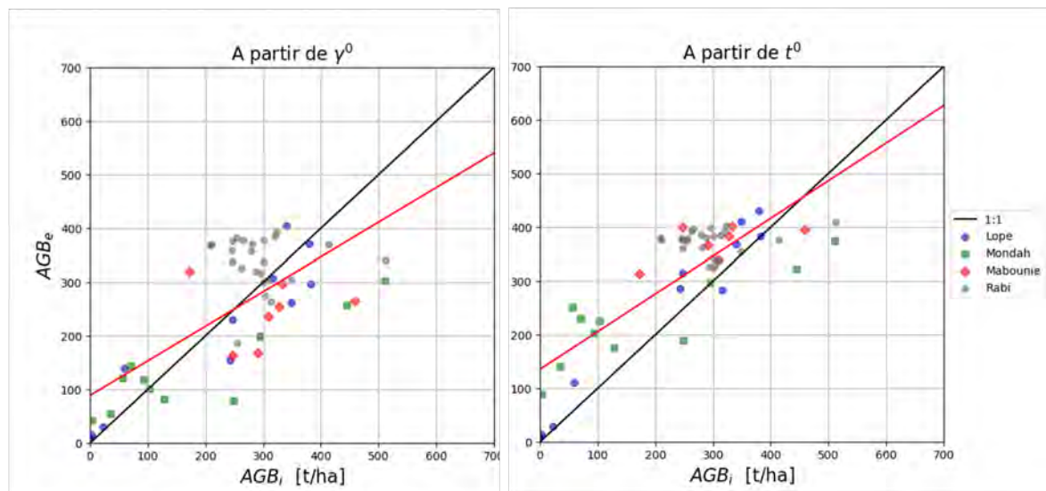
FIGURE 4.43 – Graphes de comparaison entre les biomasses estimées, AGB_e , et les mesures terrain, AGB_i dans le cas d’une inversion bayésienne des cartes d’indicateurs polarimétriques \gamma^0 (à gauche) et t^0 (à droite) à partir des modèles de régression détaillés dans le tableau 4.12 pour les données de la campagne AfriSAR DLR. Les résultats statistiques associés sont regroupés dans le tableau 4.14.
