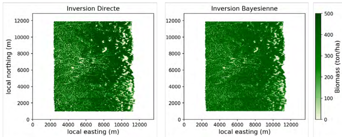
FIGURE 4.55 – Cartes de biomasse à 25 m de résolution, estimées pour le site de la Mabounie à partir de la carte de t^0 calculée pour les données acquises pendant la campagne AfriSAR ONERA. Les paramètres du modèle d'inversion sont dans le tableau 4.15. La carte de gauche a été obtenue après une inversion directe, celle de droite après une inversion bayésienne.
