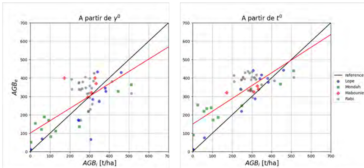
FIGURE 4.62 – Graphes de comparaison entre les biomasses estimées, AGB_e , et les mesures terrain, AGB_i dans le cas d’une inversion bayésienne des cartes d’indicateurs polarimétriques \gamma^0 (à gauche) et t^0 (à droite) à partir des modèles de régression détaillés dans le tableau 4.15 pour les données de la campagne AfriSAR ONERA. Les résultats statistiques associés sont regroupés dans le tableau 4.17.
