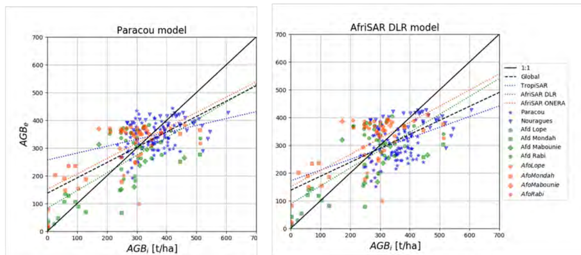
FIGURE 4.67 – Graphes de comparaison entre les biomasses estimées, AGB_e , et les mesures terrain, AGB_i dans le cas d'une inversion bayésienne des cartes d'indicateurs polarimétriques \gamma^0 à partir des modèles de régression de TropiSAR (à gauche) et du DLR (à droite) détaillés dans le tableau 4.18 pour l'intégralité des données disponibles. Les résultats statistiques associés sont regroupés dans les tableaux 4.24 et 4.25.
