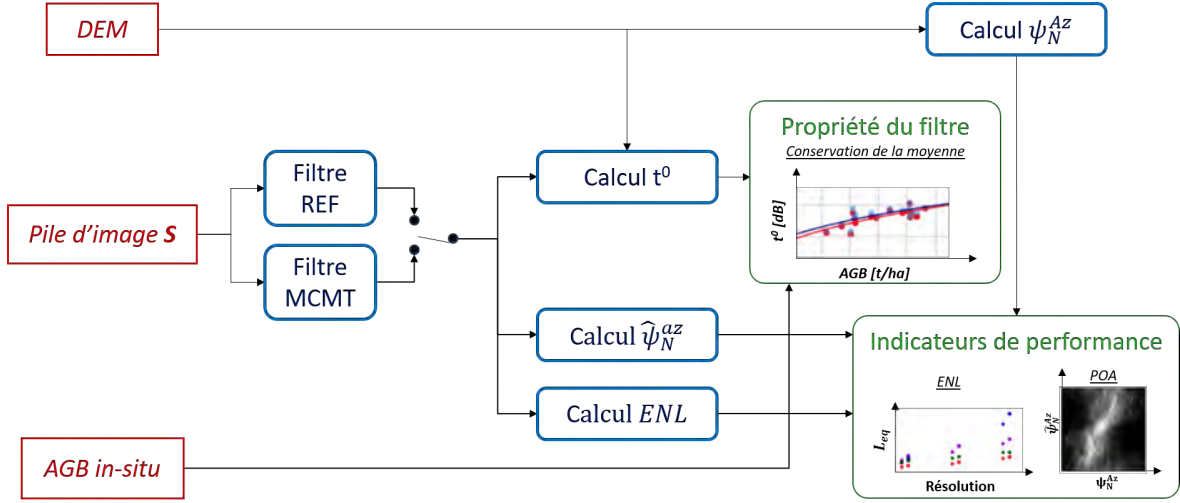
FIGURE 3.4 – Organigramme représentant le processus global d'estimation des performances des filtres REF et MCMT appliqués à une série chronologique PolSAR en bande P.
