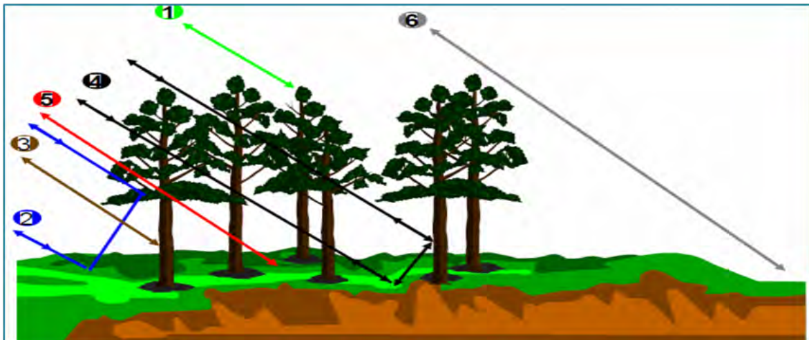
FIGURE 1.2 – Interactions entre le faisceau incident radar et la canopée. (1) Diffusion de la couronne, (2) Diffusion des troncs, (3) Interaction Tronc - sol, (4) Atténuation de la diffusion du sol, (5) Diffusion directe du sol, (6) Interaction troncs - branches. Extrait de [12].
