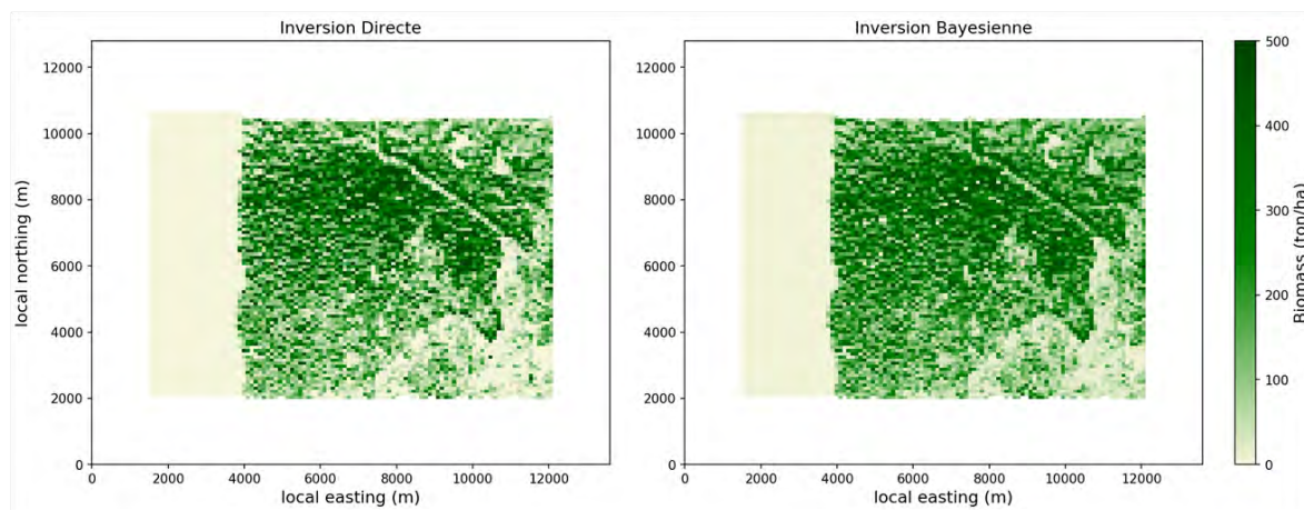
FIGURE 4.52 – Cartes de biomasse à 100 m de résolution, estimées pour le site de Mondah à partir de la carte de t^0 calculée pour les données acquises pendant la campagne AfriSAR ONERA. Les paramètres du modèle d'inversion sont dans le tableau 4.15. La carte de gauche a été obtenue après une inversion directe, celle de droite après une inversion bayésienne.
