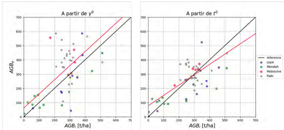
FIGURE 4.61 – Graphes de comparaison entre les biomasses estimées, AGB_e , et les mesures terrain, AGB_i dans le cas d’une inversion directe des cartes d’indicateurs polarimétriques \gamma^0 (à gauche) et t^0 (à droite) à partir des modèles de régression détaillés dans le tableau 4.15 pour les données de la campagne AfriSAR ONERA. Les résultats statistiques associés sont regroupés dans le tableau 4.16.
