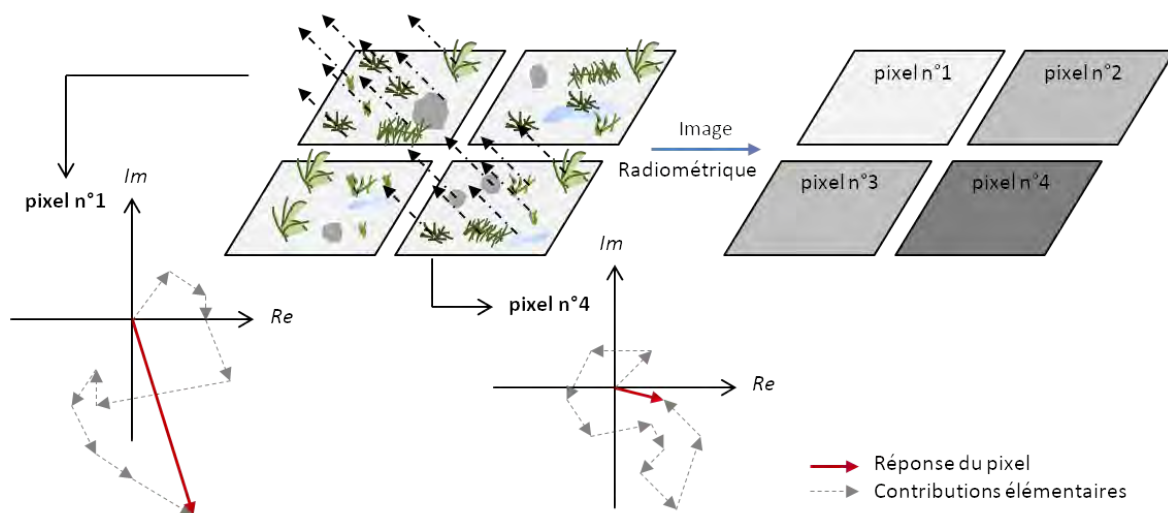
FIGURE 3.1 – (À gauche) origine physique du speckle : effets de la nature cohérente des illuminations radar avec la combinaison des contributions élémentaires dans chaque pixel. (À droite) Distribution radiométrique de l'image SAR résultante. Extrait de [2].
