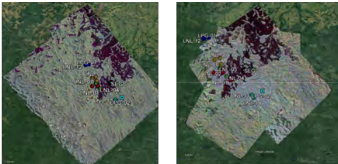
FIGURE 2.6 – Superposition des images bande P acquises sur le site de La Lopé en fausses couleurs (Rouge : HH, Vert : HV, Bleu : VV) avec une localisation des ROI. Axe azimuthal horizontal et axe vertical en range. Extrait de [11].
