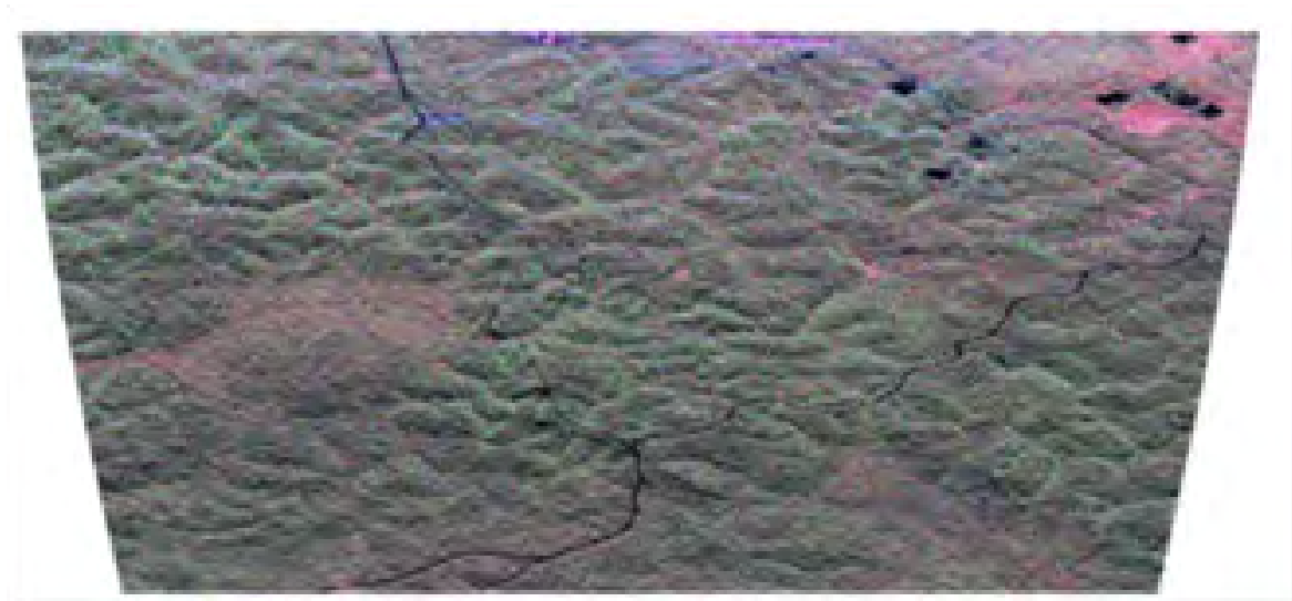
FIGURE 2.9 – Superposition des images bande P acquises sur le site de Rabi en fausses couleurs (Rouge : HH, Vert : HV, Bleu : VV). Axe azimutal horizontal et axe vertical en range. Extrait de [11].
