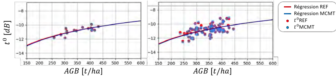
FIGURE 3.5 – Estimation de t^0 en fonction de la biomasse forestière obtenue pour les données PolSAR en bande P du site test de Paracou, acquises avec une bande passante de 125 MHz. La résolution des données après application des filtres REF et MCMT est équivalente à 5 m. Sur la partie gauche de la figure, 15 ROI de 6.25 ha sont considérées ainsi qu'une ROI de 25 ha. Sur la partie droite, 84 ROI de 1 ha sont considérées.
