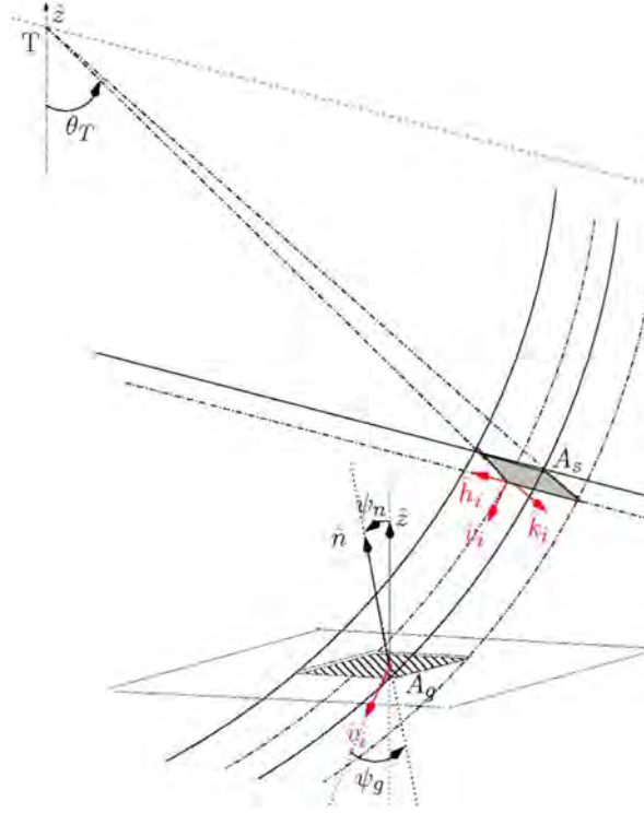
FIGURE 3.8 – Schématisation de la géométrie oblique d'un capteur SAR en fonction de l'angle d'élévation \theta_T , des surfaces inclinées et surfaces au sol A_s et A_g , de la base de transmission ( \hat{k}_i , h_i , v_i ), des vecteurs vertical et normal \hat{z} , \hat{n} , des angles de pente \psi_n et \psi_g ainsi que du volume d'interception lié à la résolution au sol de la cellule d'acquisition. Extrait de [13].
