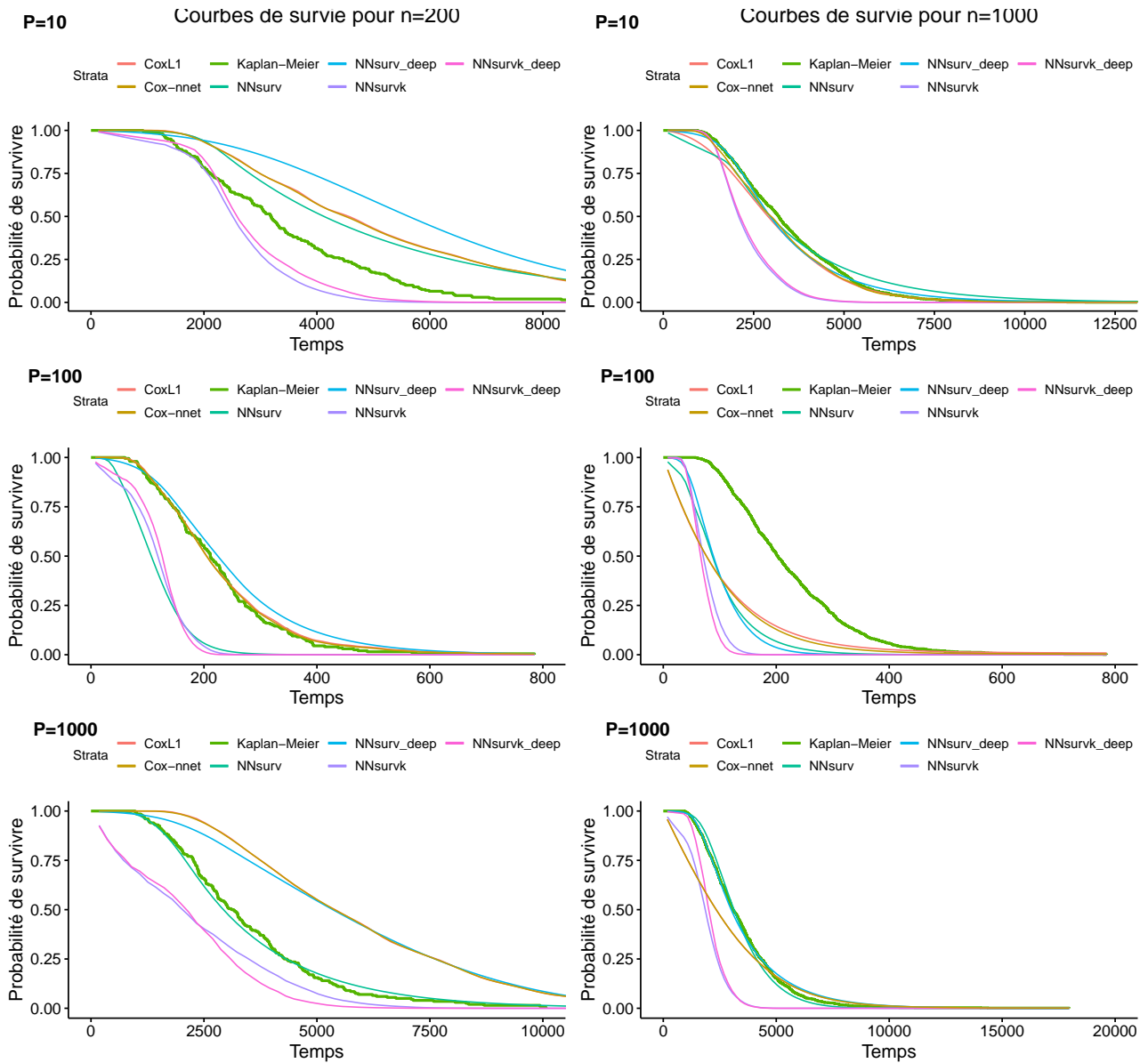
FIGURE 3.16 – Courbes de survie obtenues à partir des méthodes pour la simulation AH/Log-normale
