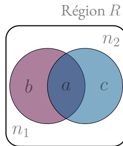
FIGURE B.1 – Schéma de la région R quand 2 sites sont considérés S = 2
