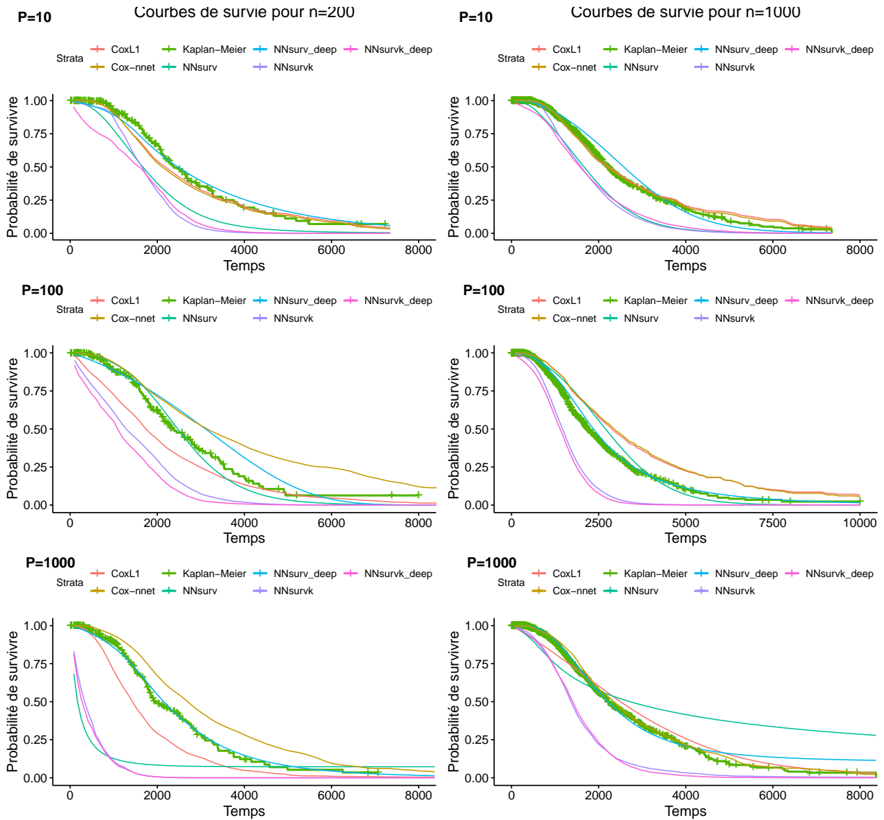
FIGURE 3.18 – Courbes de survie obtenues à partir des méthodes pour la simulation AFT/Log-normale censurée
