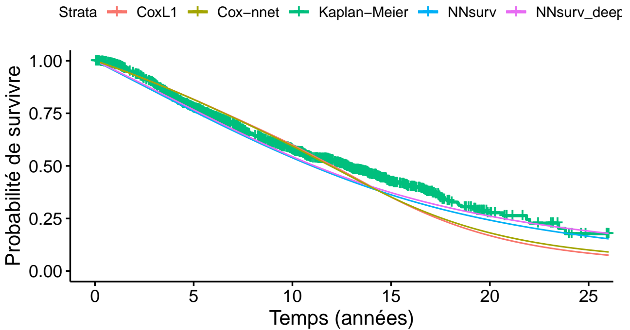
FIGURE 3.22 – Courbes de survie obtenues à partir des méthodes sur le jeu de données du cancer du sein provenant du projet METABRIC
