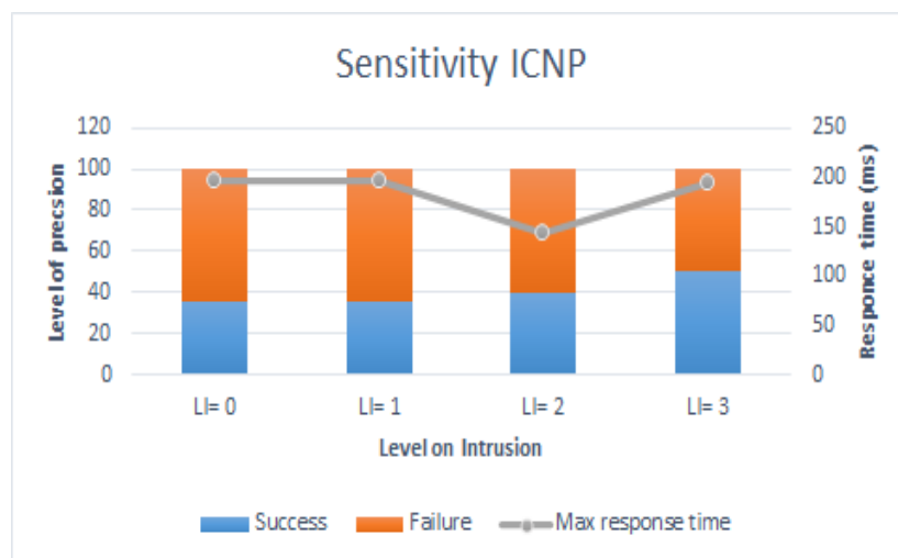
Figure 5.19 – ICNP SA results
