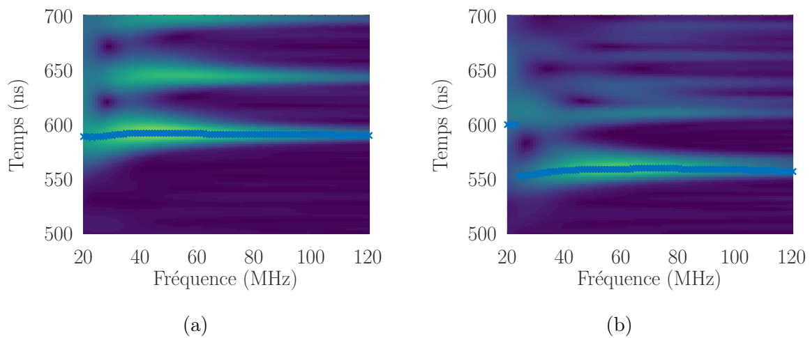
FIGURE 3.8 – Spectres en énergie pour un signal enregistré a) dans l'eau et b) dans un sphéroïde. Les croix bleues indiquent le temps de vol de la composante L du signal acoustique.
