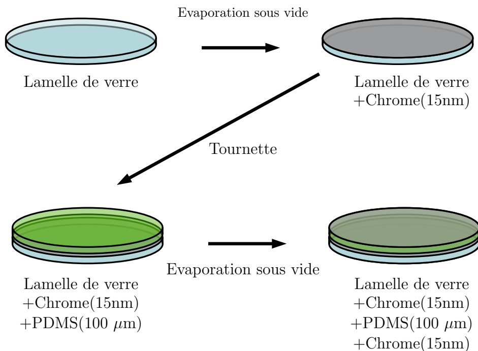
FIGURE 4.8 – Schéma des différentes étapes de fabrication de l'interféromètre de Fabry-Pérot.
