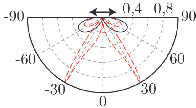
FIGURE 2.2 – Diagramme de directivité des ondes de compression (traits pleins) et de cisaillement (traits pointillés) pour une génération surfacique en régime thermoélastique (adapté du manuscrit de thèse de S. Raetz [91])
