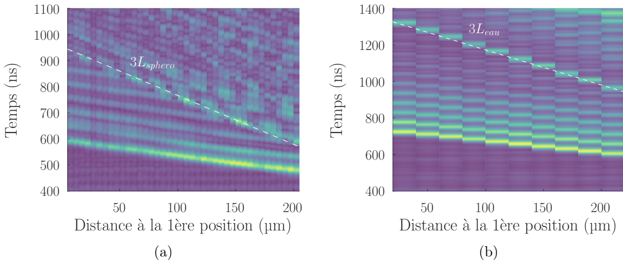
FIGURE 3.21 – Carte des spectres de répartition d'énergie temporelle à 40 MHz pour a) un sphéroïde HCT116 et b) une couche d'eau
