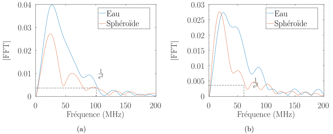
FIGURE 3.5 – a) Spectre de la composante L du signal acoustique enregistré dans l'eau (bleu) et dans le sphéroïde (rouge). b) Spectre de la composante 3L_{verre} du signal acoustique enregistré dans l'eau (bleu) et dans le sphéroïde (rouge).
