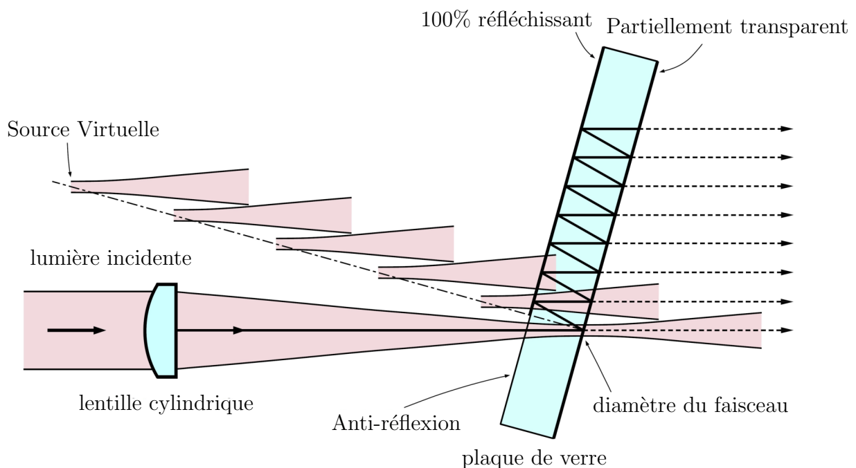
FIGURE 4.2 – Schéma de principe du VIPA. (adapté de Shirasaki [123])
