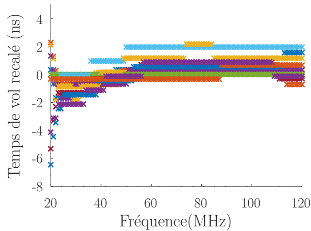
FIGURE 2.19 – Temps de vol recalés en fonction de la fréquence acoustique pour différentes positions.
