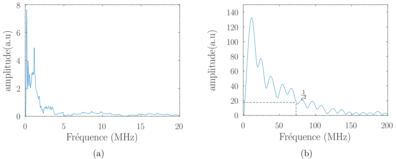
FIGURE 2.13 – a) Spectre du signal complet de 0 à 40 MHz b) Spectre du pic L dans le signal de plaque
