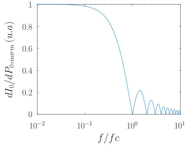
FIGURE 4.7 – Sensibilité acoustique en fonction de la fréquence pour un interféromètre de Fabry-Pérot monté sur un substrat rigide
