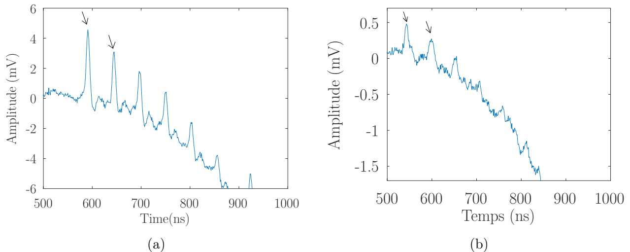
FIGURE 3.4 – Comparaison entre un signal acoustique enregistré à travers a) une couche d'eau et b) à travers un sphéroïde.
