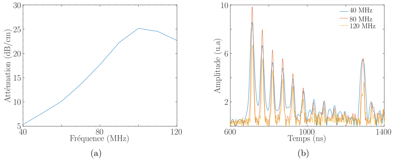
FIGURE 2.26 – a) Courbe d’atténuation mesurée sur une couche d’eau. b) Spectre de répartition temporelle de l’énergie correspondant à un signal enregistré dans une couche d’eau à 3 fréquences différentes.
