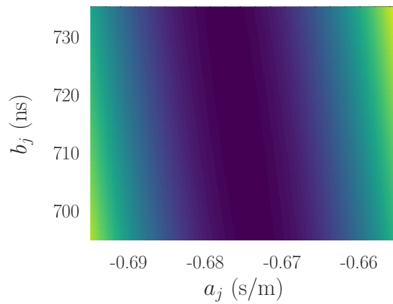
FIGURE 2.23 – Exemple de carte de l'erreur quadratique en fonction des paramètres de l'ajustement
