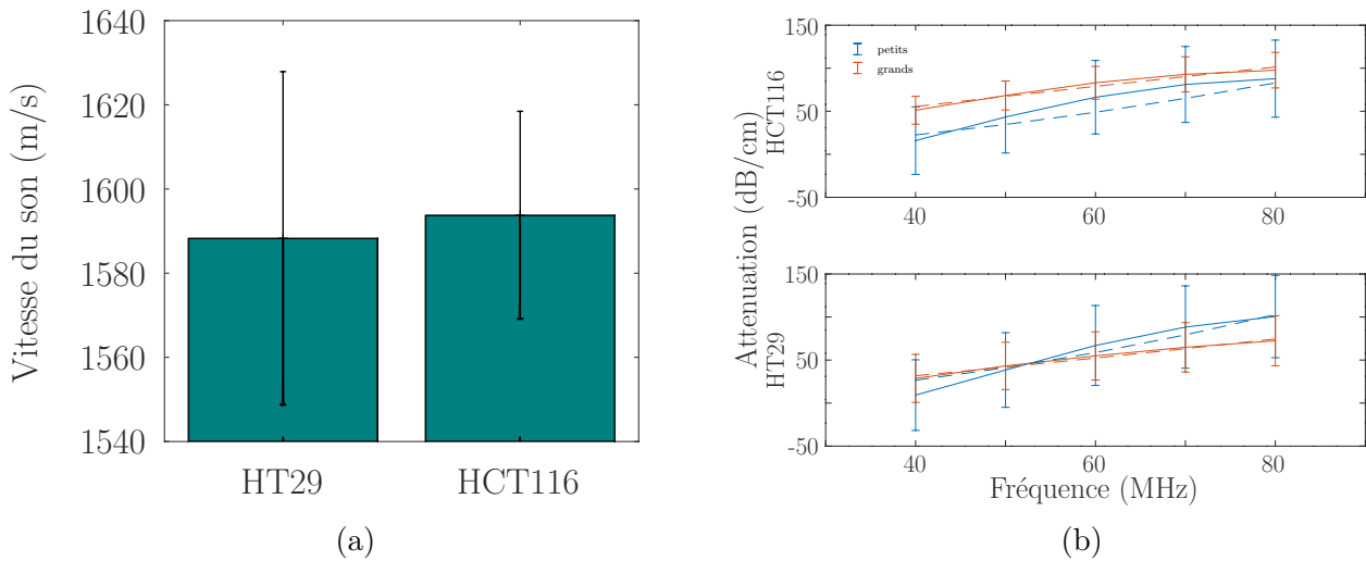
FIGURE 4.1 – Résultats de (a) vitesse du son et (b) d'atténuation acoustique sur les sphéroïdes des lignées HCT116 et HT29
