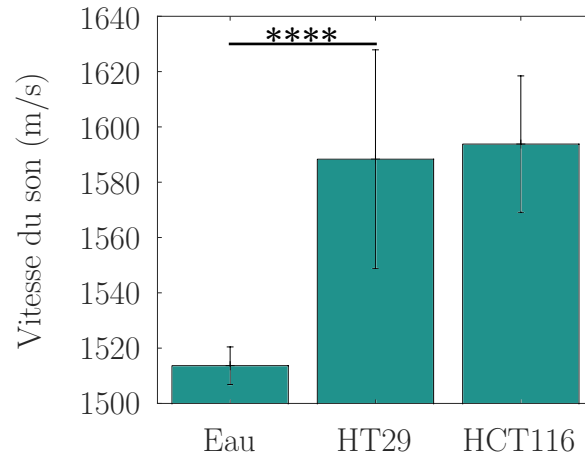
FIGURE 3.14 – Moyenne et écart des vitesses du son mesurées dans l'eau à 35°C et les sphéroïdes HCT116 et HT29. Le couple eau-HT29 donne une p-valeur de p = 0.0001 . Le couple eau-HCT116 donne une p-valeur de p = 0.005
