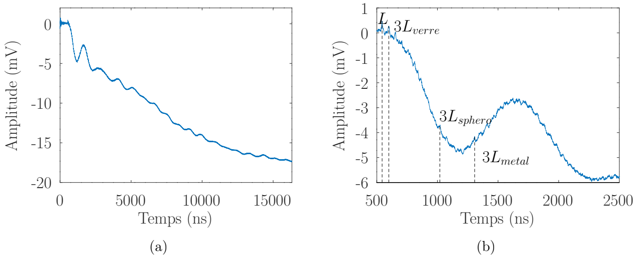
FIGURE 3.3 – Signal acoustique enregistré dans un sphéroïde : a) Signal complet et b) Zoom sur les 2.5 premières microsecondes.
