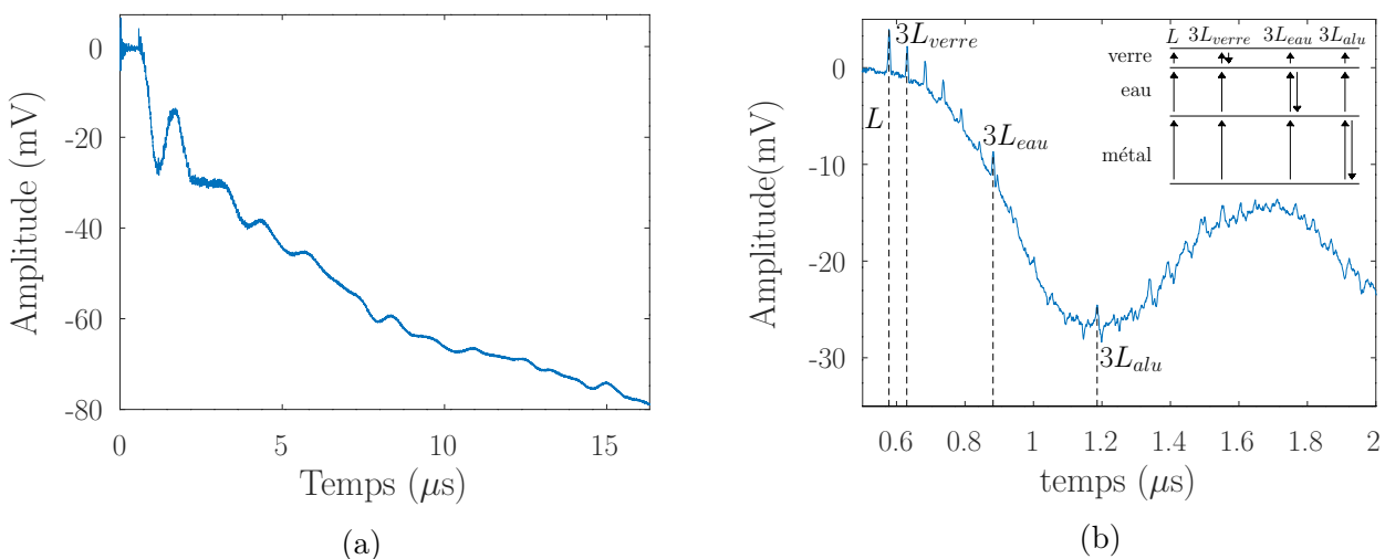
FIGURE 2.16 – (a) Signal acoustique complet enregistré à travers une couche d'eau. (b) Zoom sur les deux premières microsecondes du signal où on a mis en évidence l'ensemble des composantes longitudinales
