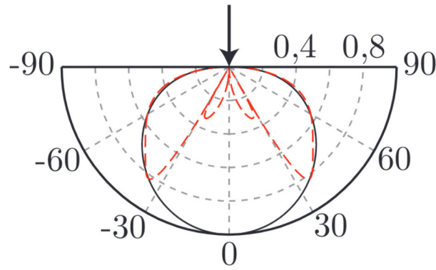
FIGURE 2.5 – Diagramme de directivité des ondes de compression (traits pleins) et de cisaillement (traits pointillés) pour une génération surfacique en régime d'ablation (adapté du manuscrit de thèse de S. Raetz [91])
