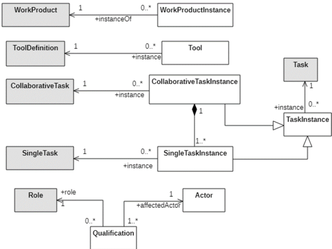
FIGURE 3.9: Relations d'instanciation entre éléments des deux paquets de ECPML.
