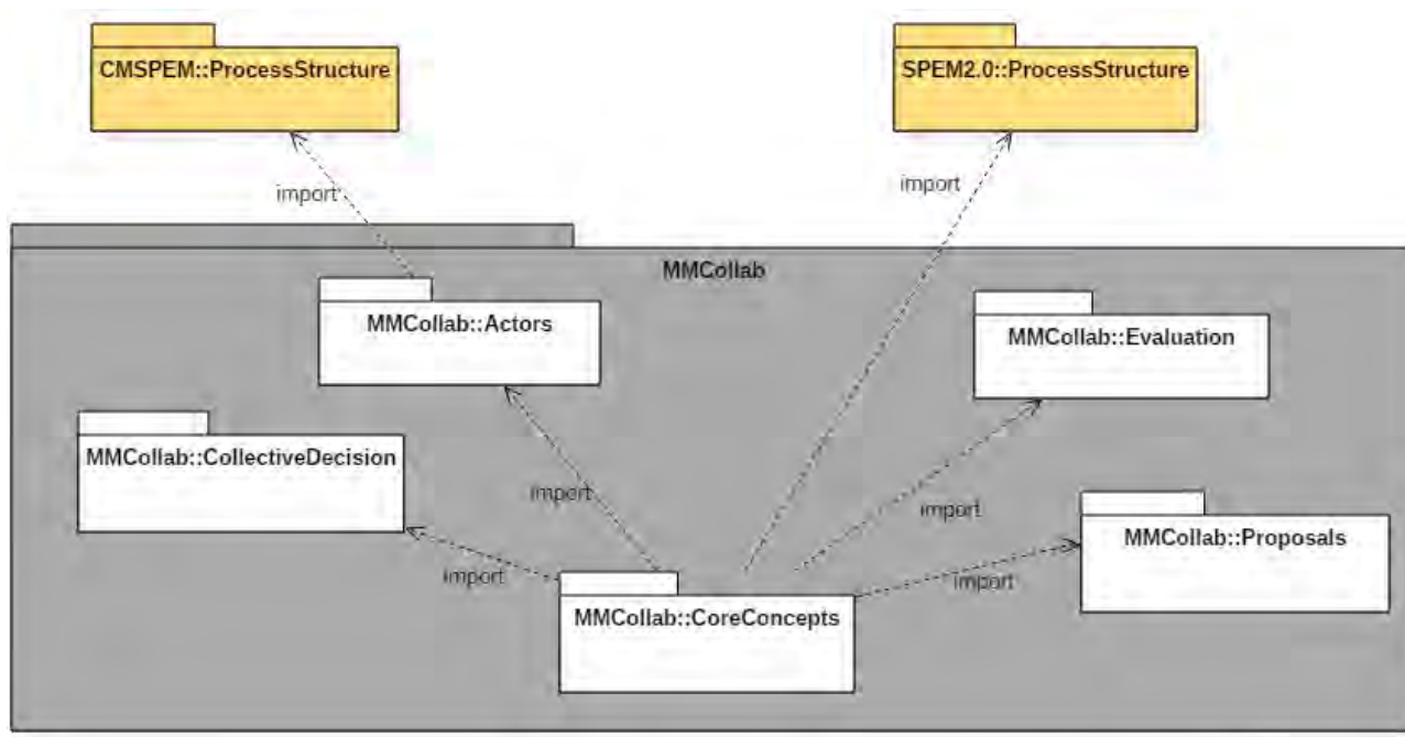
FIGURE 2.19: Organisation en paquetages du méta-modèle MMCollab (Bennani et al., 2019).
