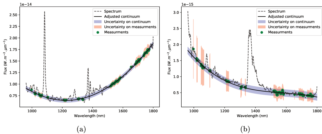
FIGURE 2.16 – Extraction du continuum d’émission : le spectre mesuré est en pointillés, les points de mesure du continuum sont représentés par des points verts avec une incertitude rose, enfin le continuum ajusté par un polynôme est représenté en trait continu noir avec une incertitude marquée en bleu. Les deux spectres correspondent à des fenêtres de 0,3'' de largeur, pour la figure de gauche (a) autour du maximum d’émission, pour la figure de droite (b) autour de 3'' Nord.
