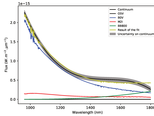
FIGURE 2.26 – Ajustement du continuum d’émission mesuré en bord de fente avec des spectres stellaires théoriques d’étoiles O5V, B0V et M2I.
