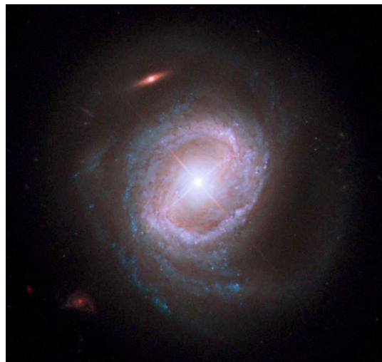
FIGURE 1.1 – Mrk 817, une galaxie spirale qui héberge en son centre un noyau actif. Les quatre aigrettes de diffraction visibles autour de la source centrale soulignent que celle-ci est non résolue ( \leq 0,1'' ). Superposition d'images prises avec les filtres B, V, I et H- \alpha de l'instrument WFC3 du Hubble Space Telescope (Crédit : ESA/Hubble).
