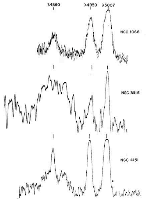
FIGURE 1.3 – Spectres de trois noyaux de galaxie autour de 500 nm tels que présentés dans Seyfert (1943). La raie la plus à gauche est la raie permise de l'hydrogène H_{\beta} à \lambda = 4860 \text{ nm} , tandis que les deux raies les plus à droites sont un doublet de transitions interdites [OIII] à \lambda = 4959 \text{ nm} et \lambda = 5007 \text{ nm} . De haut en bas les spectres correspondent à NGC 1068, NGC 3516 et NGC 4151. Les raies interdites possèdent un profil étroit dans les trois galaxies, tandis que la raie de H_{\beta} est étroite pour NGC 1068, large pour NGC 3516, et semble être la superposition d'une raie étroite sur une raie large pour NGC 4151.
