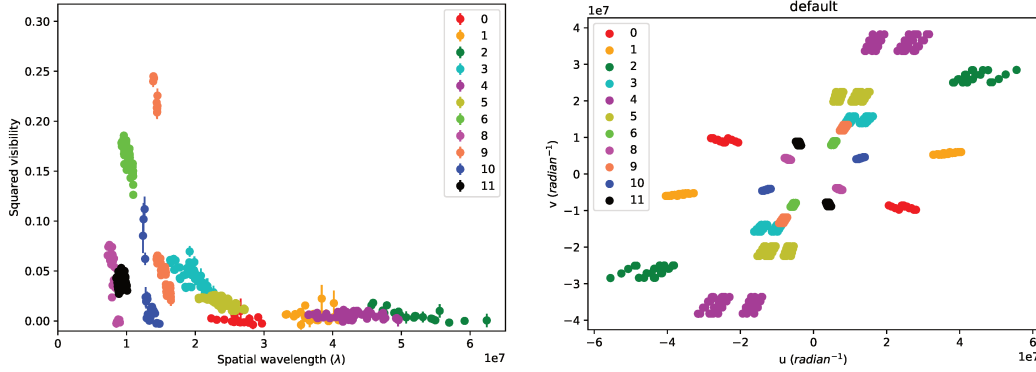
FIGURE 3.13 – Points de visibilité carrée et plan u-v en incluant les données issues des AT.
