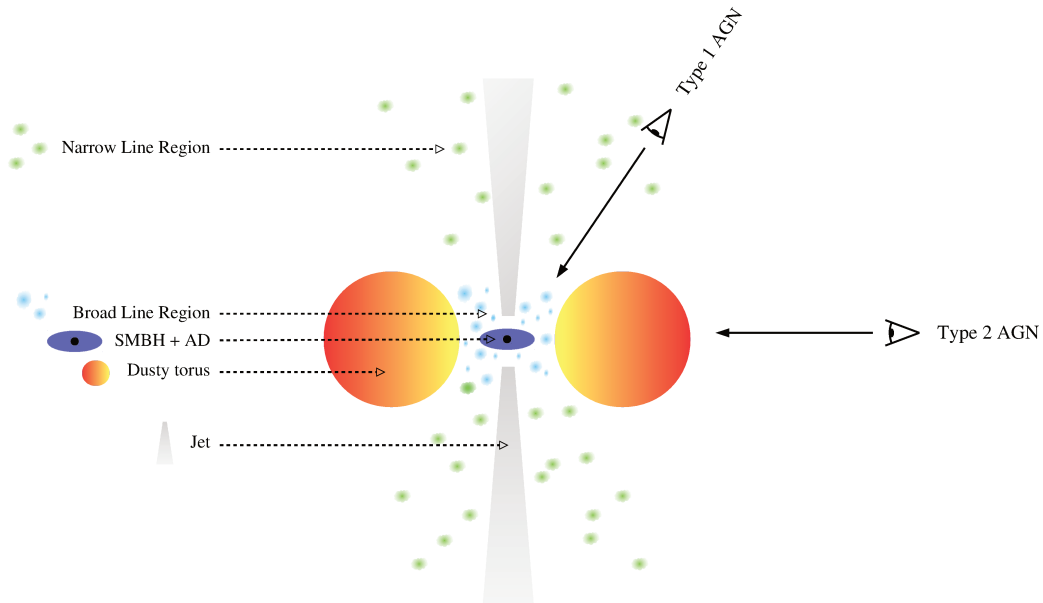
FIGURE 1.4 – Schéma classique du modèle unifié des noyaux actifs de galaxie. Les différents composants sont représentés de manière schématique au centre : le trou noir, le disque d'accrétion ainsi qu'une couronne, qui seraient respectivement les
