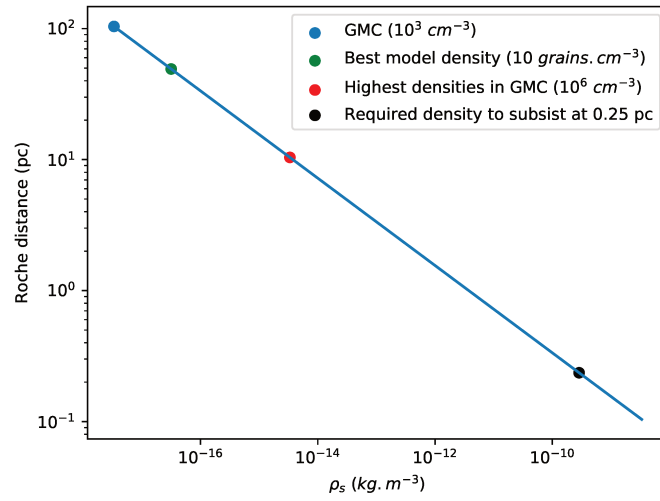
FIGURE A.2 – Distance de Roche autour de la masse centrale de NGC 1068 en fonction de la densité du satellite. Les densités représentatives du milieu interstellaire dense sont données à titre d'exemple, tout comme la densité du meilleur modèle MontAGN.
