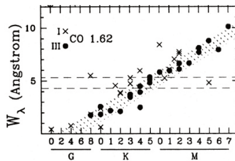
FIGURE 2.36 – Variation de la largeur équivalente de CO(6,3) 1,62\mu m en fonction du type spectral de l'étoile. Les cercles indiquent les géantes, et les croix les supergéantes. Crédit : Figure extraite de la figure 5a de Origlia et al. (1993)
