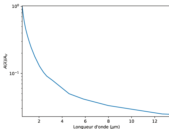
FIGURE A.1 – Courbe d’extinction utilisée en avant plan du modèle GRAVITY, exprimée en fonction de la longueur d’onde et normalisée à sa valeur dans la bande V.
