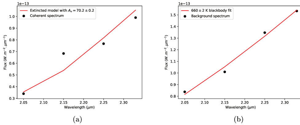
FIGURE 3.31 – Ajustements spectraux du modèle 2. (a) : ajustement d’une extinction sur le spectre cohérent observé de la source. (b) : Spectre du fond diffus calculé, et ajustement d’une émission de corps noir.
