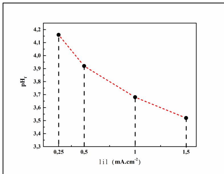
Figure III.12. Evolution du \text{pH}_{\text{final}} de l'électrolyte après l'électrodéposition de la couche à base d'oxyde de cérium en fonction des différentes densités de courant appliquées.
