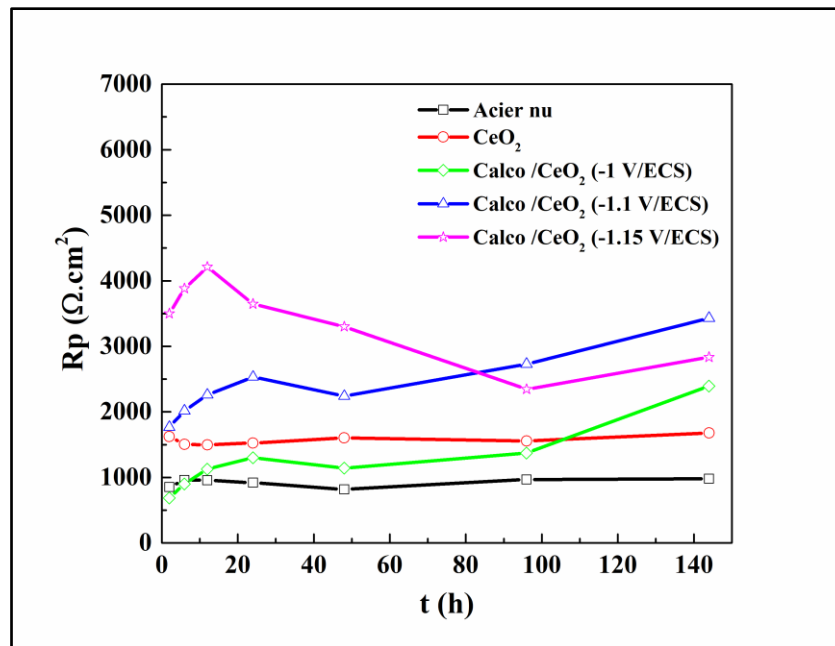
Figure IV.22. Variation en fonction du temps d'immersion dans l'eau de mer artificielle de la résistance de polarisation ( R_p ) de l'acier nu, du revêtement CeO 2 et des dépôts calcaires/CeO 2 formés à différents potentiels dans l'eau de mer artificielle exempte de Mg.
