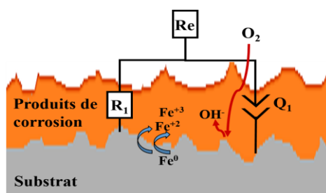
Figure V.26. Schéma montrant le circuit électrique équivalent utilisé pour analyser les données d'impédance du système acier nu/eau de mer.
