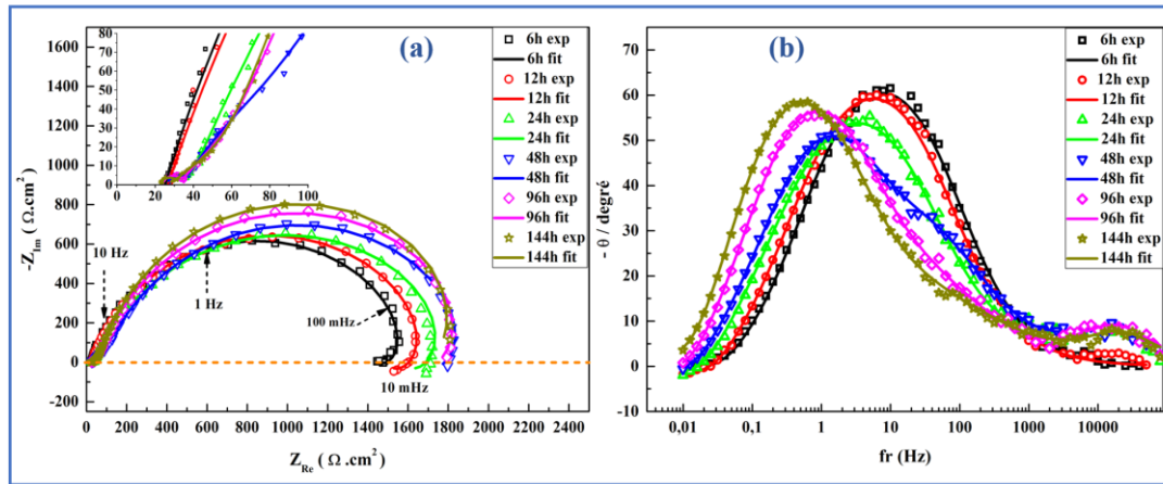
Figure V.29. Diagrammes d'impédance électrochimique expérimentaux et ajustés du système dépôt CeO 2 /eau de mer, après différents temps d'immersion, en présentation de Nyquist (a) et Bode (b).
