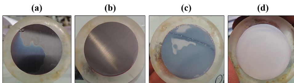
Figure III.5. Macrographies des électrodes d'acier après polarisation à 20mV/s, dans la solution aqueuse de \text{Ce}(\text{NO}_3)_3, 6\text{H}_2\text{O} à différentes concentrations : (a) 0.01M ; (b) 0.05M ; (c) 0.1M et (d) 0.2M.
