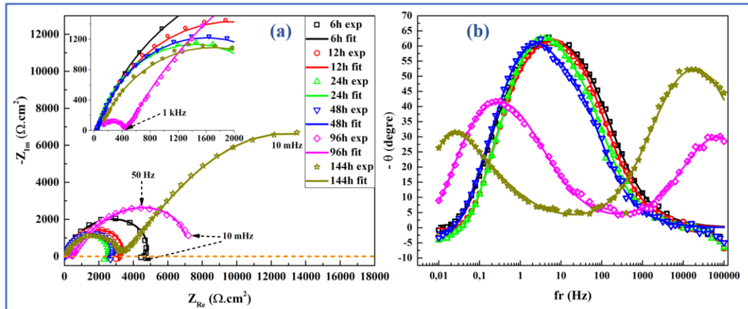
Figure V.30. Diagrammes d'impédance électrochimique expérimentaux et ajustés du système (Mg(OH) 2 /CeO 2 )/eau de mer, après différents temps d'immersion, en présentation de Nyquist (a) et Bode (b).
