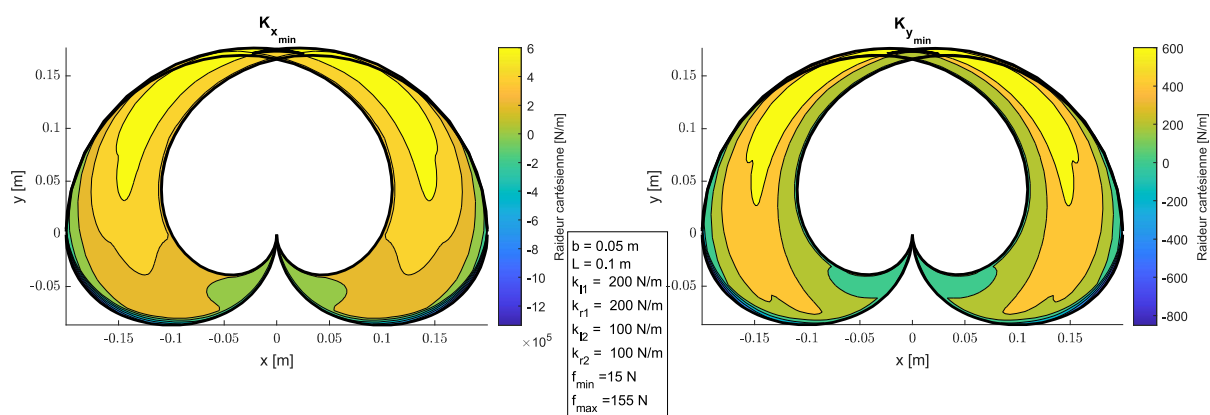
FIGURE 4.22 – Espace de travail accessible et raideur cartésienne minimale pour la stratégie strut-routed.
